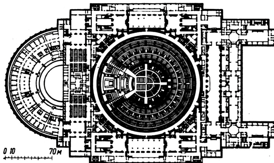
Figure 65 – Plan du Palais des Soviets, architecte Boris Iofan. (Source : Soviet-Magazine d'Architecture Soviétique , Publications PD, 1946 ; archives du Musée National d'Architecture Shchusev, Moscou).
