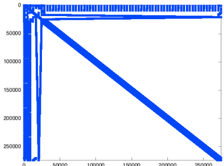
Cube 6 T-Omega: n=274625 , nnz=4018753
