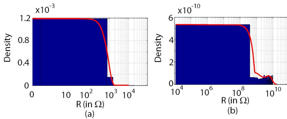
Figure 8.12: L'estimation de la fonction de densité de probabilité p(R|F_i) pour deux types de défaut (a) court-circuit (b) circuit-ouvert
