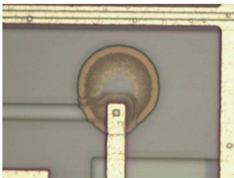
Figure 8.4: Un circuit-ouvert dans le contact causé par un résidu [3].
