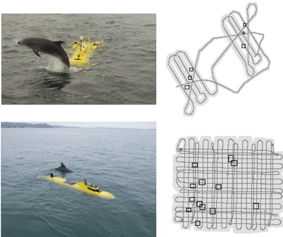
Figure 4.1 – En haut, le Redermor et sa trajectoire effectuée (vue du dessous), avec la position des amers (carrés noirs). En bas, la Daurade lors d’une expérience dans la baie de Douarnenez (photos DGA/GESMA).
