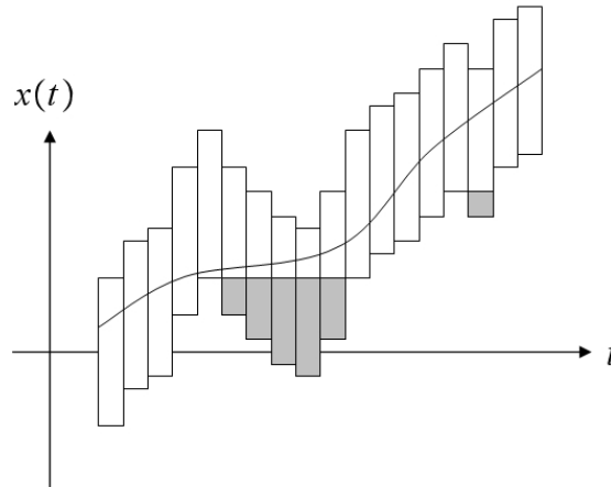
Figure 3.5 – Une contrainte de croissance sur x(t) permet d'éliminer les parties grises du tube initial.
