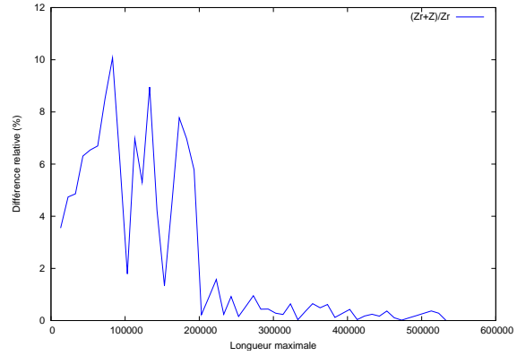
FIG. 2.16 – Comparaison entre M_1 et sa relaxation pour a10e
