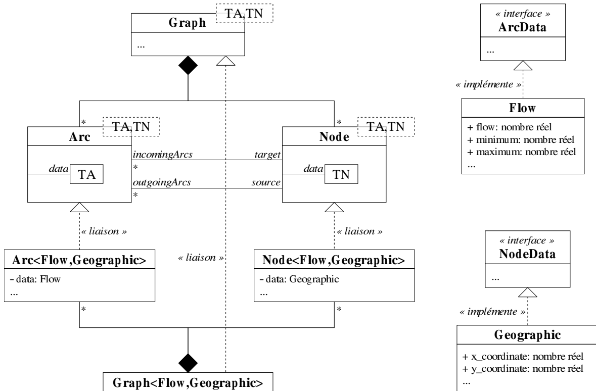
FIG. D.2 – Graphe modélisé par généricité.
