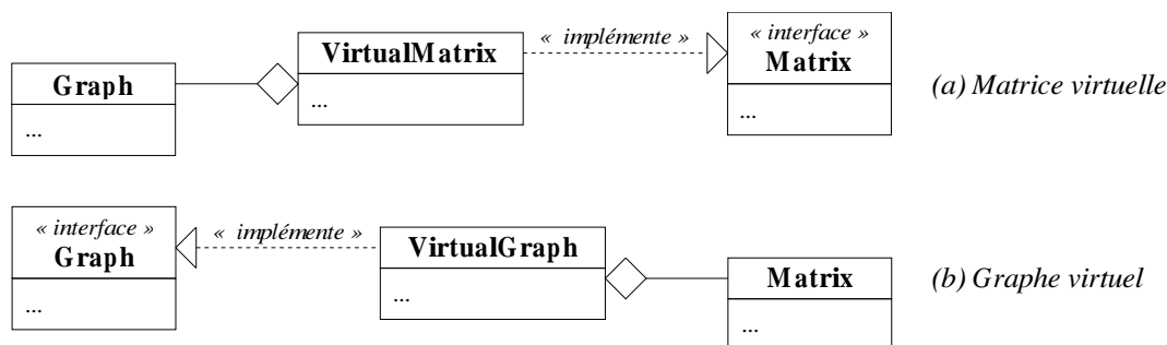
FIG. D.13 – Structure de données virtuelle.
