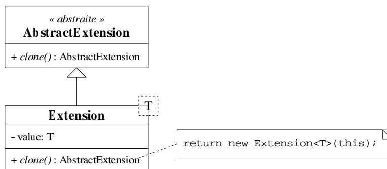
FIG. D.9 – Classe Extension .
