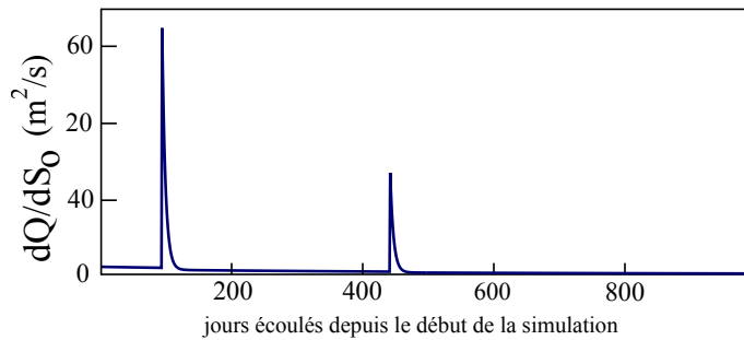
FIGURE 8 – Étude analytique de la sensibilité du débit simulé en sortie d’un modèle global à réservoir au niveau initial de remplissage du modèle. Exemple de la sensibilité du débit au niveau initial de remplissage du réservoir inférieur du modèle Vensim proposé par FLEURY, 2005. Les pics de sensibilité observés 100 et 450 jours après le début de la simulation sont déclenchés par l’activation d’une fonction de transfert à seuil gouvernée par le niveau de remplissage d’un réservoir à dynamique lente. Une erreur de 10cm sur l’estimation du remplissage initial engendre une erreur sur le débit simulé supérieure à 6\text{m}^3/\text{s} 100 jours après le début de la simulation et de 4\text{m}^3/\text{s} environ 450 jours après le début de la simulation. Ces chiffres sont à rapporter au débit de pointe de l’exsurgence considérée ( 18\text{m}^3/\text{s} ). Voir chapitre 2.
