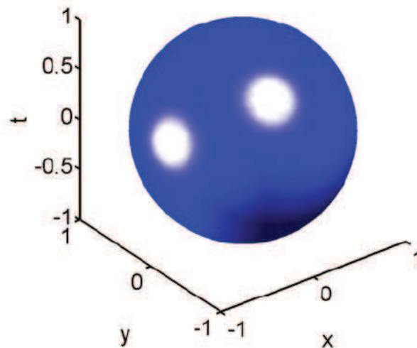
FIG. 1.5 Exemple de soliton spatio-temporel «balle de lumière».
