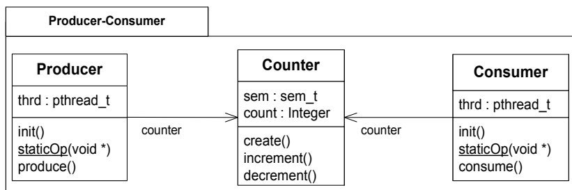
FIGURE 4.8 – Modèle de l’application Producteur/Consommateur spécifique à C++/POSIX
