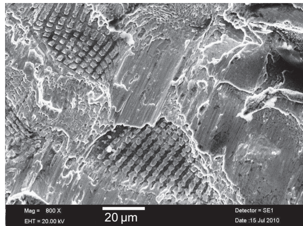
Fig 14. Image MEB qui montre l'état des micro-grilles après déformation à 1050°C et 10s-1, les micro-grilles s'avèrent inexploitables pour déterminer des champs de déformation.
