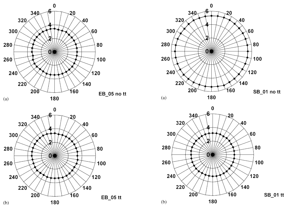
Figure 2.6 : Effet du traitement thermique sur les vitesses des ondes élastiques dans EB (gauche) et SB (droite). Les graphes du haut et du bas correspondent respectivement à avant et après la chauffe à 900°C. Les vitesses en km.s -1 sont mesurées radialement tous les 10°. Extrait de [Vinciguerra et al., 2005].
