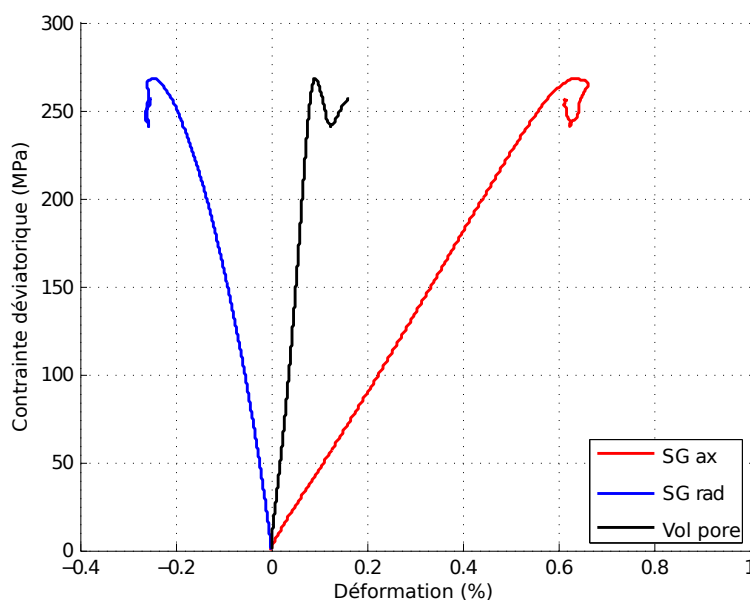
Figure 2.29 : Données de déformation acquises lors de l'augmentation de contrainte axiale au cours de l'essai VII.
