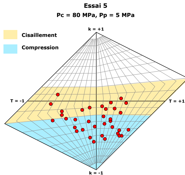
Figure 2.27 : Mécanismes au foyer des 35 événements de plus forte magnitude ( M_w > -2.6 ) enregistrés au cours de l'essai 5. Représentation dans le diagramme T, k d'Hudson.
