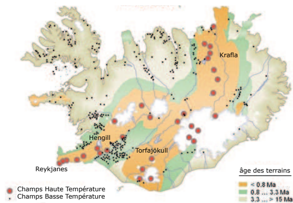
Figure 1.2 : Champs géothermiques islandais, modifié d'après Pálsson and Jonnasson [2006]. Les champs HT sont localisés au droit des chambres magmatiques ou des principaux systèmes intrusifs en refroidissement.
