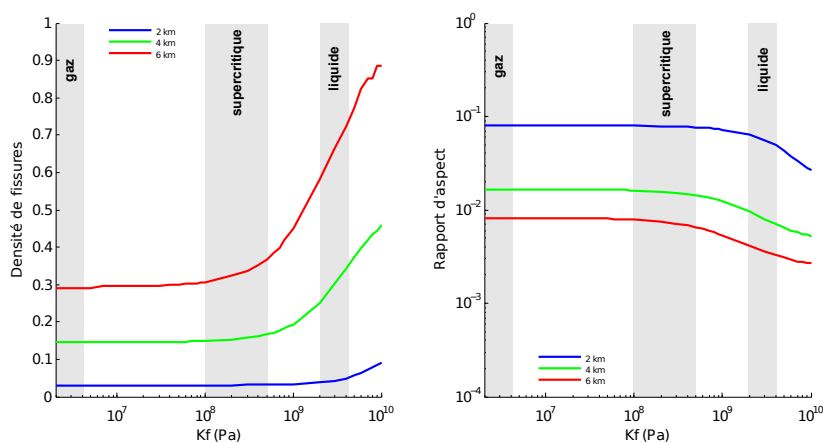
Figure 1.32 : Sensibilité des paramètres de fissuration à la compressibilité du fluide au niveau de l'anomalie de Kleifarvatn. Les porosités de fissures et totale ont été respectivement fixées à 1 et 2 %. Les courbes colorées correspondent aux 3 profondeurs d'investigation.
