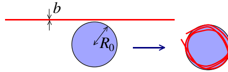
FIGURE 4.8 – Enroulage d'un filament autour d'une goutte.
