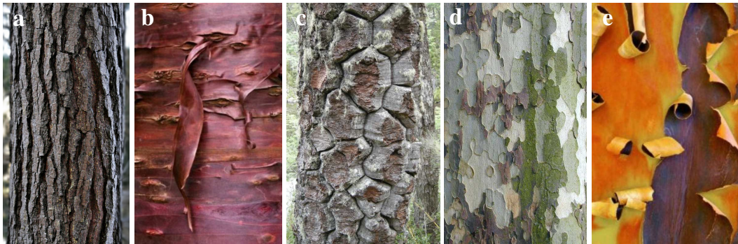
FIGURE 7.28 – Différentes textures d'écorces : (a) pin, (b) arctostaphylos, (c) araucaria, (d) platane, (e) érable (image tirée de « Écorces », très joli livre de C. Pollet, éd. Elmer).
