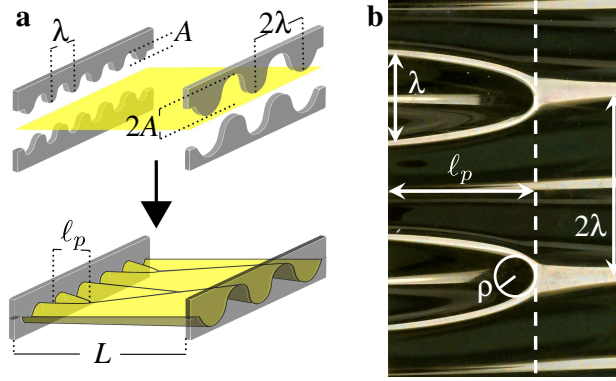
FIGURE 7.19 – (a) Expérience modèle permettant d’isoler le doublement de longueur d’onde des plis. En amont une longueur d’onde \lambda et une amplitude A sont imposées, alors qu’en aval les plis ont une longueur d’onde 2\lambda et une amplitude 2A (qui permet de préserver la largeur de la feuille). (b) Plis vus du dessus, le doublement de longueur d’onde s’effectue à une distance \ell_p des bords.
