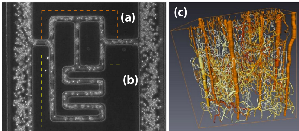
Figure 2.2: Globules rouges dans un réseau capillaire microfluidique modèle (a) Grande concentration de globules (b) concentration plus faible de globules rouges (c) Ecoulement sanguin dans un réseau capillaire (structure mesurée par tomographie) calculé par un modèle simplifié. Les couleurs montrent la concentration locale des globules rouges : les couleurs foncées correspondent à une concentration plus élevée des globules rouges alors que les couleurs plus claires montrent les concentrations plus faibles que la moyenne [3]
