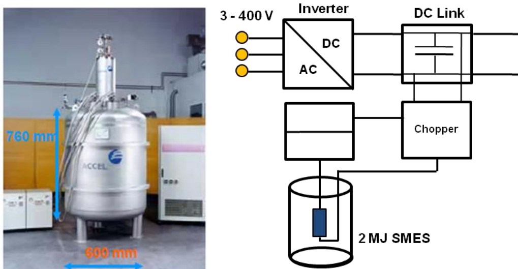
Figure 1.6. – Dispositif de stockage d'électricité par une inductance supraconductrice [Multon et al. 2008].
