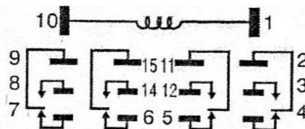
Figure 3.3- Relais Panasonic HG 4formc. La bobine excitatrice est alimentée par les contacts (1,10). Les entrées sont repérées par les contacts (9,15,11,2). Les sorties par les contacts (8,14,12,3) ou (7,6,5,4). Les contacts supportent jusqu'à 20 A sous 250 Volts AC. Le temps de réponse est 20 ms.
