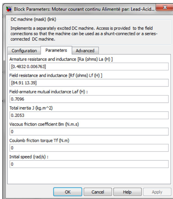
Figure 4.10 - Caractéristiques du moteur courant continu à excitation indépendante considérées sous Matlab/Simulink.
