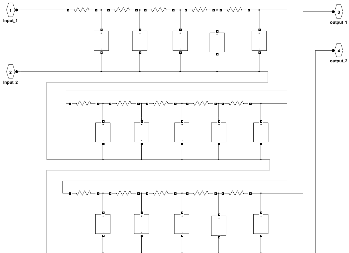
Figure 2.24 – Contenu du bloc modélisant la ligne de transmission.
