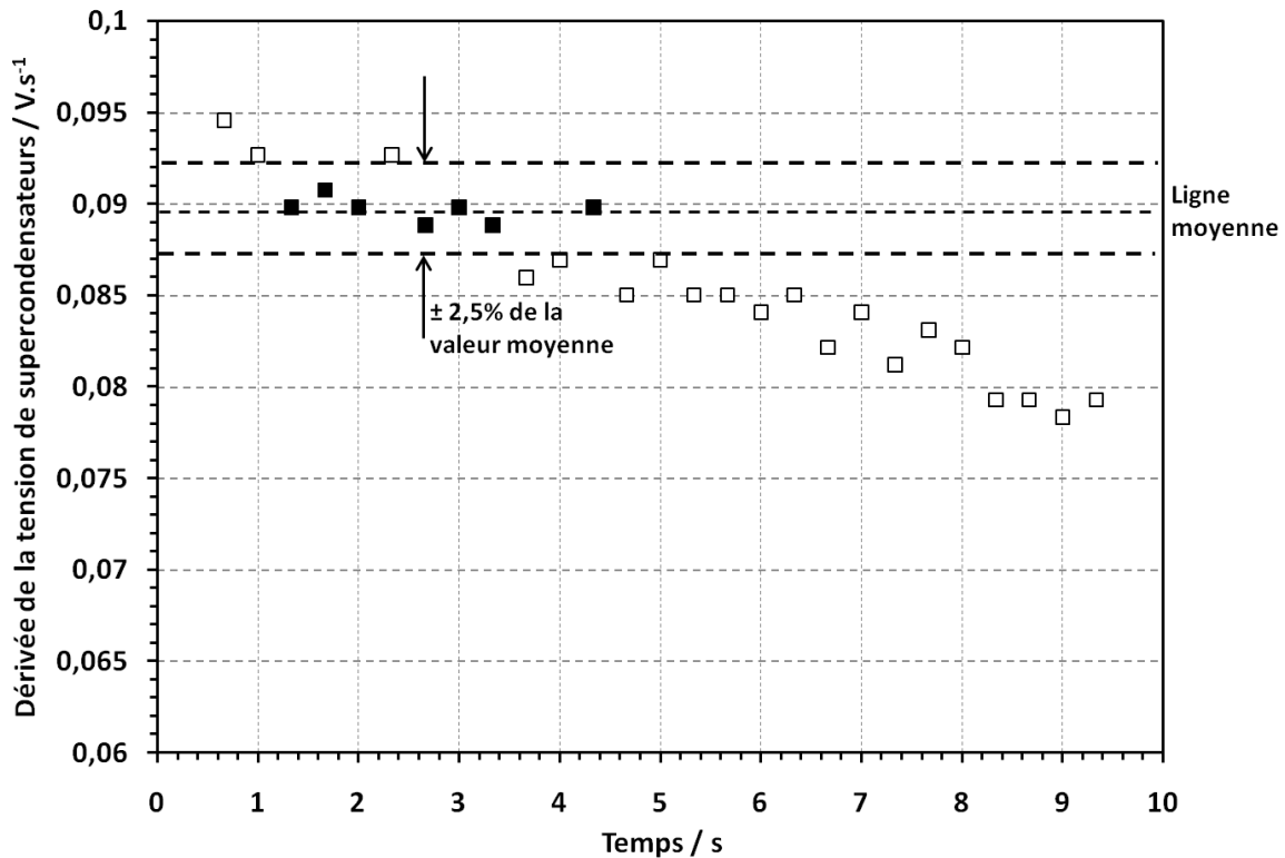
Figure 3.12 – Dérivée instantanée (marqueurs carrés fond blanc) et dérivée filtrée (marqueur carrés fond noir). Un filtre à \pm 2,5\% de la valeur moyenne est appliqué.
