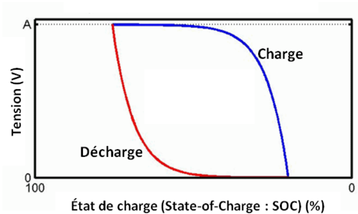
Figure 2.28 – Caractéristique tension versus état de charge (SOC)
