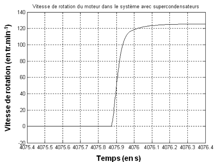
Figure 4.14 – Évolution de la vitesse de rotation du moteur à courant continu.
