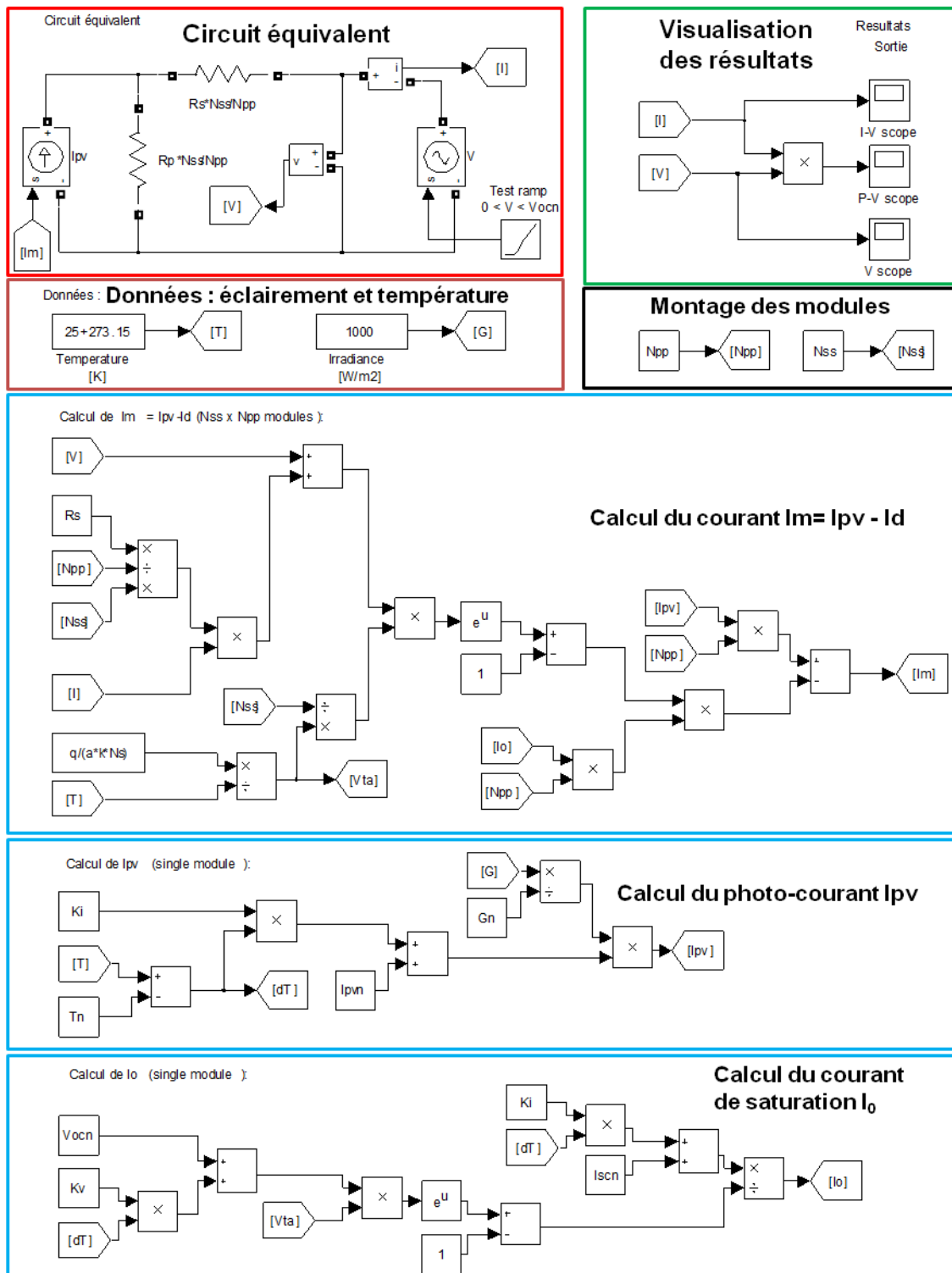
Figure 2.12 - Synoptique du modèle amélioré de la cellule photovoltaïque sous le logiciel Simulink [Villalva et al 2009].
