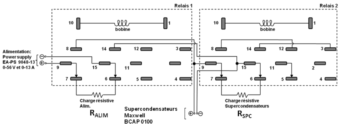
Figure 3.5. – Schéma de câblage des relais 1 et 2 pour réaliser un cycle de charge à partir d'une tension initiale.
