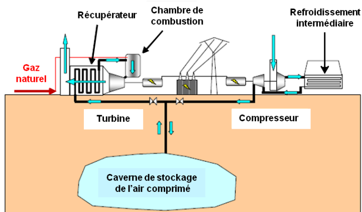
Figure 1.3 – Stockage mécanique par air comprimé [Multon et Ruer].
