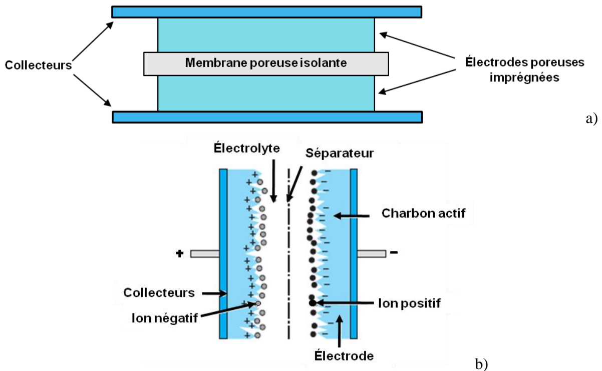
Figure 1.14 – a) Constitution d'un supercondensateur b) Schéma d'un supercondensateur.
