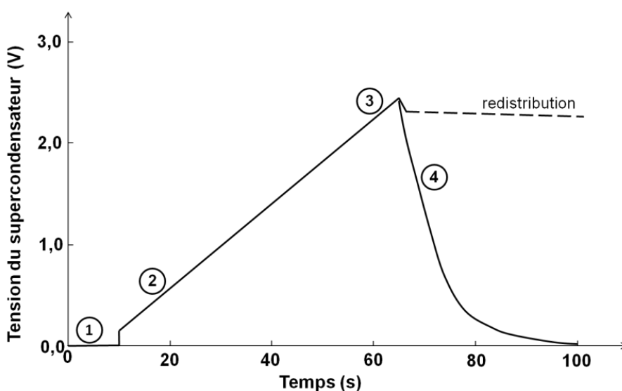
Figure 1.15 – Principe de la charge/décharge d'un supercondensateur électrostatique.
