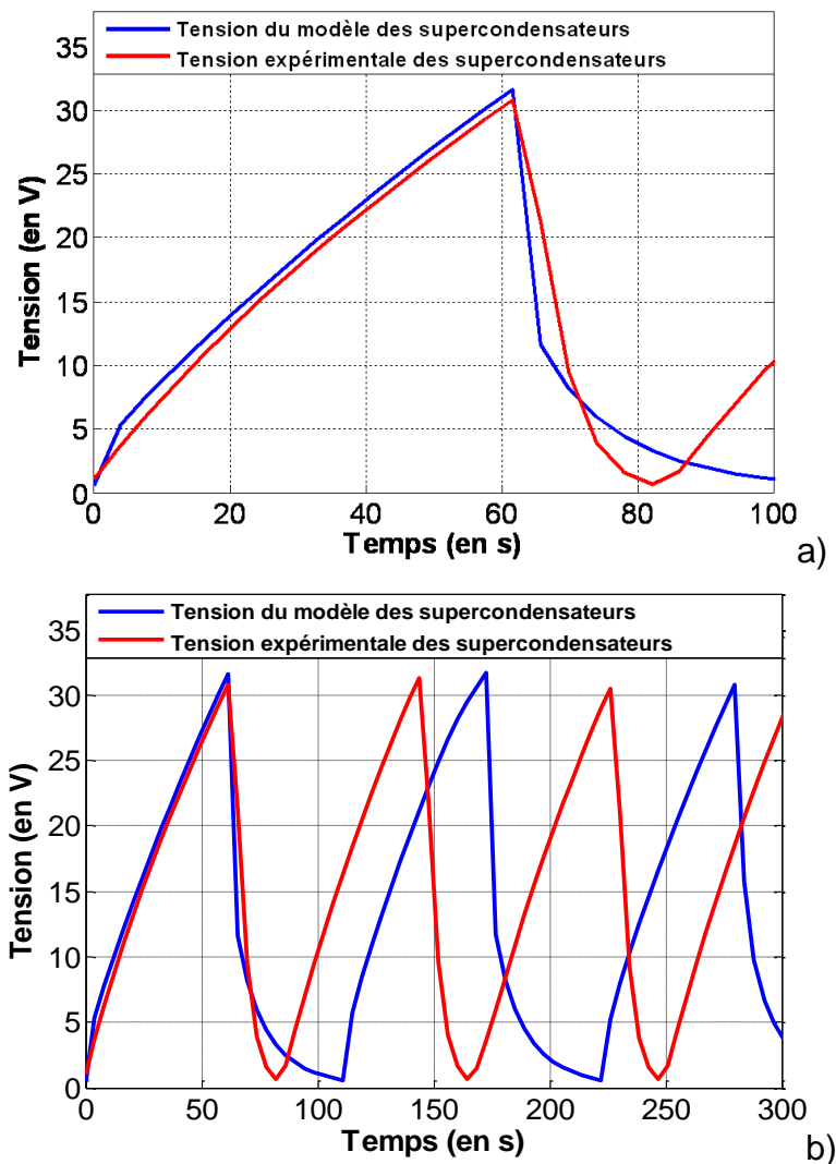
Figure 3.34. – Comparaison a) sur un cycle de charge/décharge du module de supercondensateurs ; b) sur plusieurs cycles qui se suivent.
