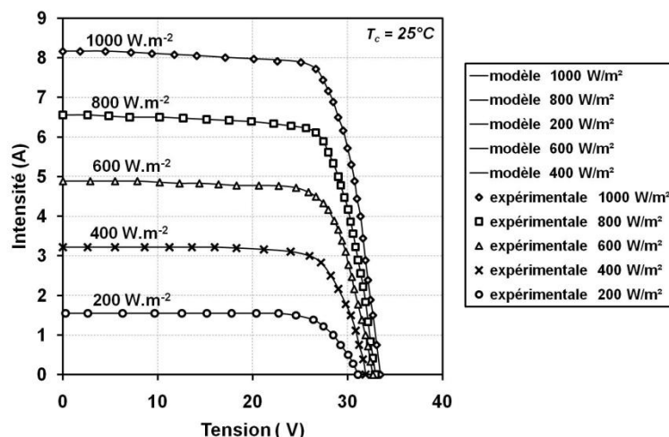
Figure 4.1 - Caractéristique courant-tension expérimentale et simulée pour le panneau photovoltaïque KC200GT avec une température de cellule de 25^\circ\text{C}
