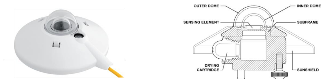
Figure 3.26. – Pyranomètre Kipp et Zonen CMP6 destiné à la mesure du rayonnement global (documentation Kipp et Zonen).
