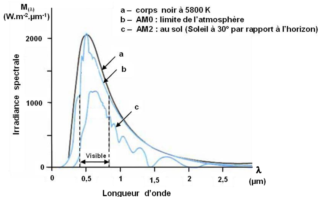
Figure 2.2 - Spectres solaires selon [Laugier et Roger 1981].
