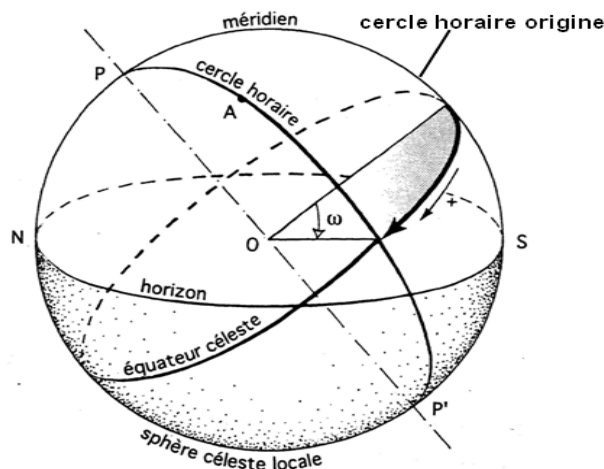
Figure 2.3 - Angle horaire \omega d'un point de la sphère céleste
