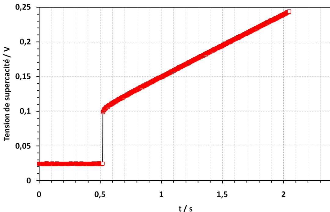
Figure 3.15 - Evolution de la tension de supercapacité en fonction du temps en échelle réduite
