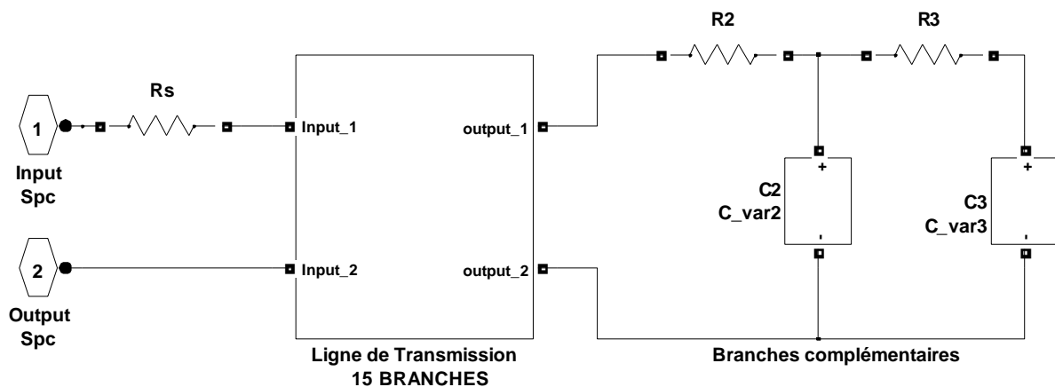
Figure 2.23 – Modèle multi-branche sous Simulink du supercondensateur (avec 15 branches).
