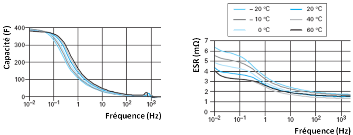
Figure 2.17 – Évolution de la capacité et de la résistance série d'un supercondensateur de capacité 350 F en fonction de la fréquence pour différentes températures.
