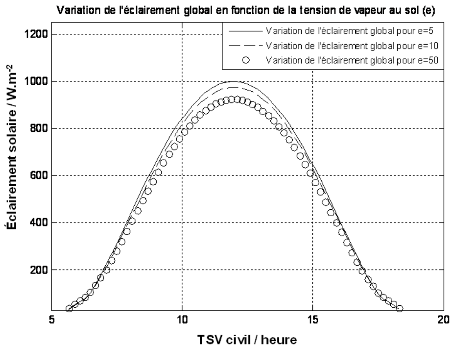
Figure 3.32– Variation de l'éclairement global reçu en fonction de " e ".
