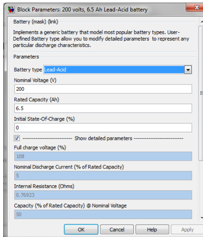
Figure 4.9 - Caractéristiques de la batterie plomb-acide choisie sous Matlab/Simulink
