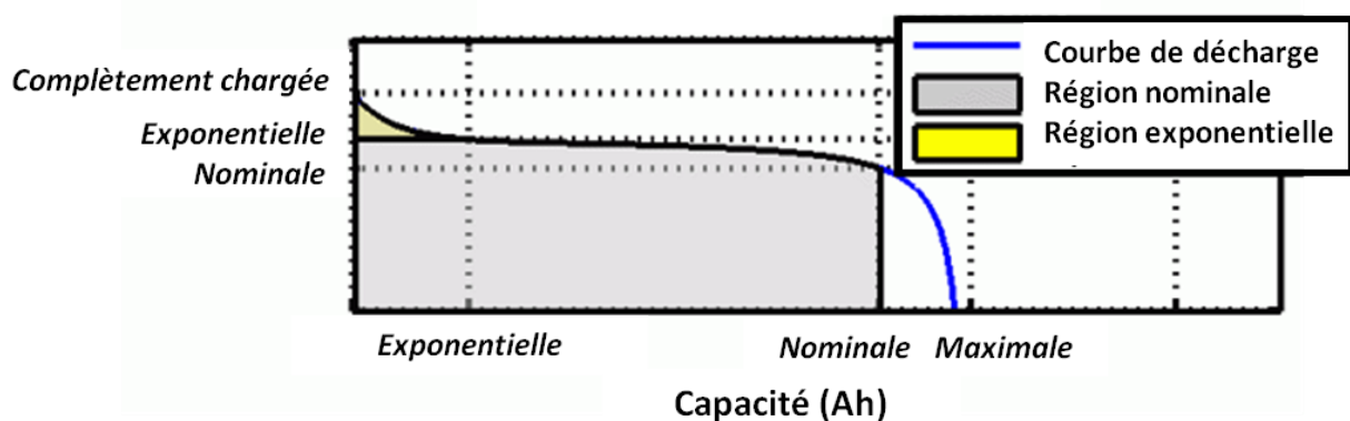
Figure 2.27 – Courbe de décharge d'une batterie.
