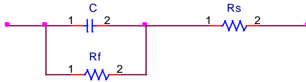
Figure 2.14. – Modélisation de base d'un supercondensateur.
