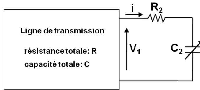
Figure 3.20 – Modèle équivalent du supercondensateur durant la phase de redistribution (première branche complémentaire).
