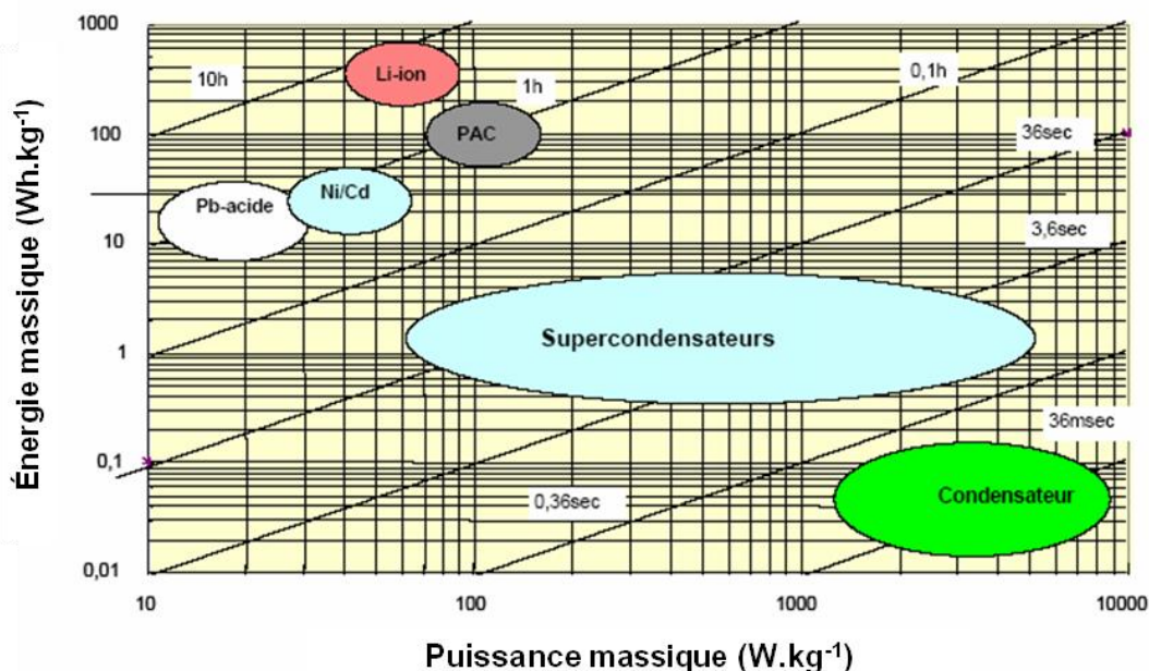
Figure 1.16 – Diagrammes de Ragone des systèmes électrochimiques de stockage d'énergie électrique.
