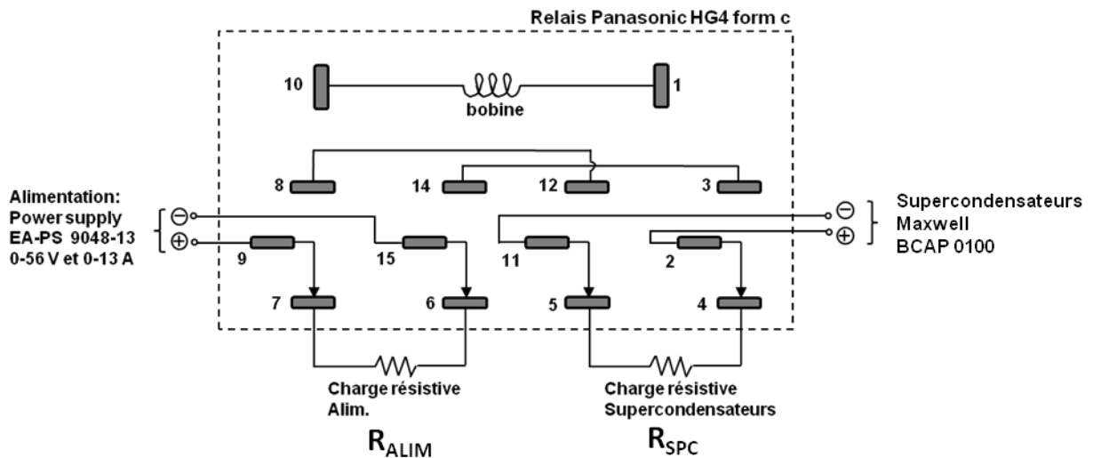
Figure 3.4 – Schéma de câblage du relais 1 pour réaliser un cycle de charge/décharge simple.
