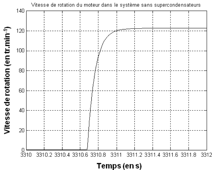
Figure 4.16 – Évolution de la vitesse de rotation du moteur à courant continu
