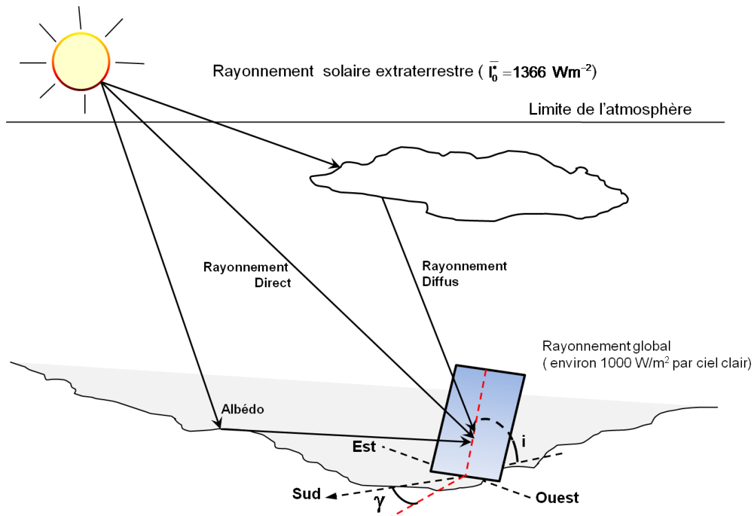
Figure 2.7 – Composantes du rayonnement solaire au sol.
