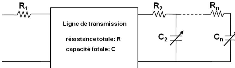
Figure 3.1 – Modèle multibranche d'un supercondensateur
