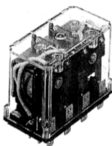
Figure 3.3- Relais Panasonic HG 4formc. La bobine excitatrice est alimentée par les contacts (1,10). Les entrées sont repérées par les contacts (9,15,11,2). Les sorties par les contacts (8,14,12,3) ou (7,6,5,4). Les contacts supportent jusqu'à 20 A sous 250 Volts AC. Le temps de réponse est 20 ms.
