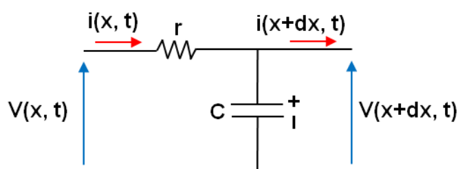
Figure 2.18 – Réseau de transmission.
