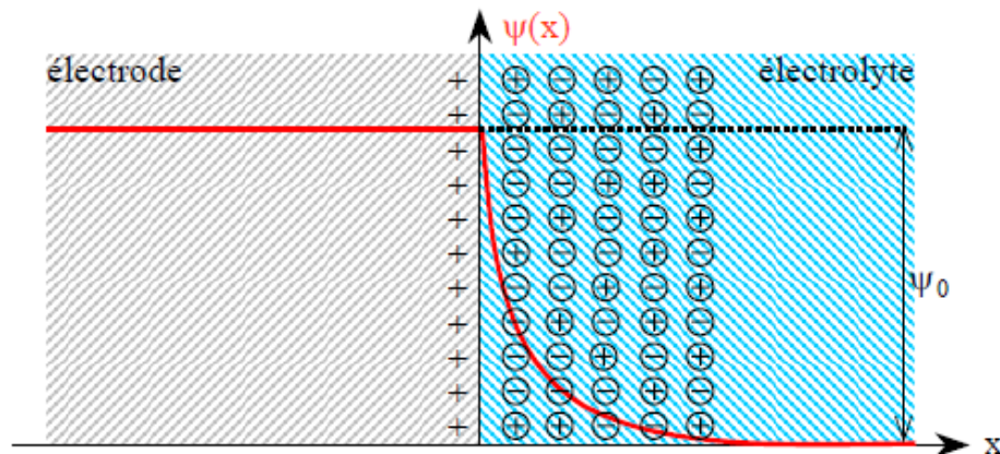
Figure 2.13. – Modèle de la couche double électrique d'après Gouy.
