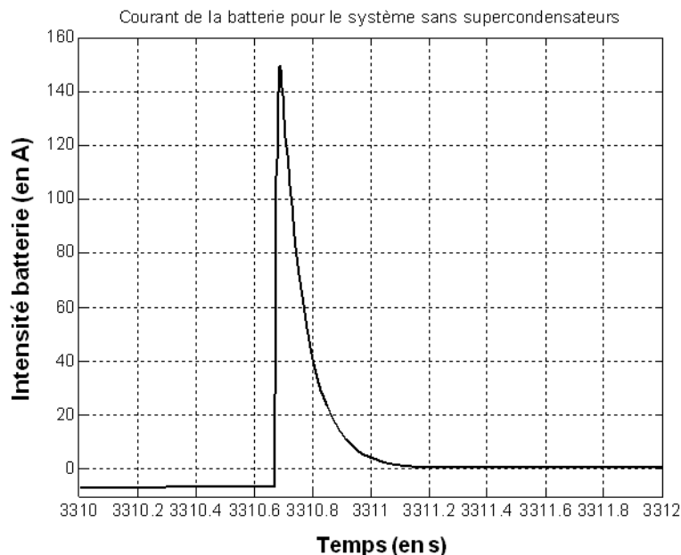
Figure 4.15 – Courant de la batterie (seule dans le système sans supercondensateurs)
