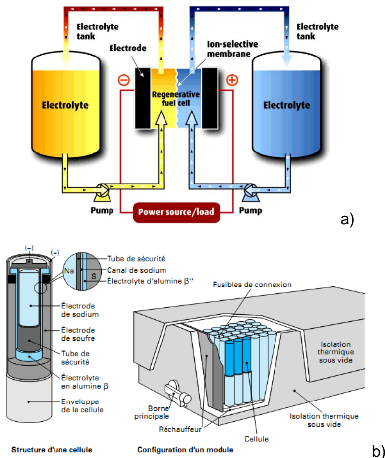
Figure 1.2. – Schéma de a) batterie à circulation b) batterie sodium-soufre.
