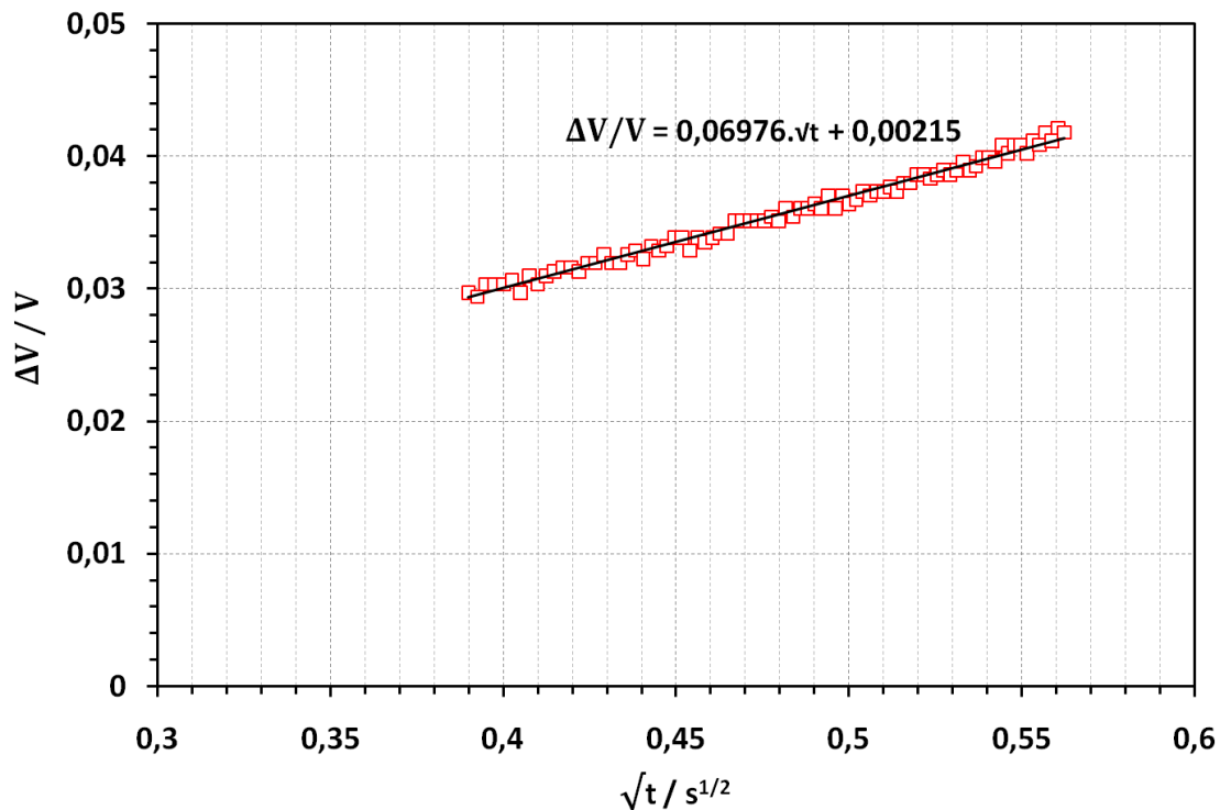
Figure 3.17 – Régression linéaire de \Delta V fonction de \sqrt{t} appliquée à l'intervalle des temps courts défini par t_{\min}=0,15 s et t_{\max}=0,32 s correspondant à la tension initiale de 2 V
