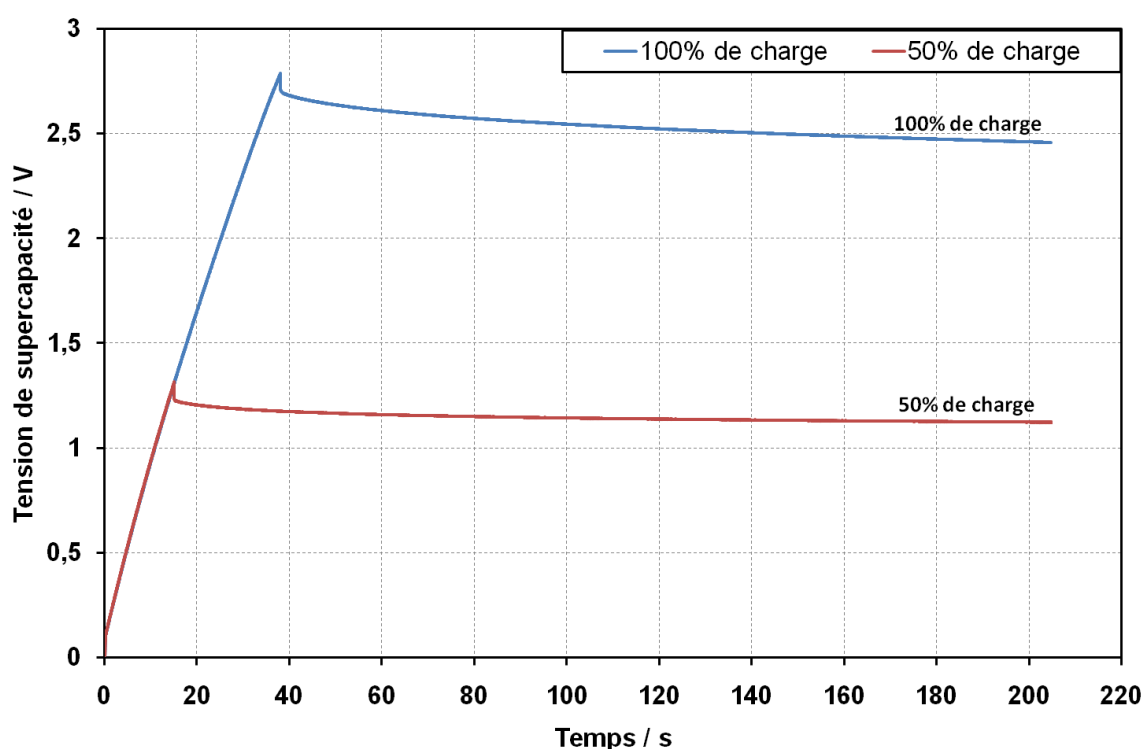
Figure 3.21 – Courbes de charge de deux supercondensateurs pour l'identification des branches complémentaires (courant de 7 A).
