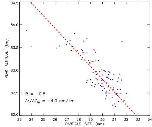
Fig. 5.19: Moyennes journalières de l'altitude des nuages en fonction des moyennes journalières de la taille des particules. Les points représentés en gris sont basés sur un nombre de données trop faible pour être pris en compte pour le calcul de la régression linéaire (droite rouge pointillée).
