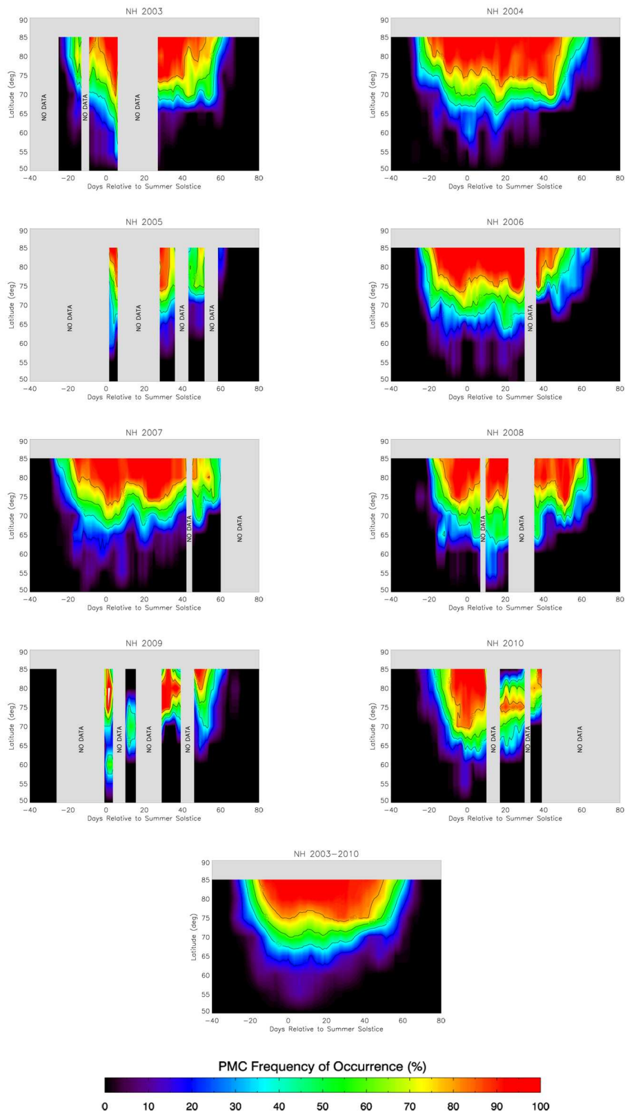
Fig. 4.6: Fréquence d'occurrence journalière, calculée pour des bandes de latitudes de 5° dans l'hémisphère Nord. Chaque été est représenté pour la période 2003-2010. Le graphique du bas correspond à la moyenne des 8 saisons représentées au-dessus.
