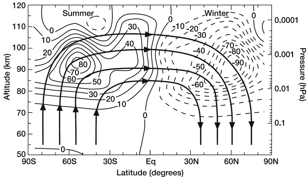
Fig. 1.6: Modélisation de la distribution méridienne du forçage dû à la dissipation de la quantité de mouvement des ondes de gravité dans l'atmosphère (en \text{m.s}^{-1}/\text{jour} ). Les valeurs positives correspondent à une orientation vers l'est. Les flèches en gras schématisent la circulation méridienne du pôle d'été vers le pôle d'hiver qui résulte de l'effet de ce forçage sur l'écoulement moyen zonal. (Brasseur and Solomon, 2005)
