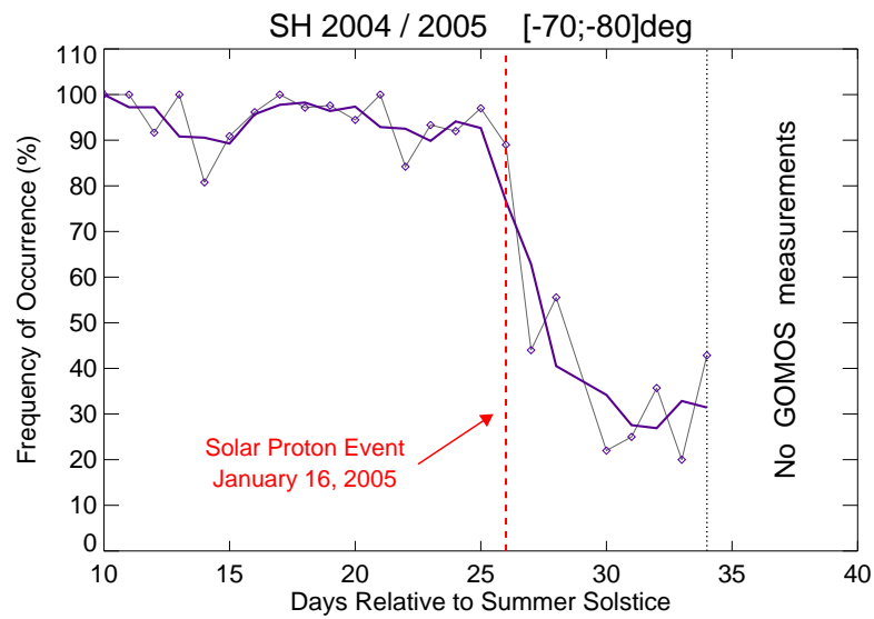
Fig. 4.9: Réponse de la fréquence d'apparition des nuages noctulescents entre -70^{\circ} et -80^{\circ} de latitude à l'événement à protons qui a eu lieu le 16 janvier 2005. Chaque symbole correspond à une moyenne zonale journalière. La ligne violette a été obtenue par application d'une moyenne glissante sur 3 jours.
