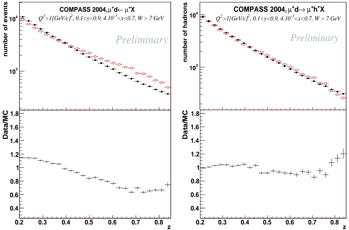
Figure 4: Comparaison des données réelles (noir) aux données Monte Carlo (rouge) en fonction de la fraction d'énergie des hadrons pour le tuning de défaut et le nouveau tuning.
