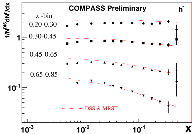
(b) multiplicités de h^-
