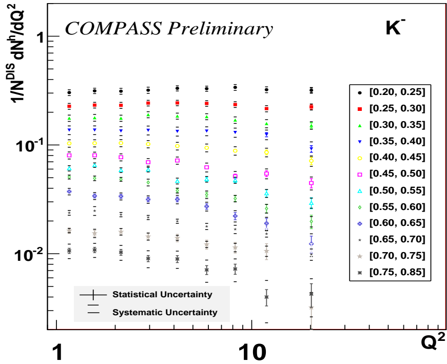
(b) multiplicités des K -
