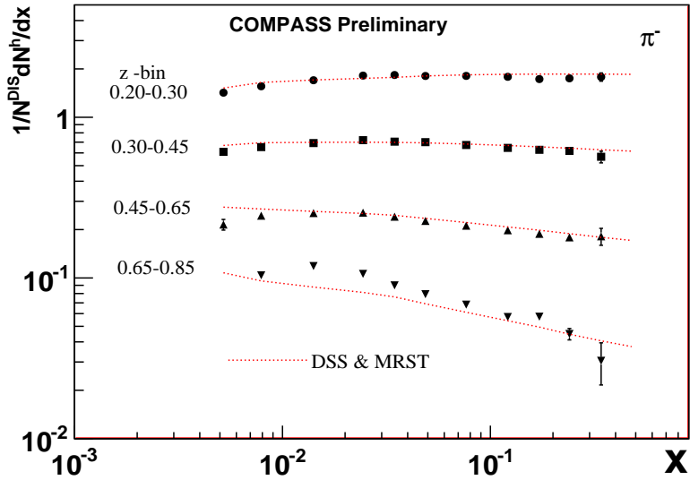
(b) multiplicités de \pi^-
