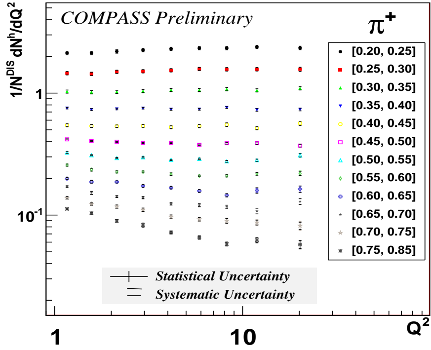
(a) multiplicités des \pi^+
