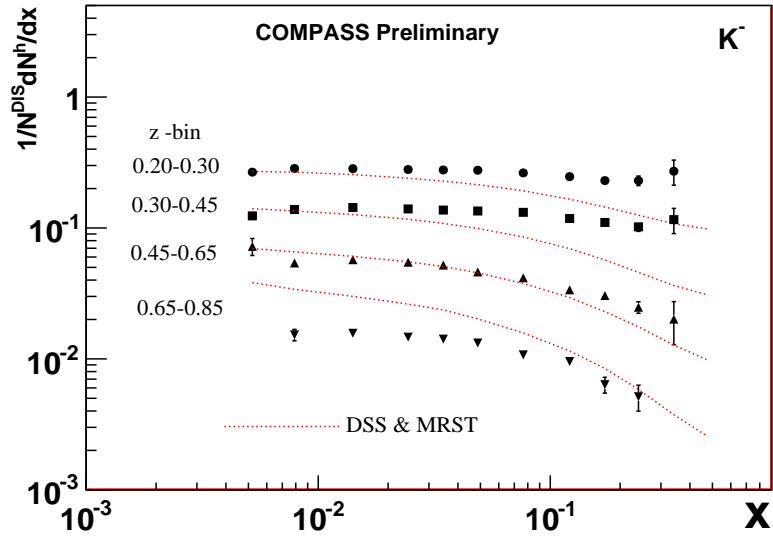
(b) multiplicités de K^-
