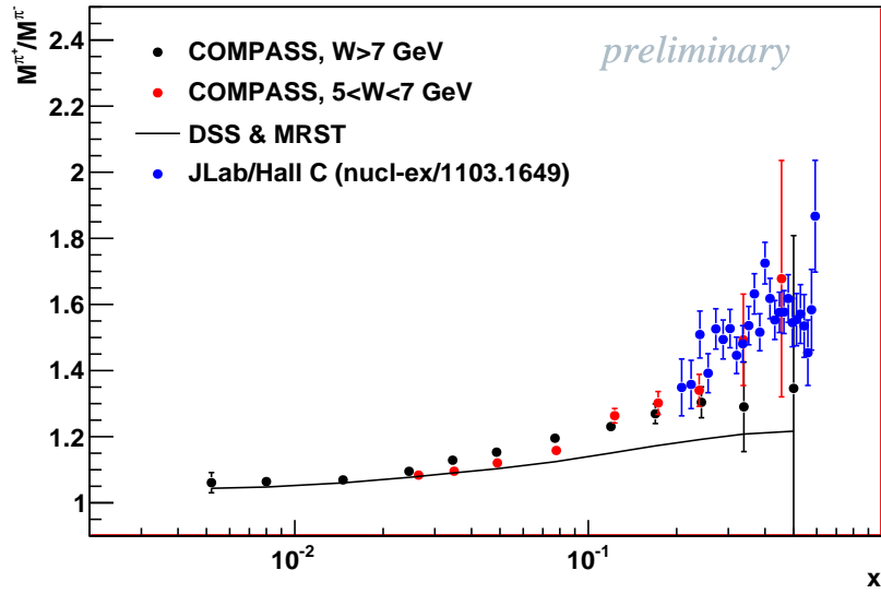
Figure 10: Rapport des multiplicités des pions positifs aux multiplicités de pions négatifs en fonction de x . Les erreurs présentées correspondent aux erreurs statistiques uniquement.
