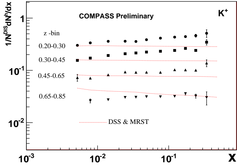
(a) multiplicités de K^+
