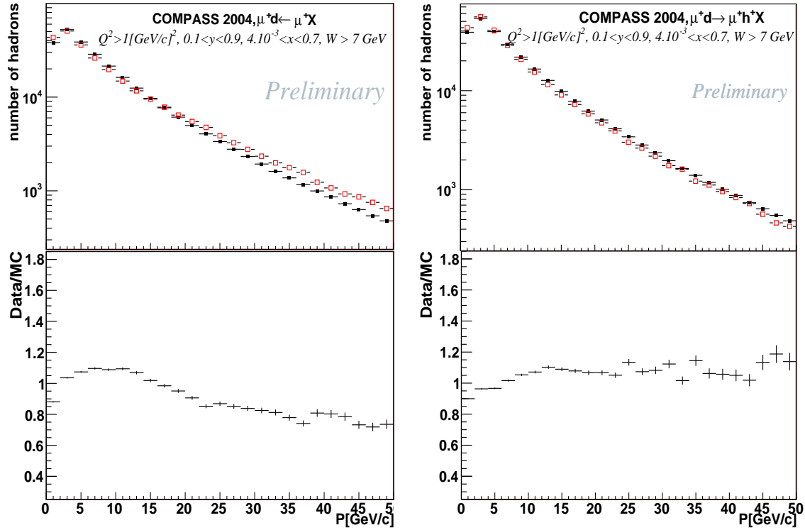
Figure 5: Comparaison des données réelles (noir) aux données Monte Carlo (rouge) en fonction de l'impulsion des hadrons pour le tuning de défaut et le nouveau tuning
