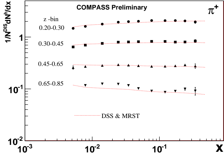
(a) multiplicités de \pi^+
