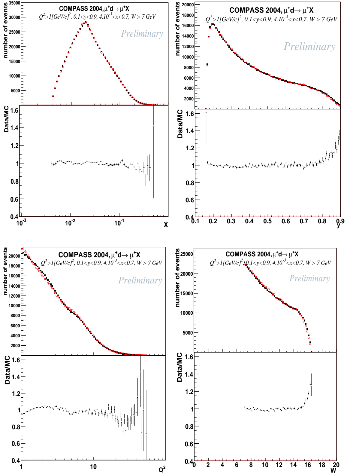
Figure 2: Comparaison des données réelles (points noirs) à la simulation Monte Carlo (points rouges) pour les variables inclusives x , y , Q^2 & W . La ligne supérieure montre les distributions des événements en fonction de ces variables alors que la ligne inférieure montre le rapport des données réelles aux données Monte Carlo.
