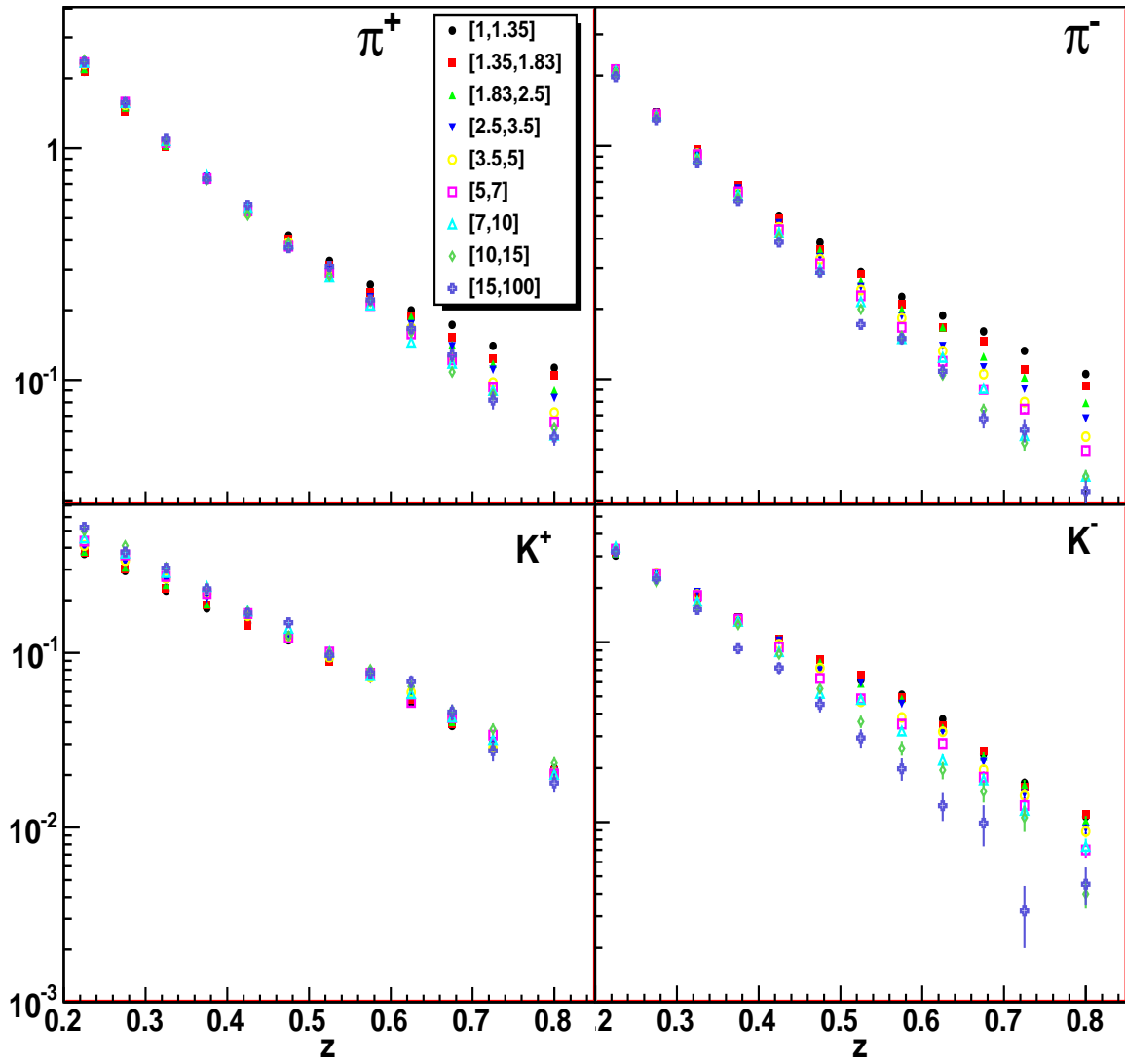
Figure 14: Multiplicités des pions et des kaons chargés en fonction de z pour 9 bins en Q^2 . Sont montrées uniquement les erreurs statistiques.
