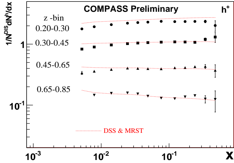
(a) multiplicités de h^+
