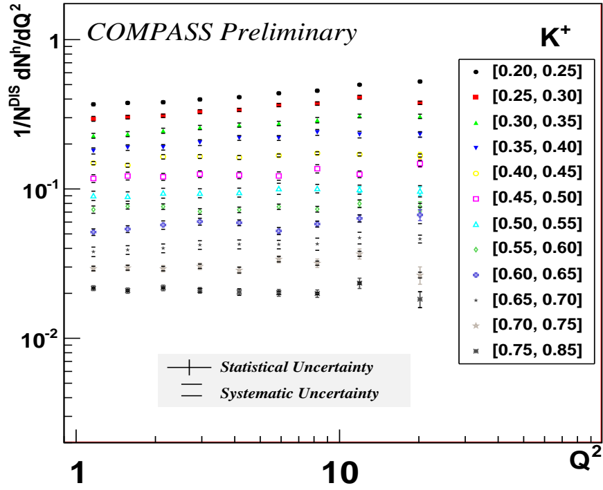
(a) multiplicités des K +
