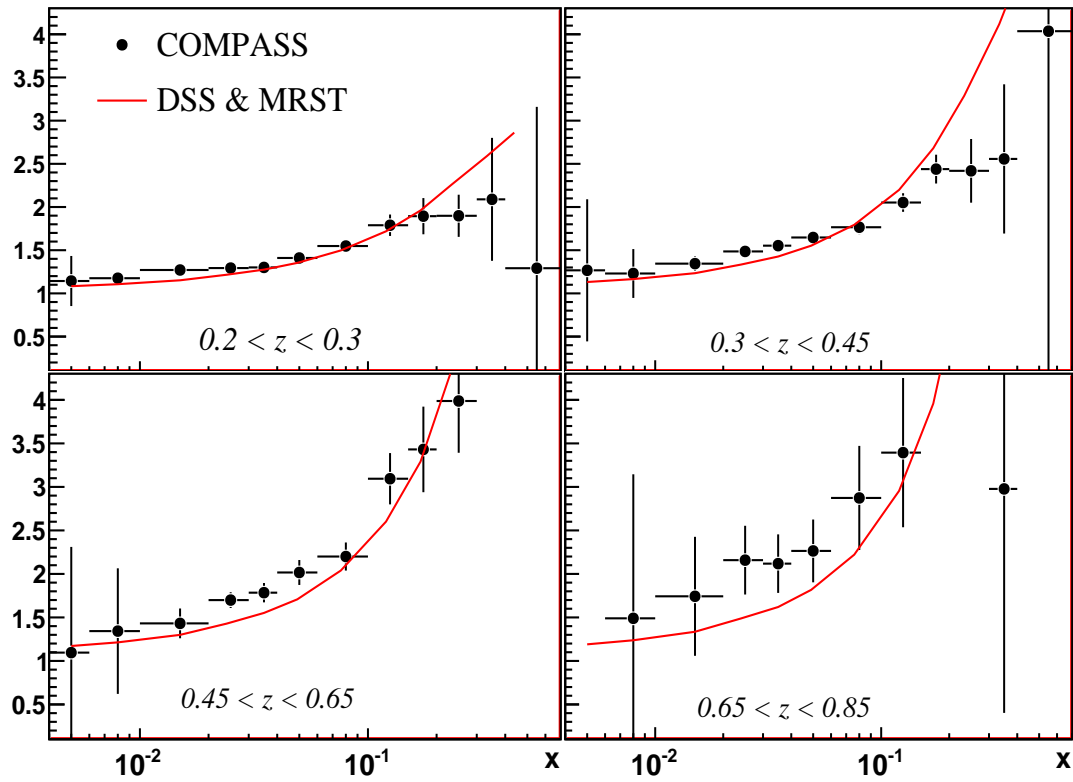
Figure 11: Rapport des multiplicités des pions positifs aux multiplicités de pions négatifs en fonction de x . Les erreurs présentées correspondent aux erreurs statistiques uniquement.
