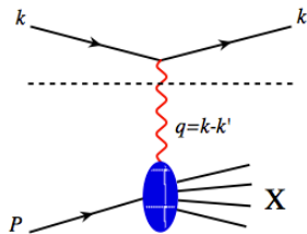
Figure 1: Diffusion d'un lepton sur un nucléon avec échange d'un photon virtuel.
