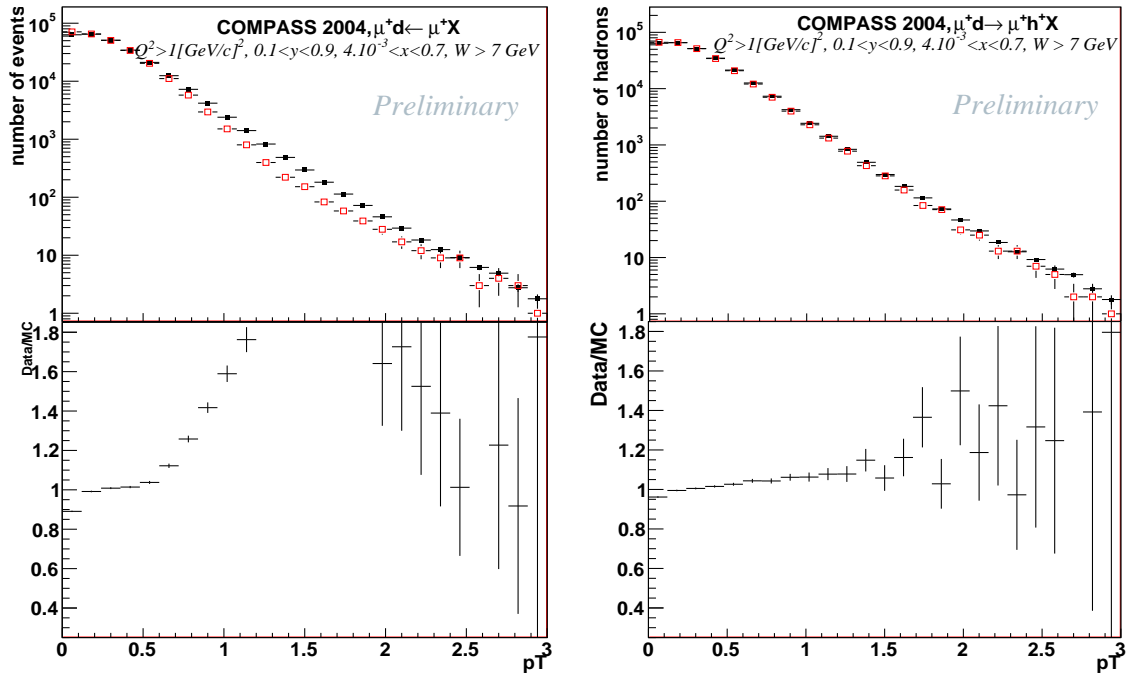
Figure 3: Comparaison des données réelles (noir) aux données Monte Carlo (rouge) en fonction du moment transverse des hadrons pour le tuning de défaut et le nouveau tuning.
