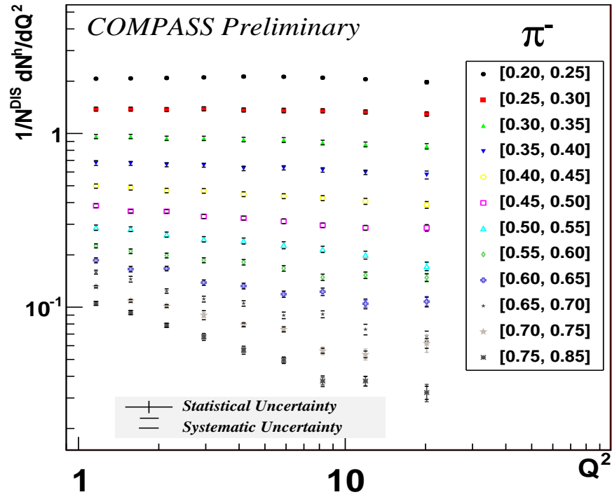
(b) multiplicités des \pi^-
