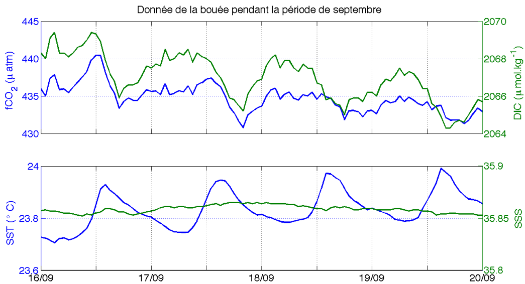
Figure IV.2 – Evolution du DIC, du fCO_2 , de la SST et de la SSS pendant la période "biologique" (septembre 2006) mesurés sur la bouée 6^{\circ}S , 10^{\circ}W .
