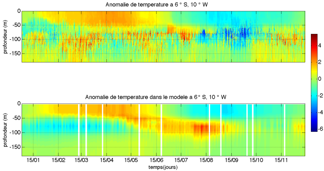
Figure E.3 – Anomalies de température a.) mesurée b.) simulée à 6° S, 10° W entre le 1/01/2007 et le 14/12/2007
