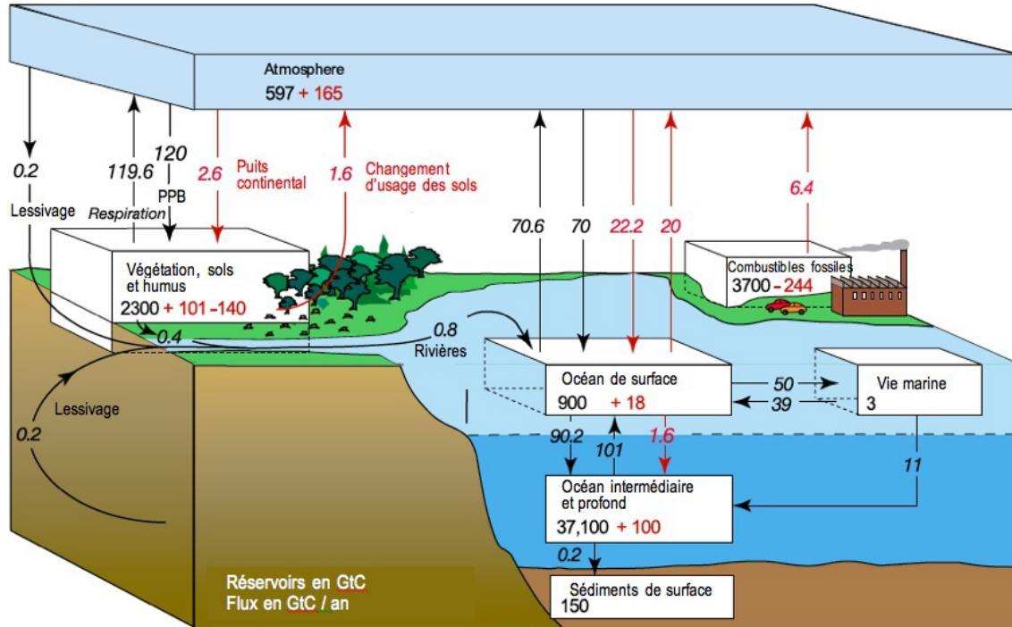
Figure I.1 – Le cycle du carbone depuis les années 1990. Les principaux flux annuels sont exprimés en GtC.an -1 . Les flux préindustriels sont en noir et les flux considérés comme liés à l'homme sont en rouge [IPCC, 2007].
