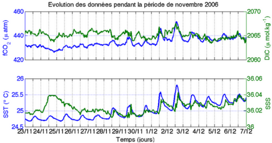
Figure IV.1 – Evolution du DIC, du fCO_2 , de la SST et de la SSS pendant la période "physique" (novembre-décembre 2006) mesurés sur la bouée 6^{\circ}S , 10^{\circ}W .
