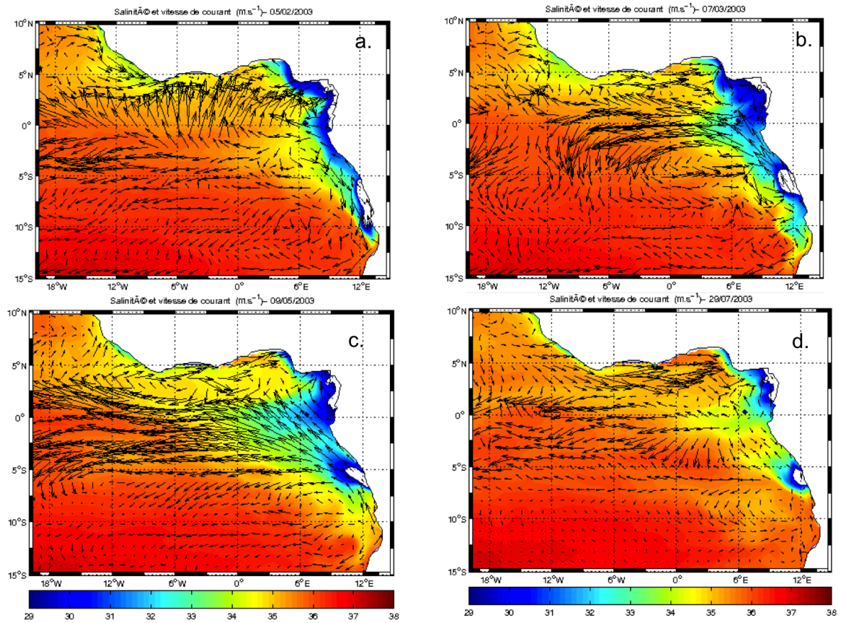
Figure V.9 – Carte de SSS et de courant dans l'Atlantique Est, a. fevrier 2003, b.) mars 2003 , c. mai 2003 et d.) juillet 2003.
