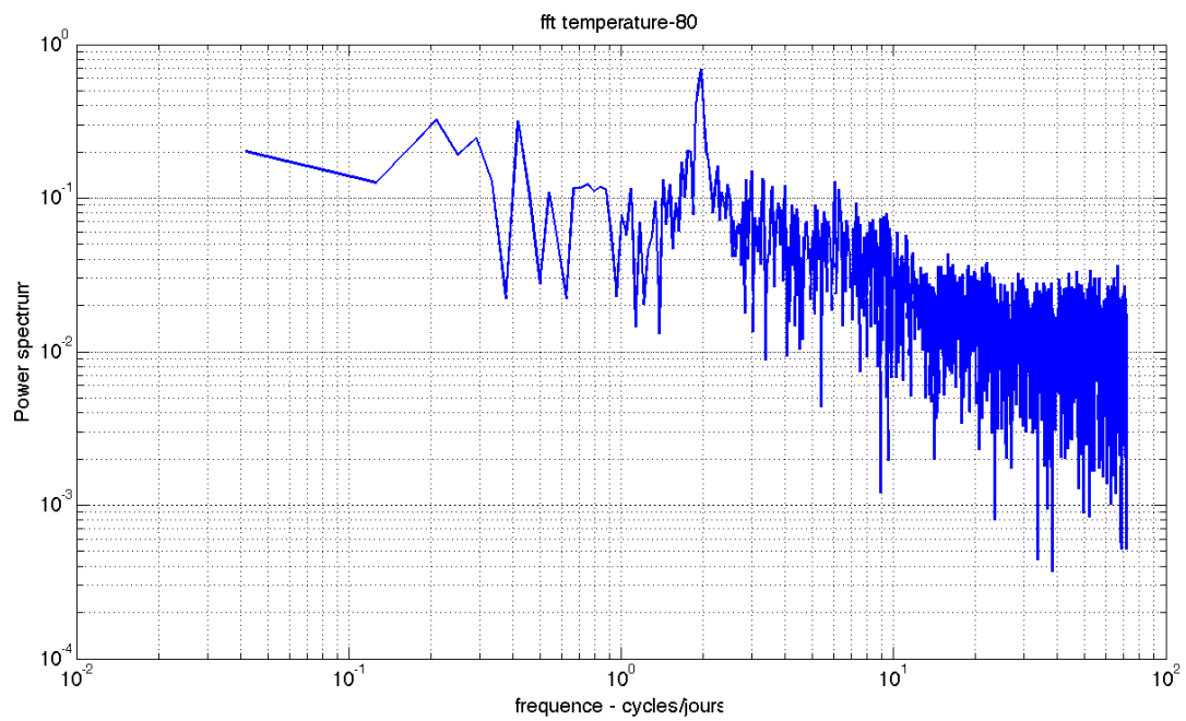
Figure IV.22 – Spectre de la température à 80 m.
