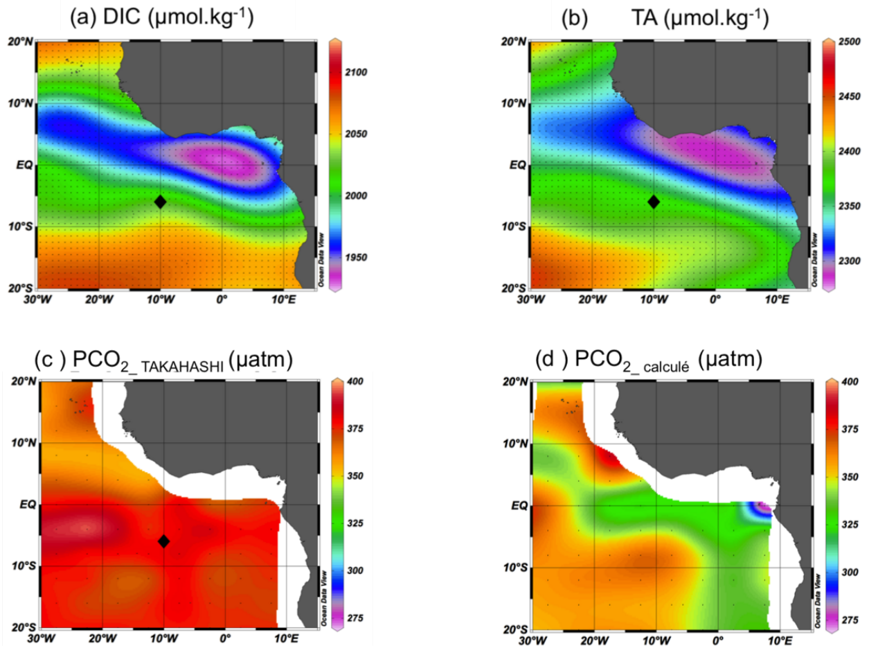
Figure I.10 – Carte issue de la climatologie annuelle [Key et al., 2004] pour DIC(a) et TA (b) et de [Takahashi et al., 2009] pour la \text{pCO}_2 (c). \text{pCO}_2_{\text{calculée}} correspond aux \text{pCO}_2 calculée à partir du DIC et de la TA de la climatologie avec le programme de [Lewis et Wallace, 1998].
