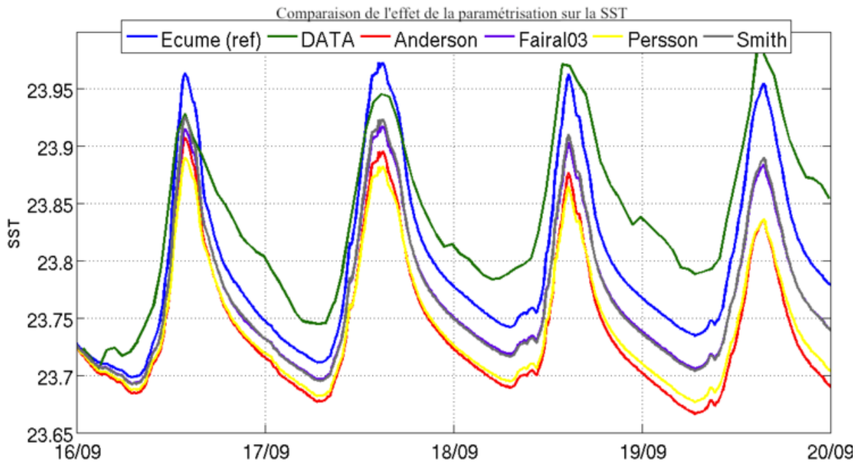
Figure IV.3 – Illustration de la SST calculée avec les 5 paramétrisations différentes : Anderson [1993], Fairall et al. [2003], Persson et al. [2005], Smith [1980] et ECUME.
