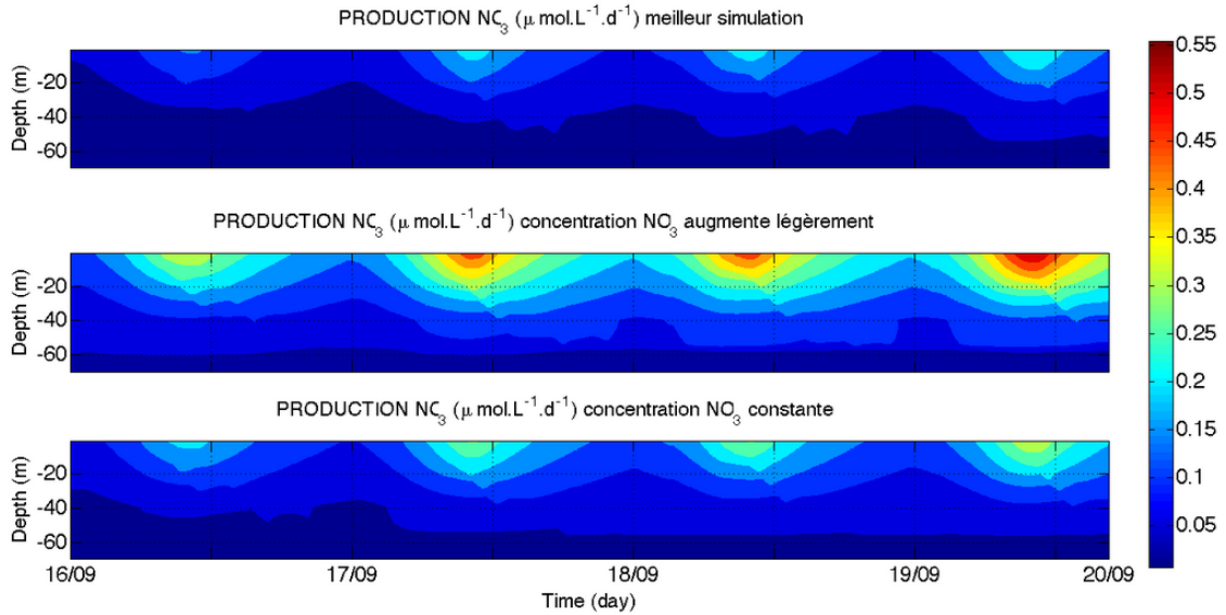
Figure C.6 – Evolution de la production de NO_3 dans la couche de mélange (haut : cas 1, milieu : cas 3 et bas : cas 2).
