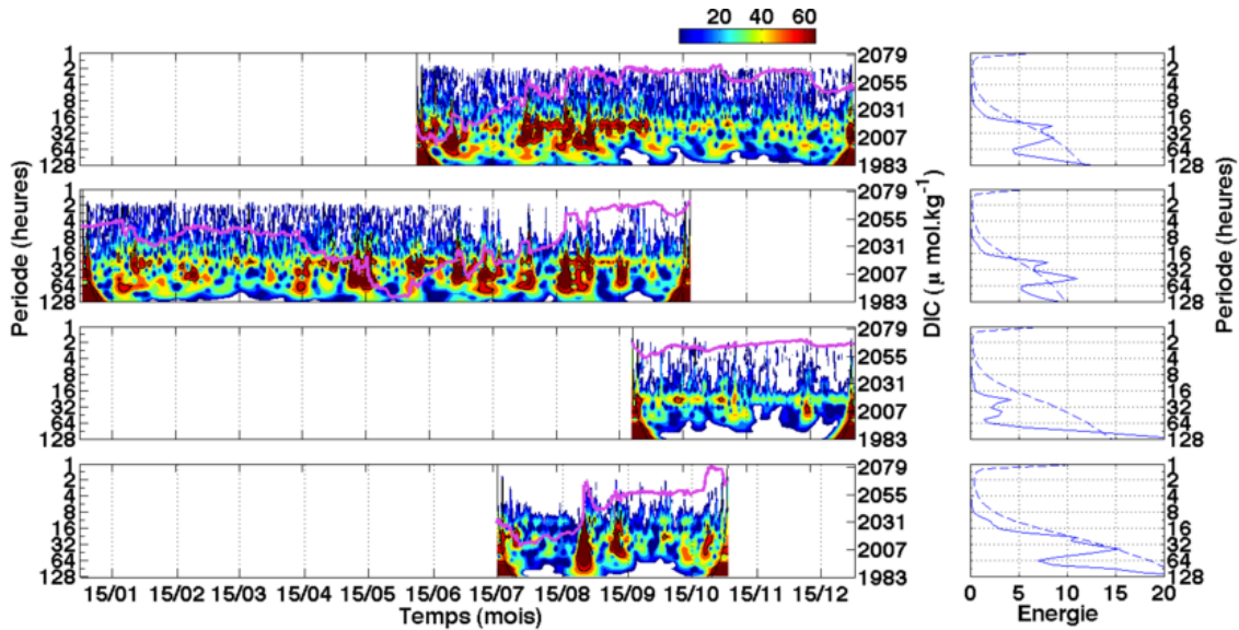
Figure III.1 – Ondelettes pour la variabilité de DIC au cours de 2006, 2007, 2008, 2009 et spectre en énergie pour chacune des années. Le trait mauve correspond à la série temporelle de DIC. A droite, l'énergie moyenne du spectre global (trait continu) avec les 95 % de confiance indiqué par le trait en pointillé.
