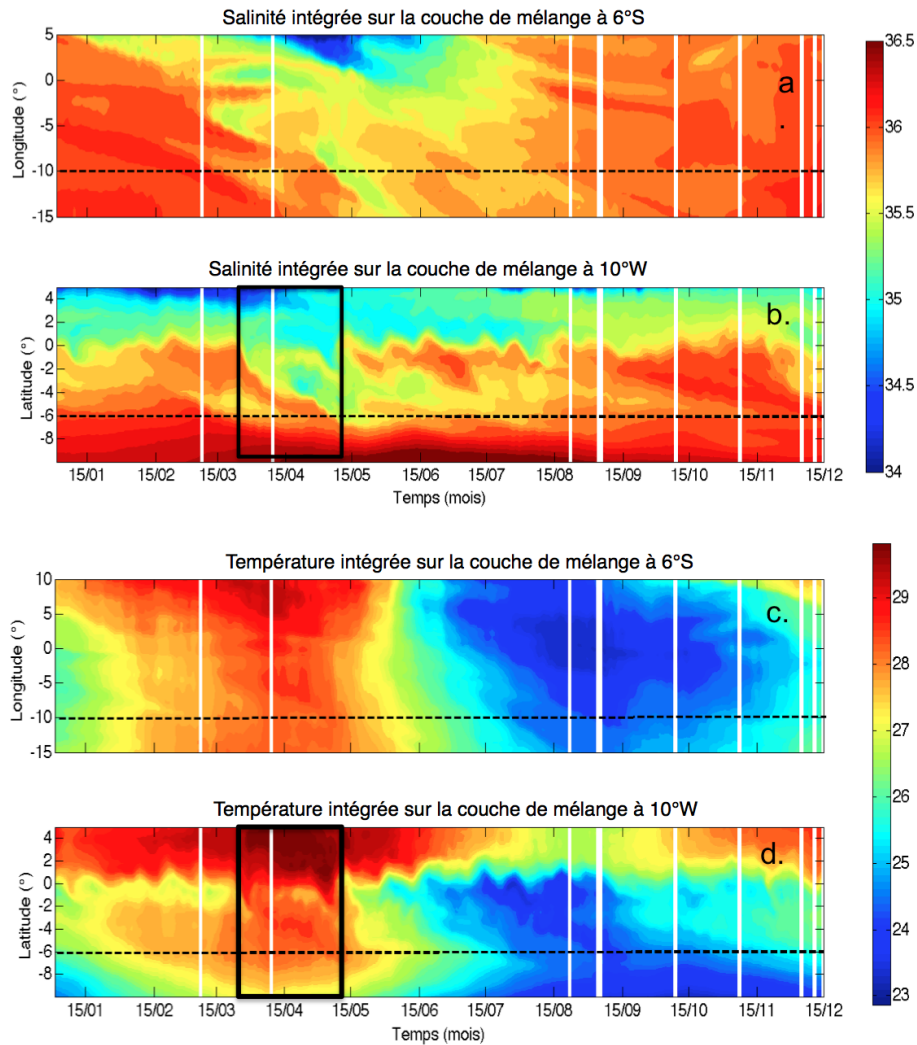
Figure V.10 – Evolution de la salinité et de la température dans la couche de mélange du modèle 2007 en fonction du temps et de la latitude. a.) salinité à 6°S, b.) salinité à 10°W c.) température à 6°S et d.) température à 10°W. La ligne en pointillés noirs correspond à la position de la bouée. Le rectangle noir correspond à des eaux chaudes ayant une faible salinité.
