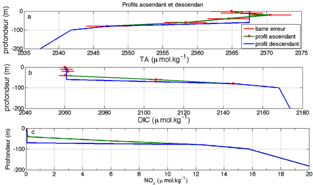
Figure IV.5 – Profils DIC et TA ascendants ajustés à partir des erreurs sur les mesures de \mu\text{mol.kg}^{-1} et ajustés à la profondeur de couche de mélange mesurée pendant E4d.
