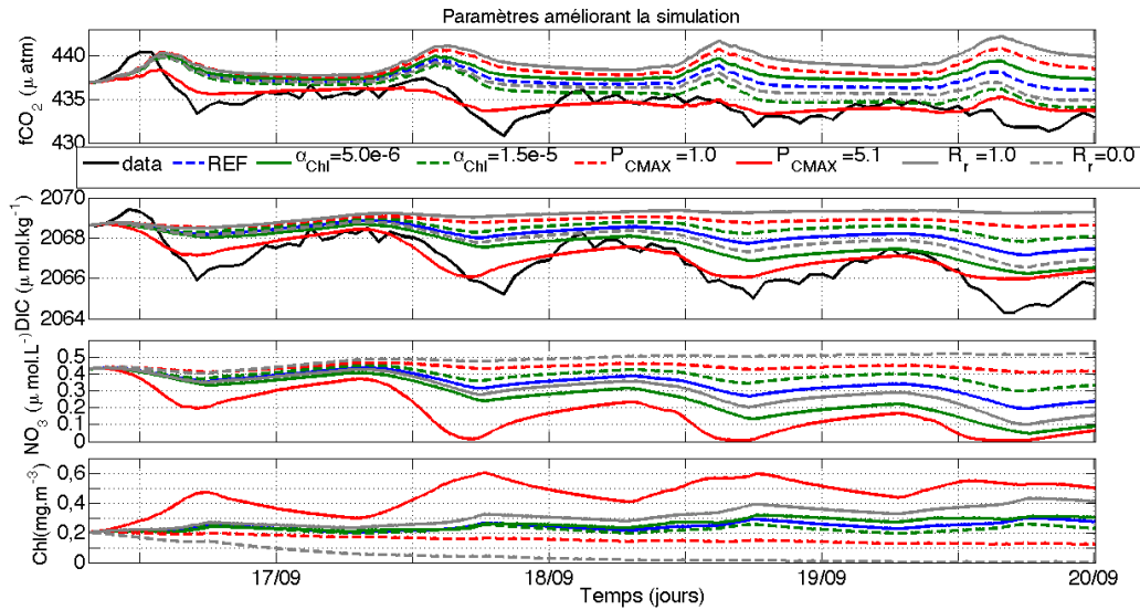
Figure C.8 – Evolution de la fCO 2 , du DIC, des NO 3 et de la chlorophylle.
