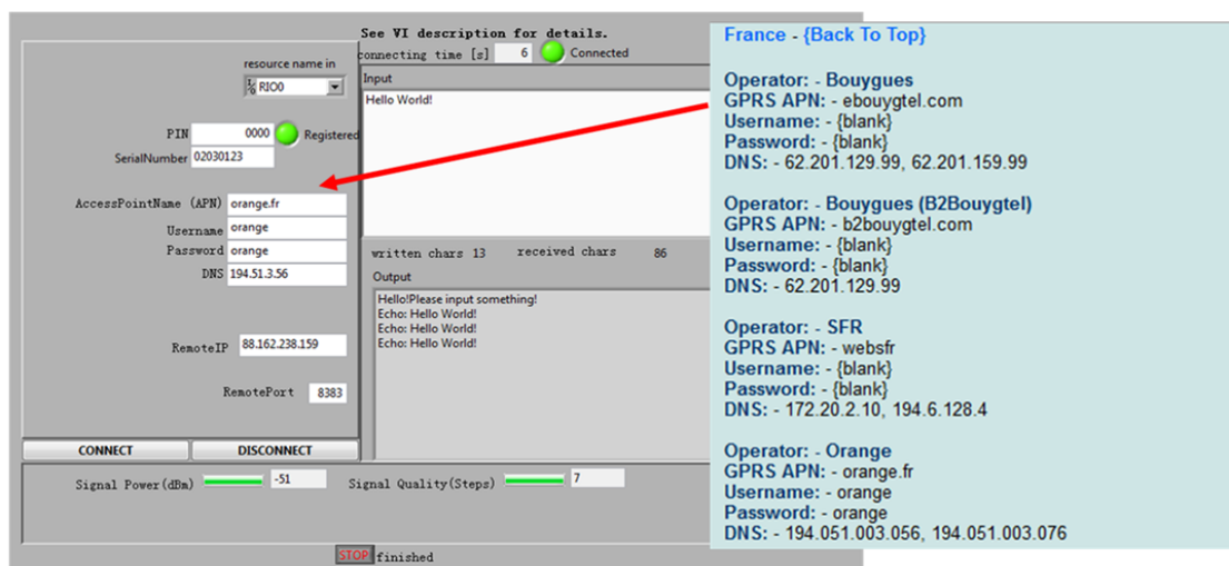
Figure II.19 – La transmission des données par GPRS.
