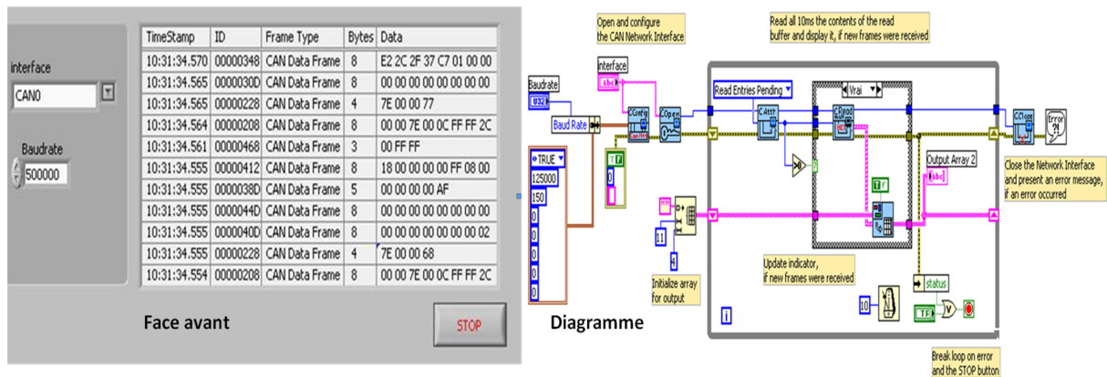
Figure II.10 – la trame reçue par le programme “CAN Receive”
