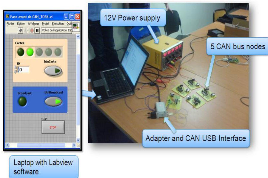
Figure II.6 – Test de fonctionnement sur table du bus CAN ouvert réalisé
