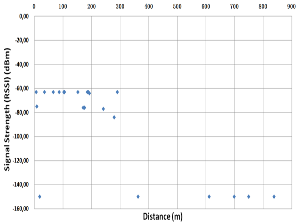
Figure III.18 – RSS et distance pour la zone urbaine
