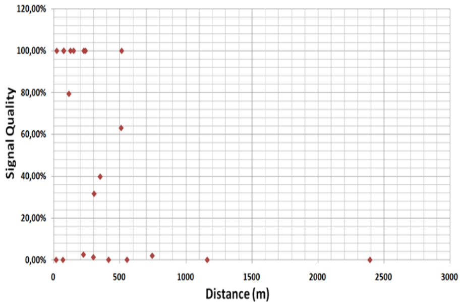
Figure III.21 – Qualité du signal et distance sur autoroute
