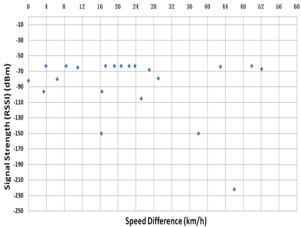
Figure III.17 – RSS et différence de vitesse sur autoroute
