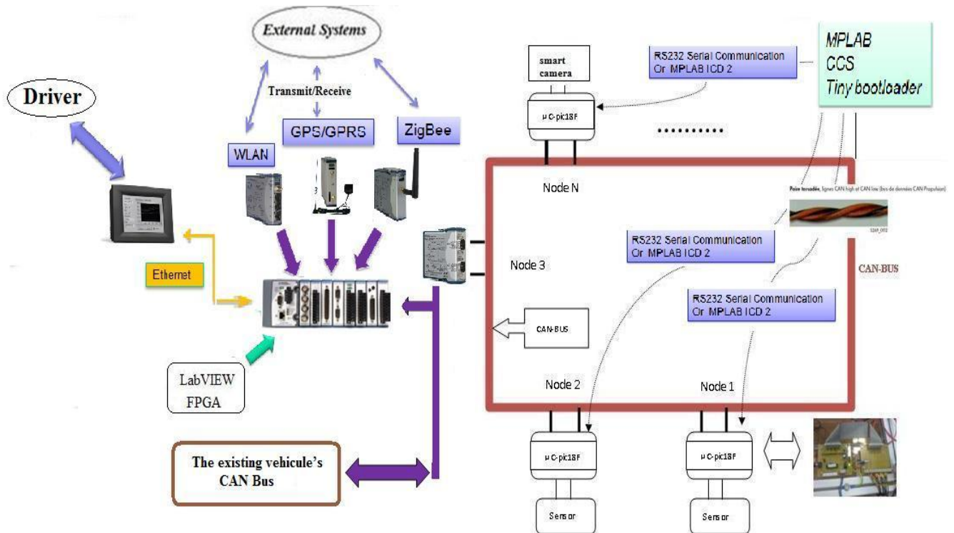
Figure II.3 – Le CAN pervasif avec le CRio
