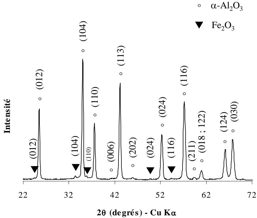
Figure III.1 : Diagramme de diffraction des rayons X du produit obtenu après calcination sous air à 1000^\circ\text{C} pendant 10 min de la solution solide amorphe \text{Al}_{1.8}\text{Fe}_{0.2}\text{O}_3
