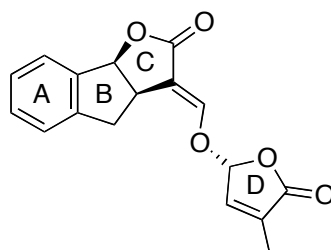
Schéma 141 : Structure du GR-24, analogue synthétique des strigolactones naturelles
