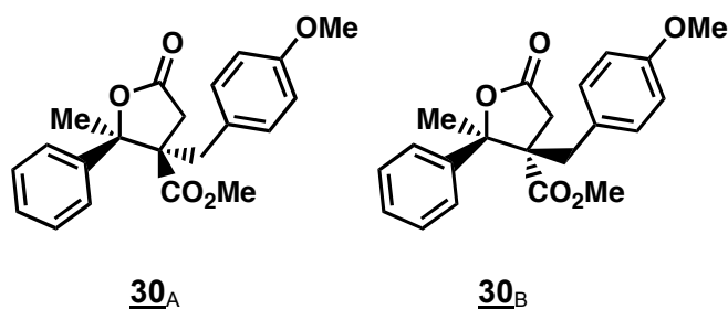
Schéma 118 : Diastéréoisomères A et B de 30
