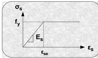
Figure 3-76 : Loi de comportement des aciers longitudinaux utilisée dans le logiciel Beam Compo.
