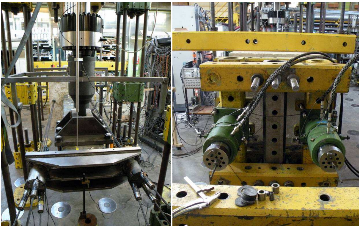
Figure 3-20 : Détails des plaques d'ancrage des câbles de précontrainte à l'avant puis à l'arrière du corps d'épreuve.
