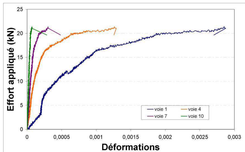
Figure A3- 15: Propagation des déformations sur l'axe gauche de la lamelle SLAc3i – avant décollement de la lamelle.
