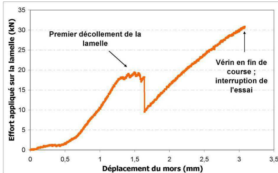
Figure A2- 7: Courbe Effort/Déplacement du mors – Bloc SLA2 / 1 ère phase.
