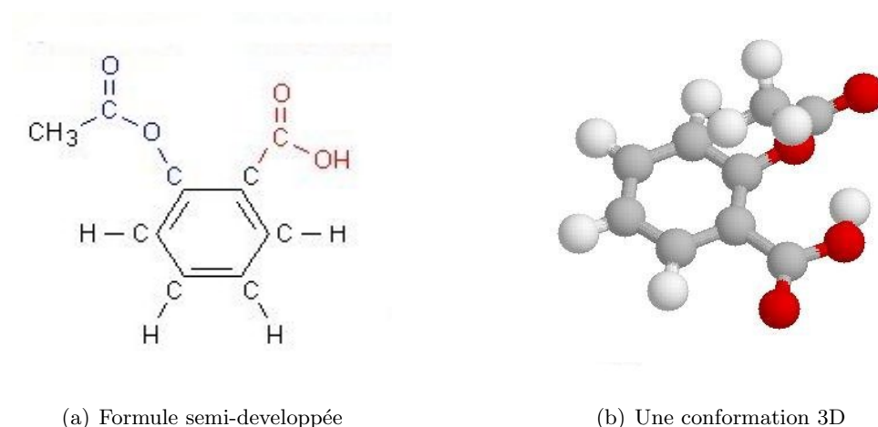
FIGURE 1.1: Représentations 2D et 3D de l'aspirine
