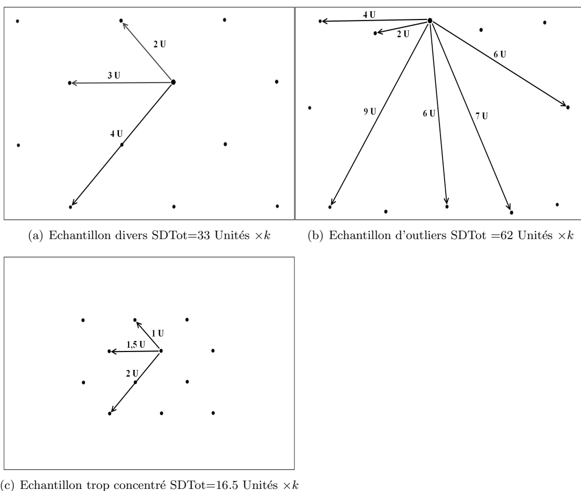
FIGURE 4.8: Visualisation de la dissimilarité totale de différents échantillons (les chiffres sont expliqués par la suite)
