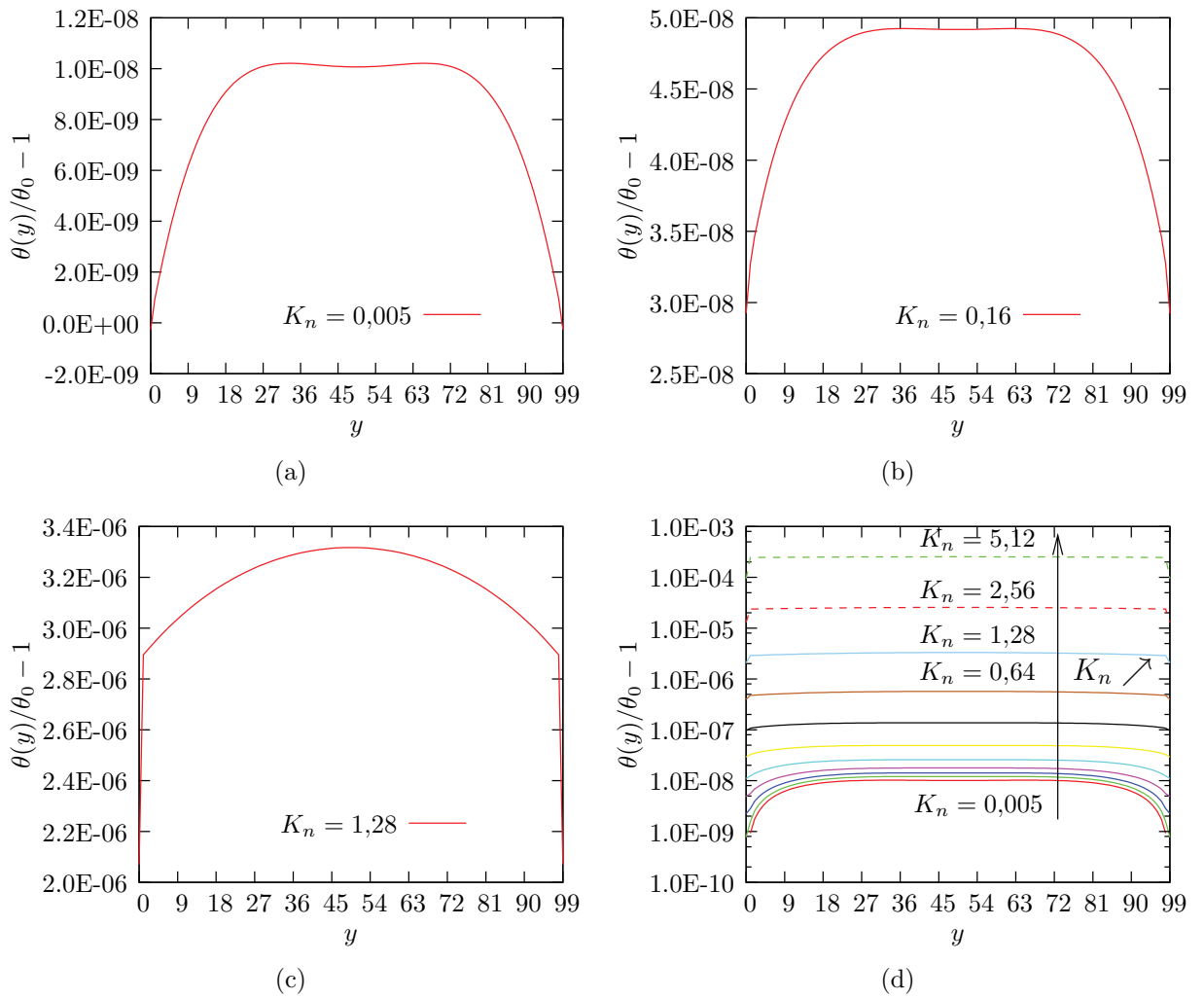
FIGURE 6.16 – Champs de température pour différents nombres de Knudsen et un nombre de Mach Ma = 0,0001 . Résultats obtenus grâce au schéma basé sur \mathcal{H}_{4|5} . Sur la figure (d) les abscisses sont en échelle logarithme.
