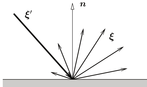
FIGURE 4.1 – Illustration de la diffusion par une paroi d'un faisceau de particules incidentes à la vitesse \xi' . La vitesse des particules réémises est notée \xi . Le vecteur n est la normale à la paroi, dirigée vers le fluide.
