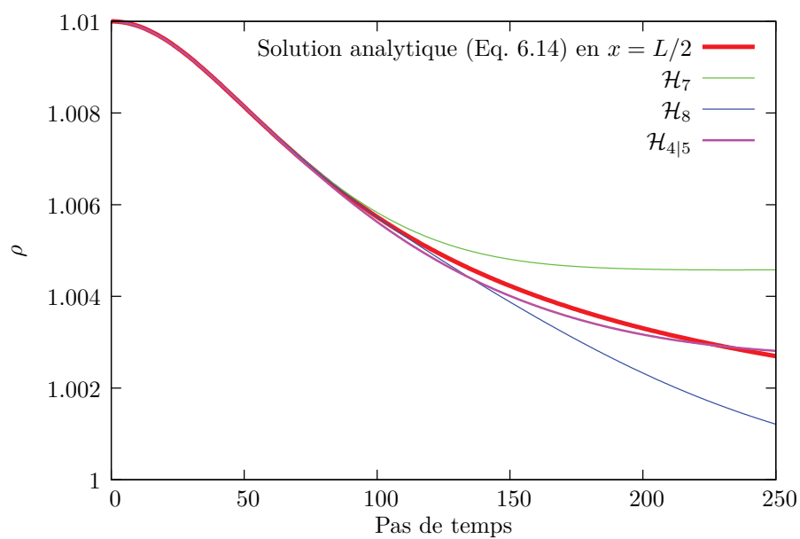
FIGURE 6.4 – Valeur de la densité \rho(L/2,t) en fonction du temps discret en x = L/2 , position où la densité est maximale. Comparaison de la quadrature composite \mathcal{H}_{4|5} avec deux quadratures “pures” d’ordres équivalents.
