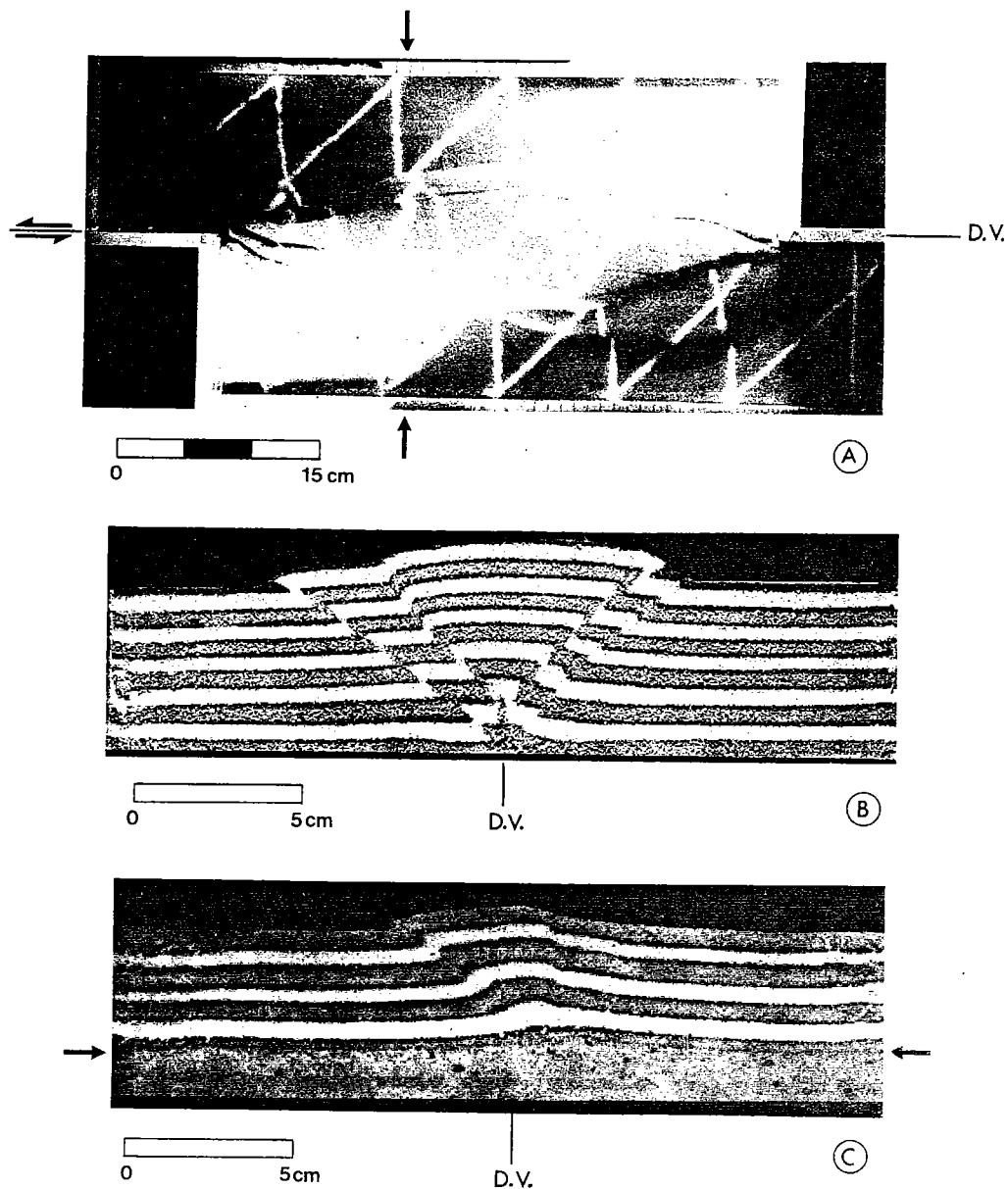
Fig. 3. — Planché photo : vue de dessus et coupes de modèles après déformation ( R = 1/3 ). (A) Vue de dessus d'un modèle de type fragile montrant un réseau de failles décrochevauchantes. Les flèches localisent la coupe B. (B) Coupe dans un modèle de type fragile. On note un fuseau de failles inverses (pendage moyen 50^\circ ), soit rectilignes, soit courbes, mais convergentes à la base du modèle. Les failles s'enracinent sur la discontinuité de vitesse basale (D. V.). (C) Coupe dans un modèle de type fragile-ductile. Les flèches indiquent l'interface sable-silicone. Trois plans de faille sont observables et leur pendage varient de 40 à 90^\circ .
