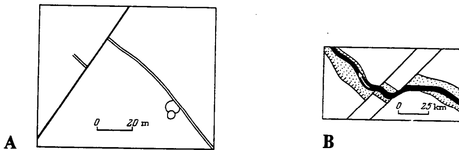
Fig. 1 - 17. Exemples de jeux récents sénestres sur la faille de Darvaz-Karakul (Afghanistan - Badakhstan). A - Mur médiéval tronçonné par une faille sénestre. B - Vallée éocène décalée le long de deux décrochements sénestres (d'après Kuchay and Trifonov, 1977).
