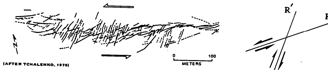
Fig. 1 - 3. Exemple naturel de Riedel R synthétiques et de Riedel R' antithétiques d'un décrochement sénestre. Ces structures ont été créées lors du tremblement de terre de Dash-e Bayaz (Iran) décrit par Tchalenko and Ambraseys (1970), Tchalenko (1970).
