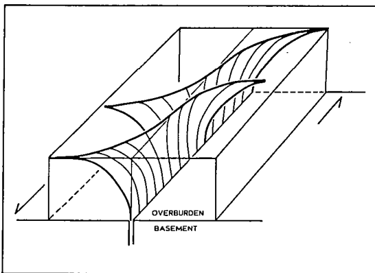
Fig. 1 - 9. Géométrie hélicoïdale théorique de plans axiaux de plis en échelon associés à un décrochement sénestre. Cette interprétation est inspirée des travaux analogiques de Naylor et al. (1986) sur la géométrie des Riedels et de descriptions d'exemples naturels de Sylvester and Smith (1976) et Gamond and Odonne (1984) (d'après Sylvester, 1988).
