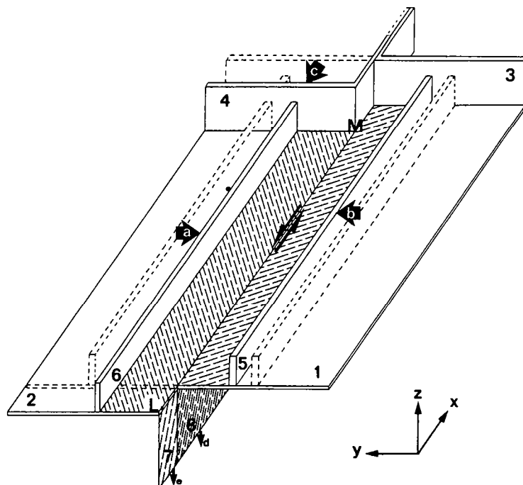
Fig. 2. — Vue en perspective du dispositif expérimental montrant les plaques basales (1, 2), plaque en « L » (3, 4), pistons (5, 6), feuilles plastiques (7, 8) et ligne médiane (L. M.), ainsi que les déplacements imposés aux pistons (a, b), déplacement imposé aux plaques 2 et 4 (c) et le sens de plongement des feuilles plastiques (d, e). Les flèches situées au centre du modèle, parallèles à la ligne médiane, indiquent le déplacement relatif des plaques 1 et 2. Les pointillés représentent un état initial, les traits pleins, un état final.
