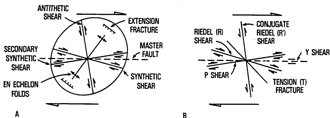
Fig. 1 - 2. Relations angulaires entre les structures caractéristiques susceptibles de se développer dans la couverture sédimentaire, au dessus d'un décrochement de socle (d'après Christie-Blick and Biddle, 1985).
