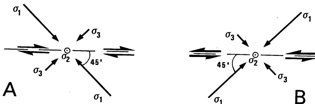
Fig. 1 - 1. Champ de contraintes associé à un décrochement.
