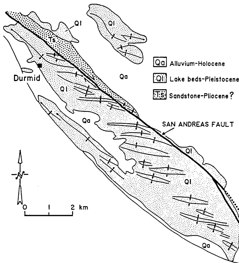
Fig 1 - 11. Plis en échelon affectant les sédiments d'âge Plio-Pléistocène le long de la faille de San Andreas près de Salton sea (d'après Dibble, 1977). Les plis en échelon sont disposés le long d'une faille décrochante dextre. Cependant, leur formation est certainement due à un décrochement dextre de socle masqué par la couverture sédimentaire, à l'aplomb de la zone plissée (Sylvester, 1988).
