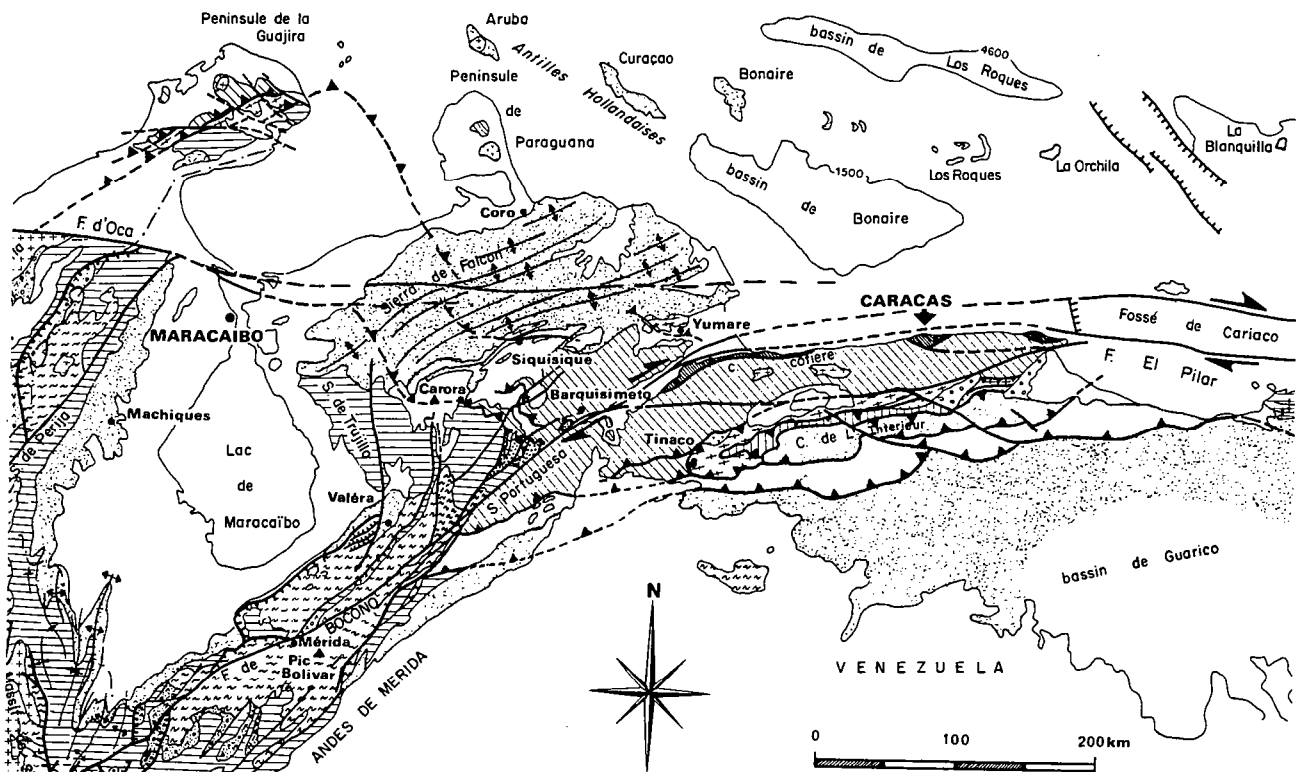
Fig. 7 - 2 Grands traits structuraux du Nord-Ouest du Venezuela (d'après Stéphan, 1985).
