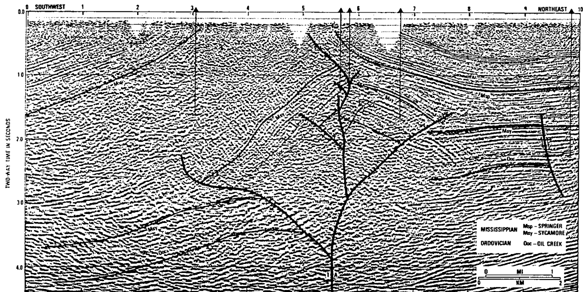
Fig. 1 - 14. Structure en fleur dans le bassin d'Ardmore (Oklahoma). (A) Schéma structural du Bassin. (B) Profil sismique orienté Sud Ouest - Nord Est, perpendiculairement à la direction de déplacement. Ce profil se situe sur une faille secondaire (d'après Harding, 1985).
