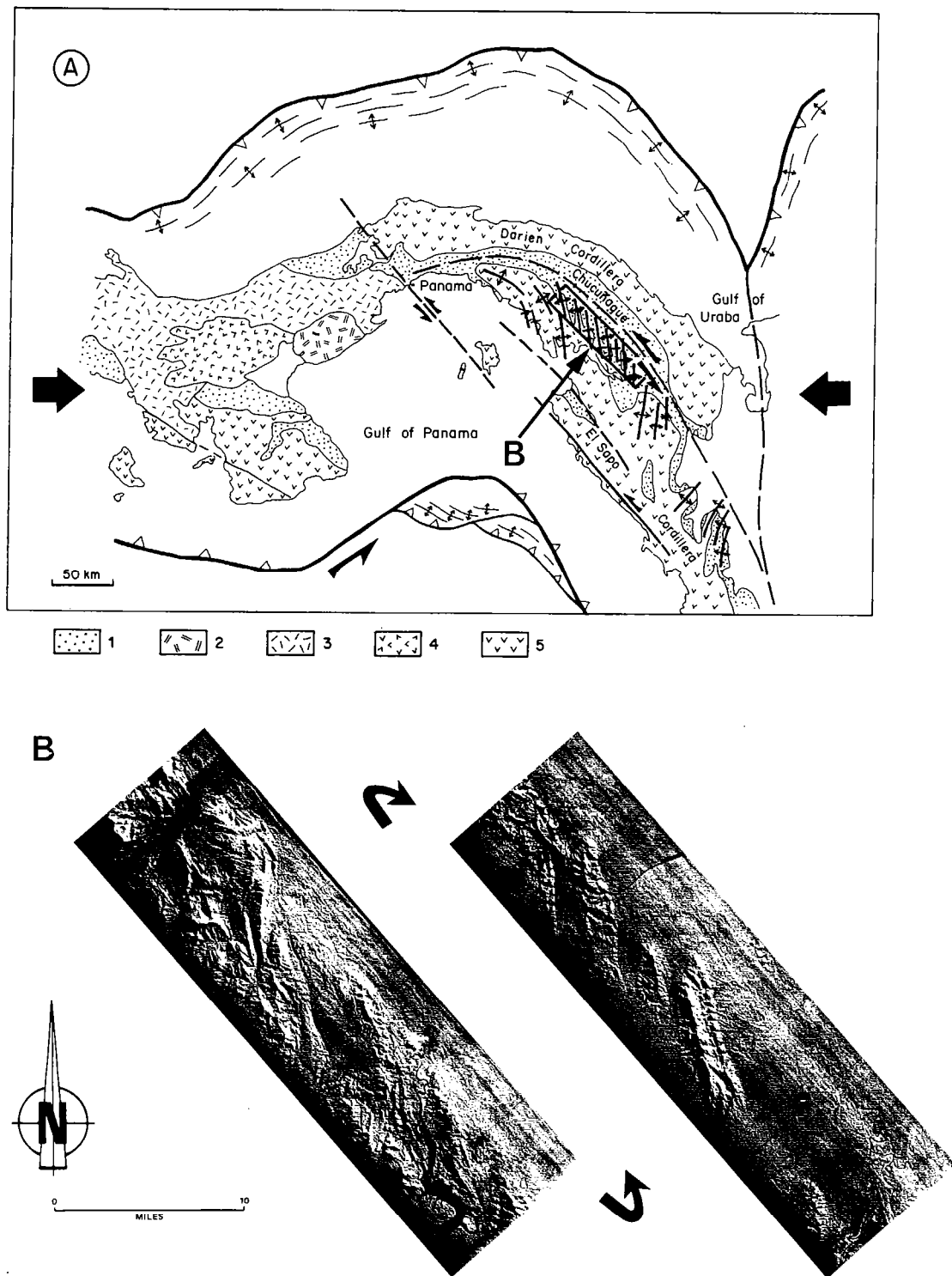
Fig. 1 - 10. Plis en échelon sur la marge ouest du domaine Caraïbes (d'après Stephan et al., 1986). (a) Dispositif structural du feston de Panama. (L) Image radar des plis en échelon de la bordure sud de la dépression de Chucunaque (voir (a) pour localisation) (d'après Wilcox et al., 1973).
