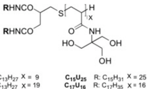
Figure 54. Structure chimique du C_nU_m cmc = 4,9-7,9 \mu M ;
