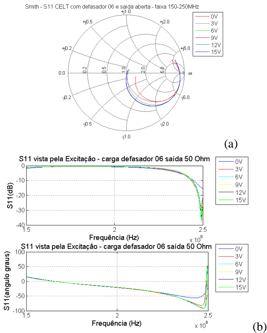
Figura 70 - Caracterização da câmara com defasador SO-06 na saída e carga 50 \Omega (150MHz-250MHz) (a) Carta de Smith (b) S11 Módulo e Ângulo.
