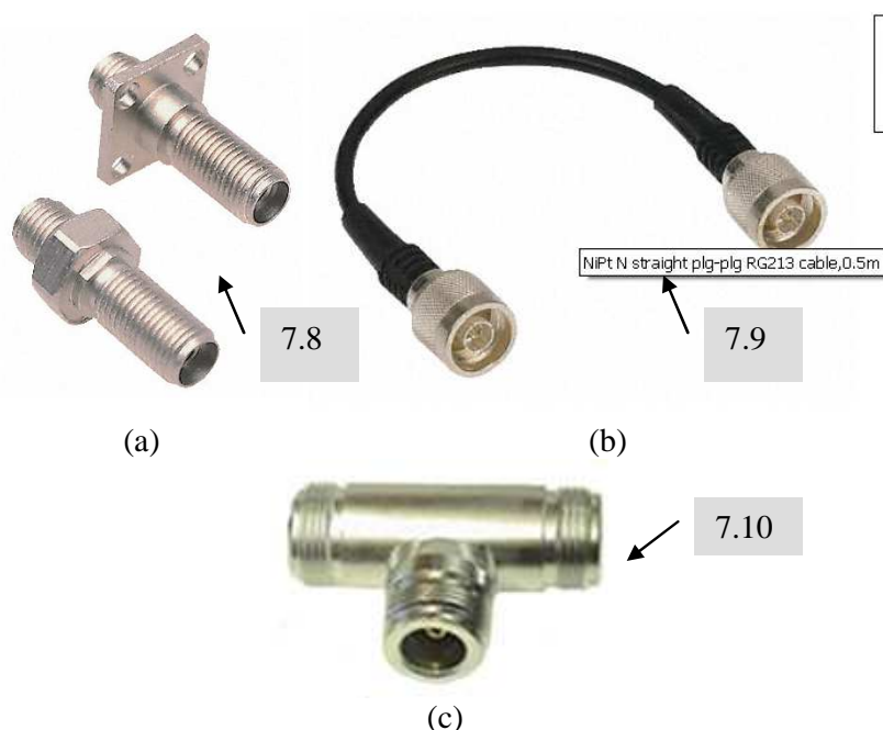
Figura 83 - (a) Conector de fibra óptica;; (b) Cabo de conexão tipo N –macho/macho; (c) Adaptador tipo N (3 x fêmea).
