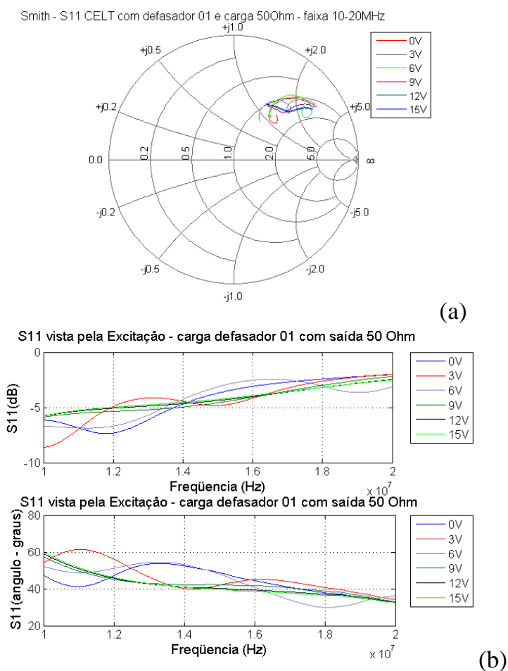
Figura 67 - Caracterização da câmara com defasador SO-01 na saída e carga 50Ω (10-20MHz) (a) Carta de Smith (b) S11 Módulo e Angulo
