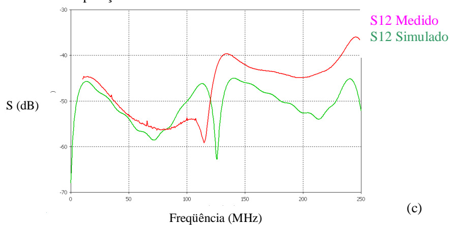
Figura 60 - Caracterização da câmara com carga 50 \Omega . Comparação dos valores em dB, medidos e simulados. (a) S11; (b) S13; (c) S12.
