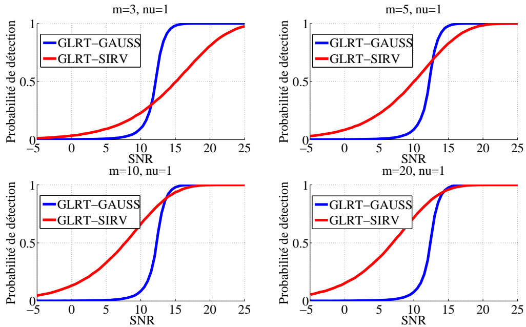
FIGURE 3.2 – Comparaison des performances du GLRT-GAUSS et du GLRT-SIRV dans un environnement non gaussien (Bruit K distribué \nu = 1 pour plusieurs dimensions)
