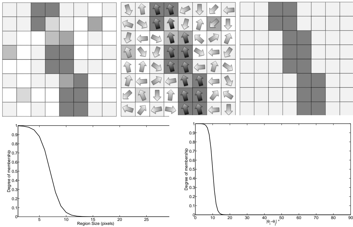
FIGURE 2.7 – Exemple d’application de la règle d’inference : à chaque pixel est attribué une orientation qui correspond à une structure plus globale qu’à l’échelle du pixel. En fonction des similitudes d’orientation et de contraste, les pixels puis les régions de petite taille sont fusionnés de façon privilégiée.
