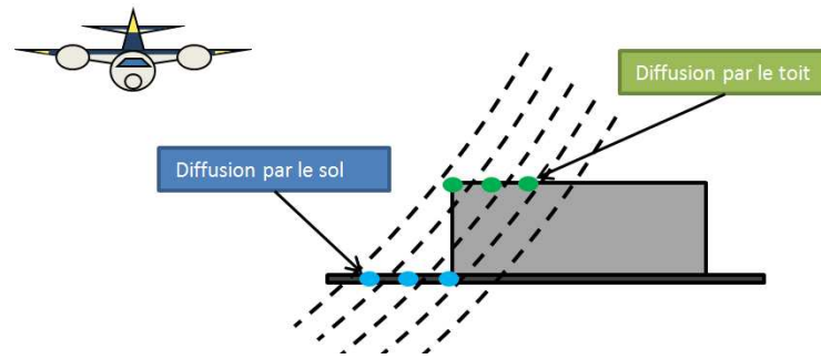
FIGURE 3.2 – Principe du layover en milieux urbains, exemple sur un bâtiment. Les lignes en pointillé représentent les lignes équidistantes à l’avion.
