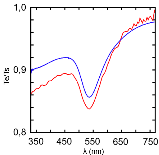
FIGURE V.10 – Mesures de spectrophotométries standard et résolue spatialement pour l'échantillon S05P09.
