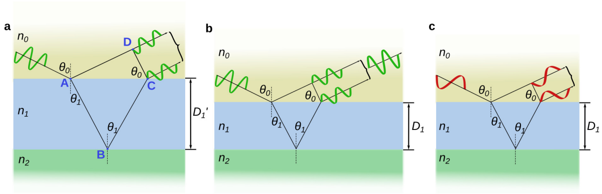
FIGURE II.12 – Représentations schématiques de l'interférence entre les ondes réfléchies par le 1^{er} et 2^{nd} dioptres. Pour une longueur d'onde donnée, le résultat de l'interférence dépend de l'épaisseur de la couche intermédiaire (épaisseur D dans la figure a et D' \neq D dans la figure b). Si l'on garde l'épaisseur de la couche intermédiaire constante, on constate que le résultat de l'interférence dépend de la longueur d'onde d'illumination (longueur d'onde \lambda dans la figure b, et \lambda' \neq \lambda dans la figure c).
