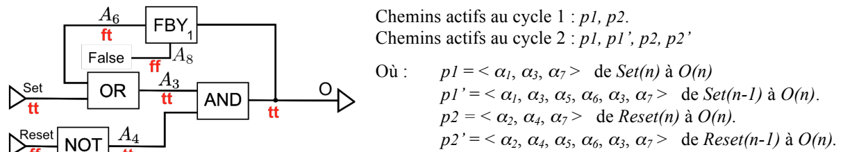
Figure II-g Chemins activés par l'exécution d'un scénario
