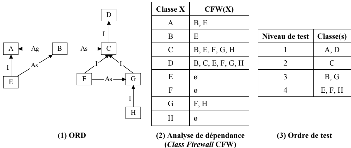
Figure I-c Ordre de test de Kung et al.
