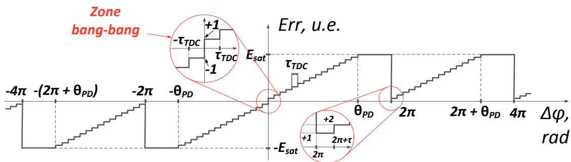
Figure 2.6: Réponse statique entrée-sortie du PFD
