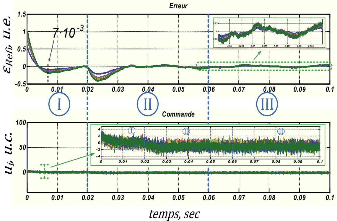
Figure 5.37: Simulations temporelles du réseau des Modèles de synthèse de l'ADPLL avec le bruit extérieur, l'évolution de l'erreur de suivi \varepsilon_{Ref_i} de toutes les ADPLLs (première sous-figure) et de commande de leurs correcteurs u_i (deuxième sous-figure) au cours du temps.
