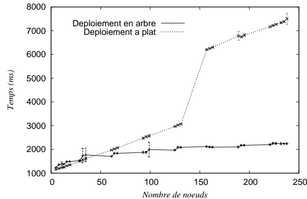
FIGURE 3.7 – Lancement d’une application effectuant des opérations de sorties (affichages) avec correspondance de l’arbre de routage des communications hors-bande selon l’arbre de déploiement de l’environnement d’exécution.
