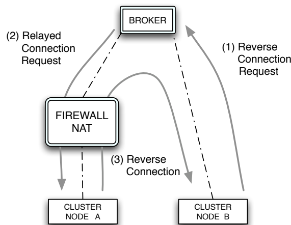
FIGURE 5.8 – Établissement d'une connexion inversée.
