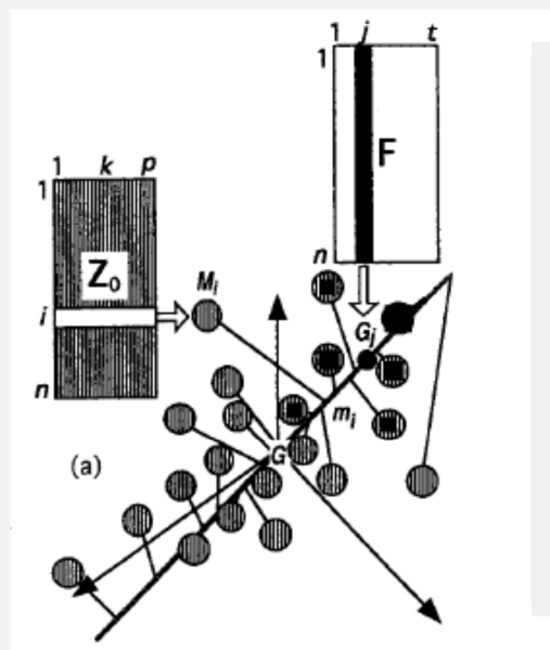
Figure B. Marginalité et tolérance dans l'OMI (Dolédec et al. , 2000). A partir de la matrice sites-habitat Z basée sur n sites et p variables, et de la matrice des profils d'espèces F (la matrice Y à t espèces, exprimée en proportions par colonne), on définit un espace multidimensionnel dont le centre de gravité est G (les conditions d'habitat les plus générales dans le jeu de données). Les cercles gris représentent les positions des sites; les carrés noirs celles de l'espèce j (la taille des carrés est proportionnelle à la fréquence de j ). La marginalité de j est définie par le décalage entre son centre de gravité G_j et G . La tolérance est une mesure de la variance inter-axes de cette marginalité.
