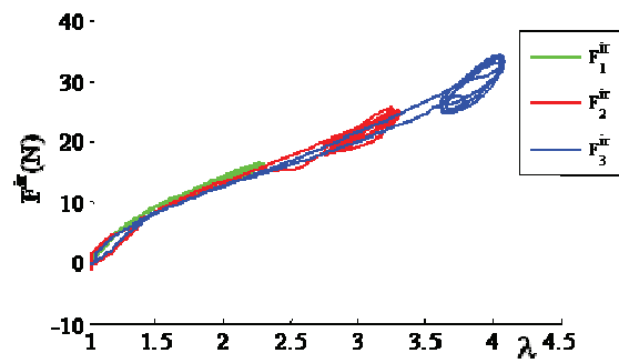
Figure 4-14 b : Réponses force-élongation
