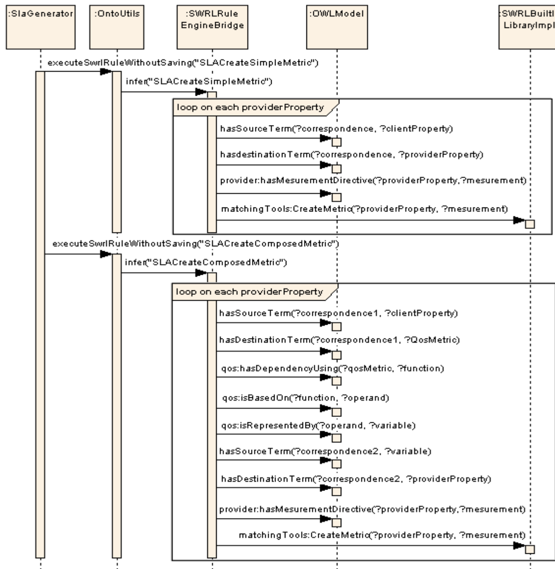
Figure 59 – Diagramme de séquence de l'étape de génération des métriques de QoS
