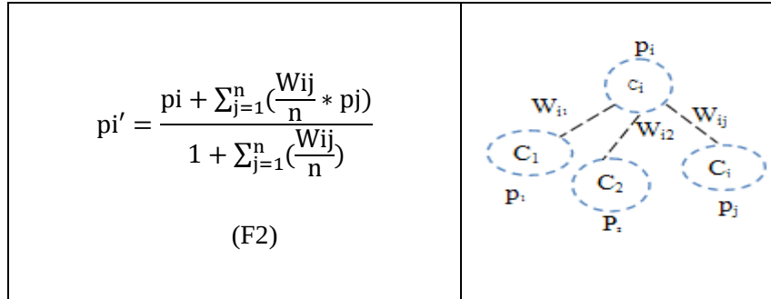
Figure 36 – Formule de propagation des probabilités des correspondances
