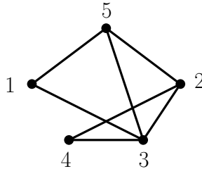
FIG. 2.1 – Exemple de graphe étiqueté à 5 sommets
