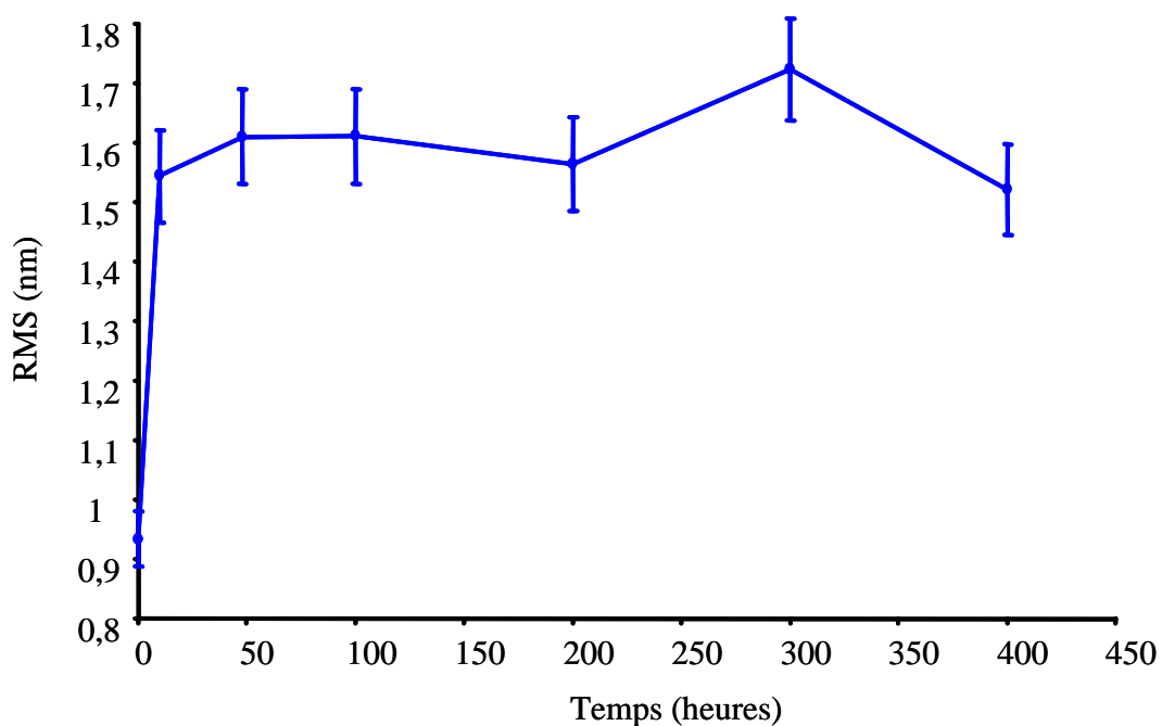
Figure 5- 4 : Evolution de la rugosité en fonction de la durée de chauffage sous vide à 60°C
