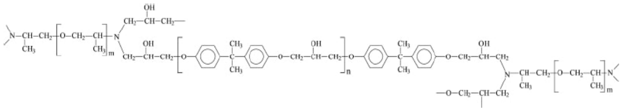
Schéma 3 : Structure de la résine époxy/amine
