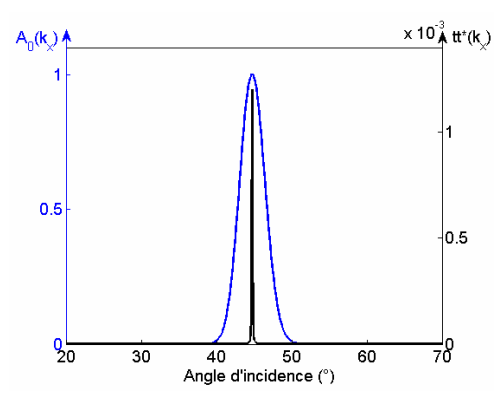
Figure VIII-15 a,b,c & d: Comparaison de la répartition d'ondes planes incidentes A_0(k_x) avec l'amplitude au carré du coefficient de transmission
