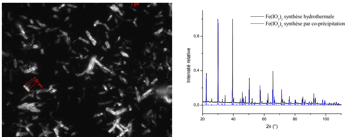
Figure I-7 : Microcristaux d'iodate de fer obtenus par synthèse hydrothermale.
