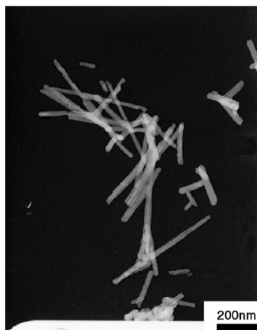
Figure I-5 : Image MET de nanocristaux de Fe(IO 3 ) 3
