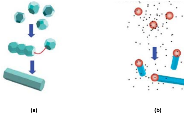
Figure I-26 : Représentations schématiques des mécanismes de croissance par (a) attachement orienté et (b) catalysés par des précurseurs cristallisés ; d'après P. D. Cozzoli 102
