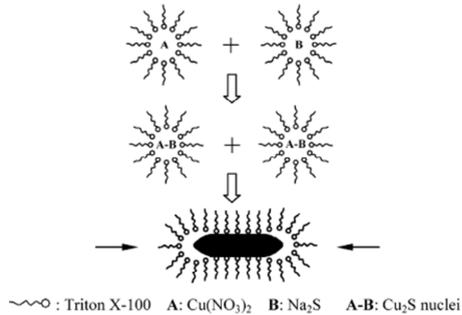
Figure I-27 : Représentation schématique du mécanisme de croissance par agrégation orientée pour des nanofils de \text{Cu}_2\text{S} dans le système (Triton X-100/cyclohexane/eau). Les flèches indiquent l'axe de croissance préférentiel ; d'après Y. Ding 110
