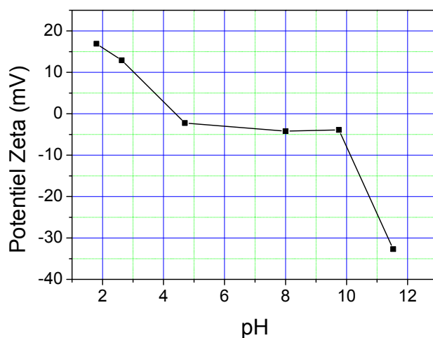
Figure IV-7 : Variation de potentiel zêta en fonction du pH pour les dispersions de nanobâtonnets cristallisés de Fe(IO 3 ) 3 dans NaCl à 0,001M
