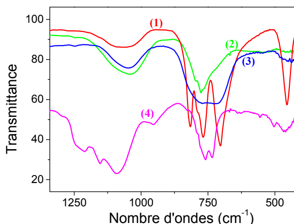
Figure IV-13 : Comparaison des spectres IR pour (1) des poudres cristallisées obtenues par voie hydrothermale (2) des poudres issues de ME amb en milieu acide (3) des nanoparticules primaires amorphes à partir d'une ME à base de Triton et (4) des poudres issues de ME A en milieu basique
