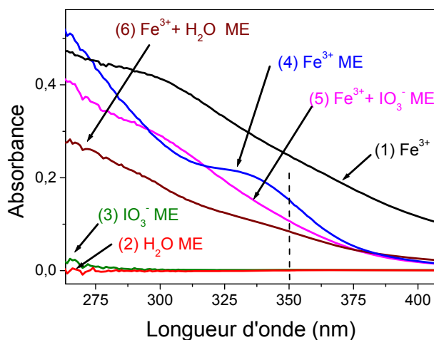
Figure II-6 : Spectres d'absorption UV-visible pour 1) une solution aqueuse de \text{Fe}^{3+} à 0,003M et pour (2-6) des solutions micellaires AOT/isoctane avec W=6 et [\text{AOT}] = 0,05\text{M} dans le cas 2) d'une solution micellaire d'eau pure, 3) d'une solution micellaire de \text{IO}_3^- à 0,1 M, 4) d'une solution micellaire de \text{Fe}^{3+} à 0,03 M, 5) à t=2 min après le mélange de solutions micellaires de \text{Fe}^{3+} à 0,03M et d' \text{IO}_3^- à 0,1M et 6) à t=2 min après le mélange d'une solution micellaire de \text{Fe}^{3+} à 0,03M et d'une autre contenant simplement de l'eau pure
