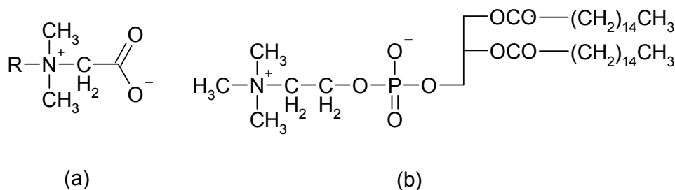
Figure I-14 : Schéma de molécules tensioactives amphotères : (a) un exemple de dérivé de la bétaïne et (b) la lécithine (dérivé de glycérophospholipide)
