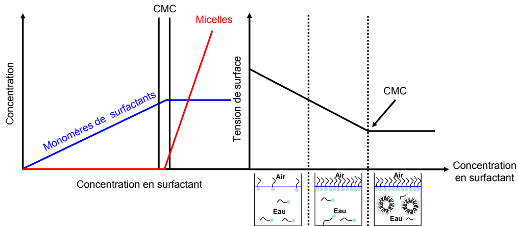
Figure I-16 : Schéma représentatif de la formation des micelles en fonction de la concentration en tensioactifs
