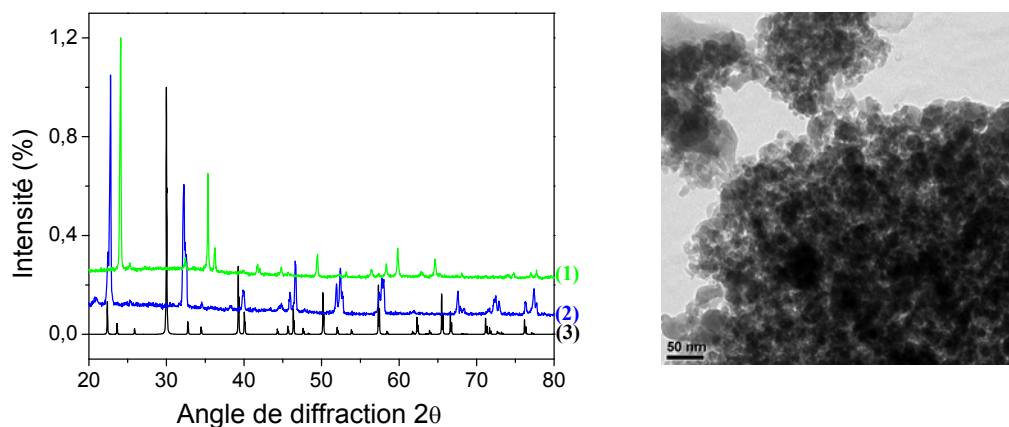
Figure IV-14 : Comparaison entre les diagrammes de diffraction des rayons X pour, (1) : Poudre obtenue de ME amb en milieu acide, (2) : Poudre obtenue de ME A en milieu basique, (3) : Le diagramme (ICSD#154674) de l'iodate de fer de référence. Image MET de la poudre obtenue de ME amb en milieu acide
