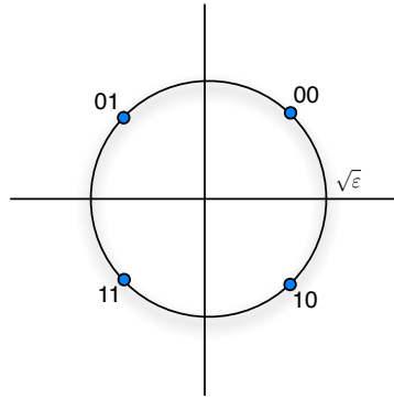
FIGURE 2.3 Constellation QPSK avec codage de Gray
