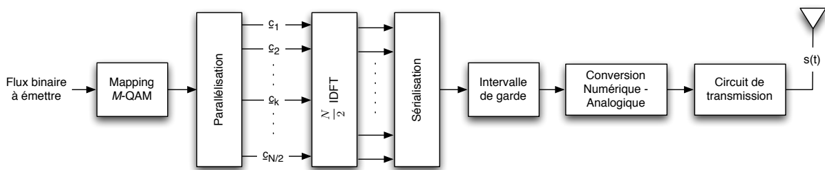
FIGURE 2.6 Émetteur OFDM classique
