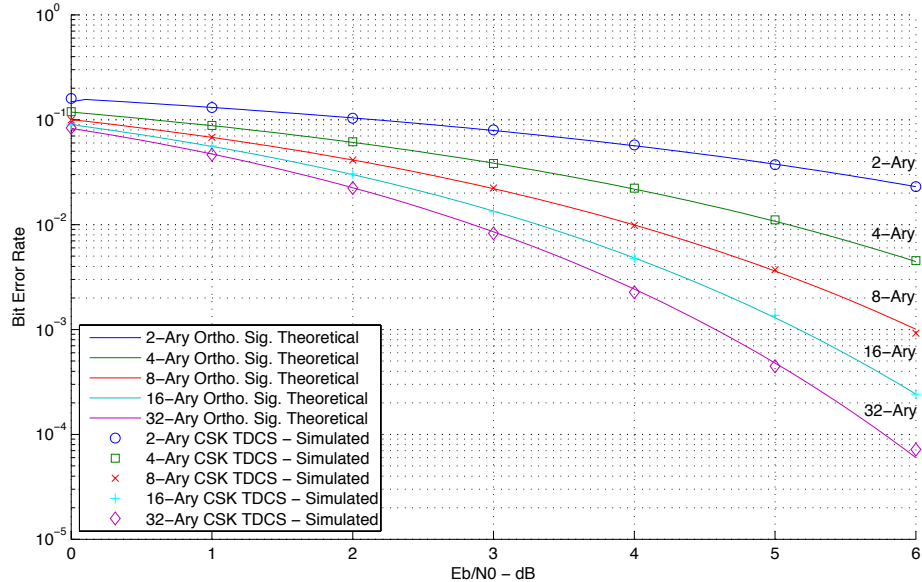
FIGURE 4.3 Taux d'erreur binaire d'un système TDCS - CSK
