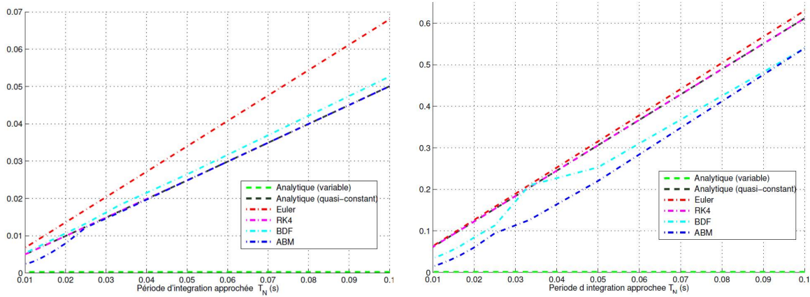
(a) Evolution de \|s - \hat{s}\| .
