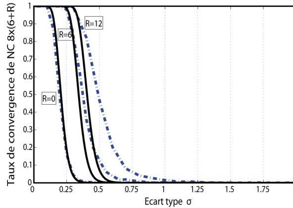
Figure III.15 : Probabilité de convergence de NC 8 \times (6+R) pour apprendre la fonction F=X_1 And X_2 . Les courbes discontinues représentent les résultats obtenus en simulation et les courbes discontinues représentent les résultats de calcul à partir du modèle de probabilité.
