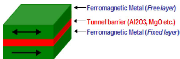
Figure I.19 : Jonction tunnel magnétique MTJ [WS09]
