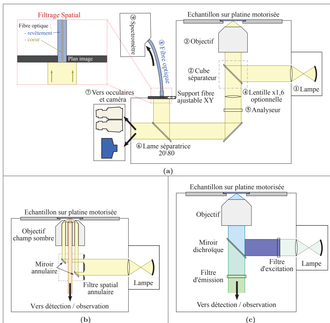
FIGURE 3.4 – (a) Schéma du montage de microspectroscopie. (b) Principe de fonctionnement du champ sombre en éclairage épiscopique. (c) Principe de fonctionnement de la microscopie de fluorescence.
