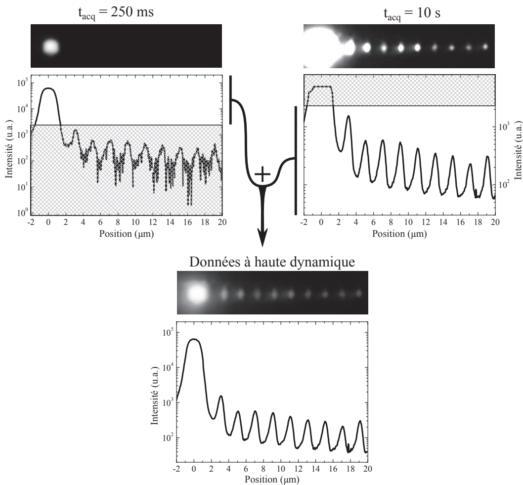
FIGURE 5.22 – Principe de l’algorithme HDR. Deux photographies de fluorescence acquises avec deux temps d’exposition différents sont combinées afin d’étendre la gamme d’intensité maximale de la caméra. Chaque graphe présent sous les photos correspond à une courbe de profil prise le long de la chaîne de microsphères. L’image HDR est en échelle logarithmique.
