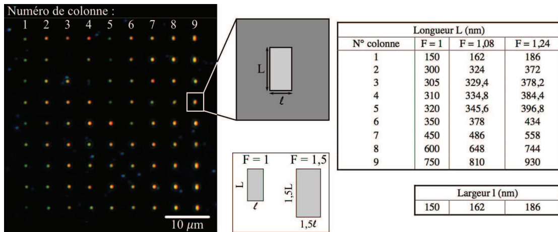
FIGURE 2.17 – Image en microscopie optique champ sombre d'un réseau de particules d'Or de 100 nm assemblées dans des boîtes de longueur L variable. Tableau des dimensions associées pour trois facteurs d'homothétie F.
