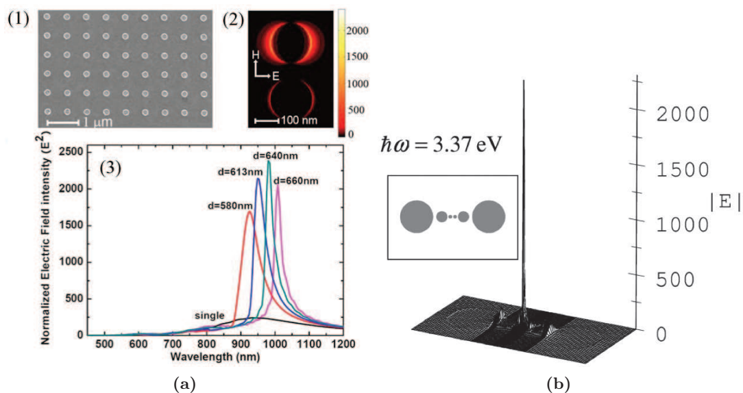
FIGURE 1.28 – (a) (1) Photographie MEB d'un réseau de plots d'Or de 180 nm, (2) Cartes de champ d'une nanoparticule dans un réseau (en haut) et toute seule (en bas) et (3) Intensité de champ E pour une particule unique et des réseaux de période d variable [Chu 2008]. (b) Exaltation géante du champ E par une nanolentille à base de sphère en Ag [Li 2003].
