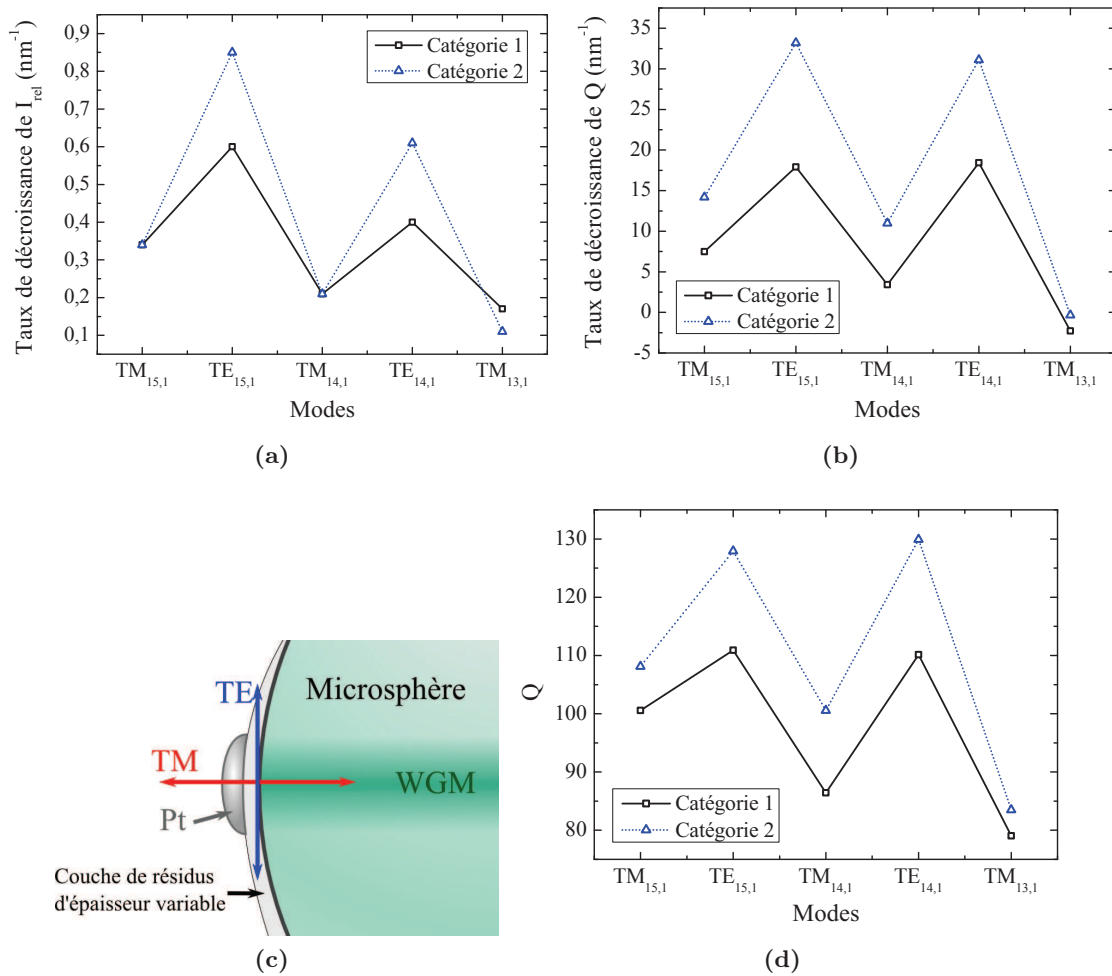
FIGURE 5.15 – Taux de décroissance de (a) I_{rel} et (b) Q en fonction de l'épaisseur de Pt déposée pour trois types d'objets : microsphères sans résidus (catégorie 1), microsphères partiellement (catégorie 2) et idéalement (catégorie 3) recouvertes de résidus. (c) Schéma montrant l'interaction selon la polarisation entre une nanopastille de Pt et un WGM d'une microsphère. (d) Facteur de qualité mesuré pour un dépôt de 0,2 nm de Pt, dans chaque configuration.
