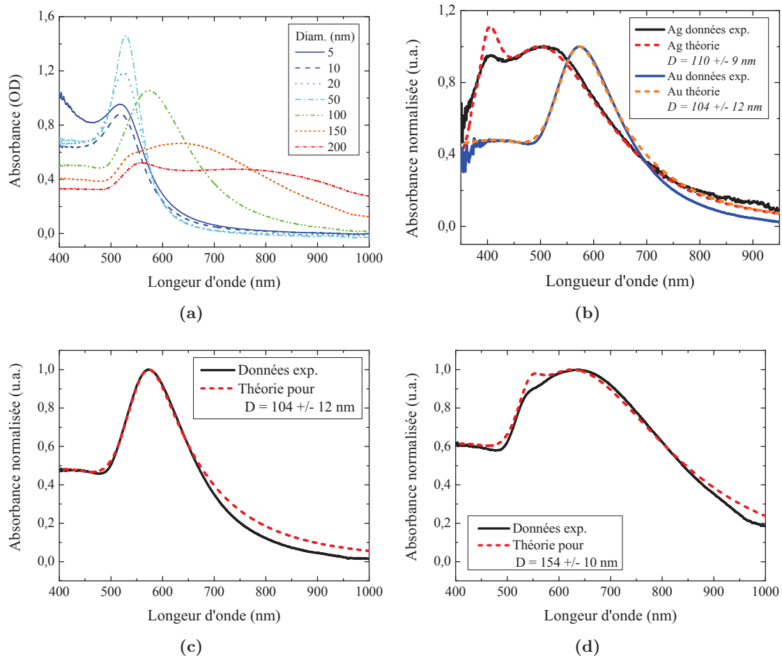
FIGURE 3.2 – Absorbance mesurée de suspensions colloïdales métalliques. (a) Particules d’Au de diamètre variable. (b) Comparaison entre deux suspensions colloïdales de nature différente et ajustement avec la théorie de Mie. (c) et (d) Réponse optique expérimentale et ajustement théorique des deux solutions d’Au sélectionnées pour la fabrication de superstructures.
