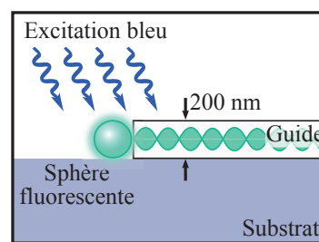
FIGURE 5.2 – Injection de lumière dans un guide à partir d'un émetteur local déposé à l'entrée du guide.
