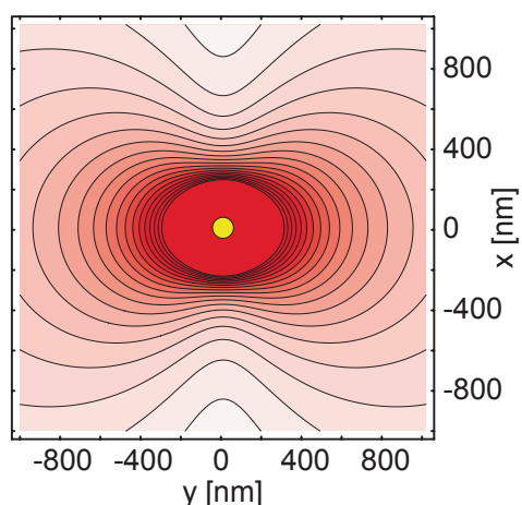
FIGURE 1.29 – Emission dipolaire par une nanoparticule : carte de champ lointain diffusé pour une illumination dans l'axe z et une polarisation en x [Hakanson 2008].
