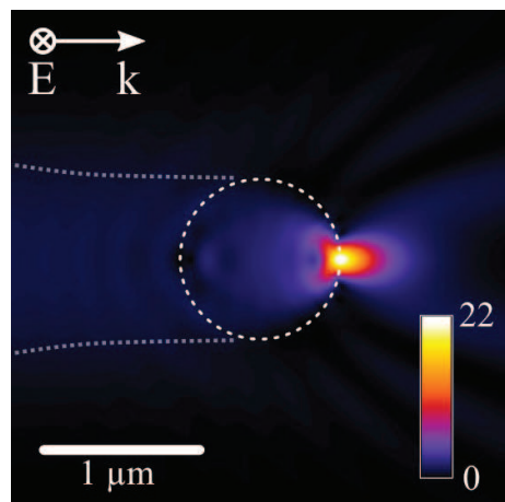
FIGURE 5.25 – Carte d'intensité du champ E d'une microsphère de \text{SiO}_2 de 1\ \mu\text{m} éclairé par un faisceau laser focalisé à \lambda = 405\ \text{nm} .
