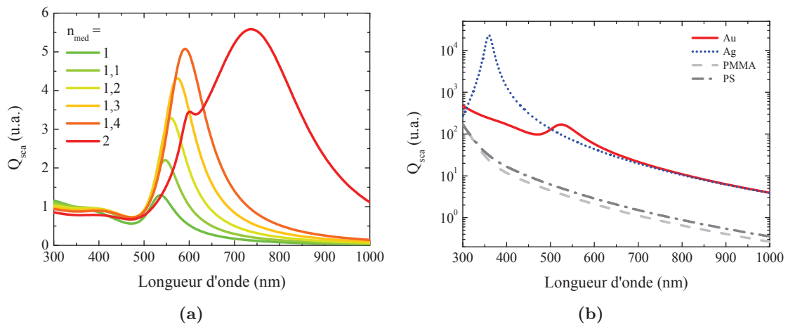
FIGURE 1.10 – Sections efficaces de diffusion : (a) particules d'Or de 100 nm dans milieu d'indice croissant et (b) comparaison de l'intensité de diffusion entre nanoparticules métalliques et diélectriques ( D = 50 nm).
