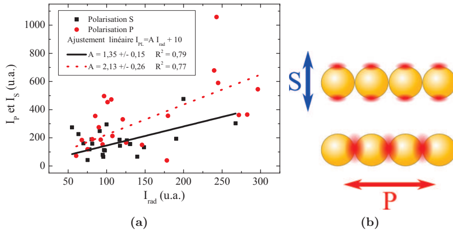
FIGURE 4.27 – (b) Schéma montrant la position des points chauds EM (halos rouge) dans une chaîne de billes d'Or pour 2 polarisations de la lumière.
