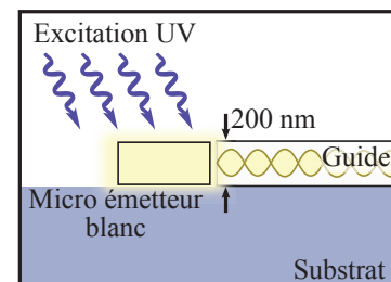
FIGURE 5.5 – Injection de lumière dans un guide à partir d’une microsource blanche de géométrie adaptée aux dimensions du guide.
