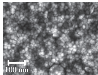
FIGURE 2.9 – Image MEB d'un dépôt d'ITO de 100 nm sur verre.
