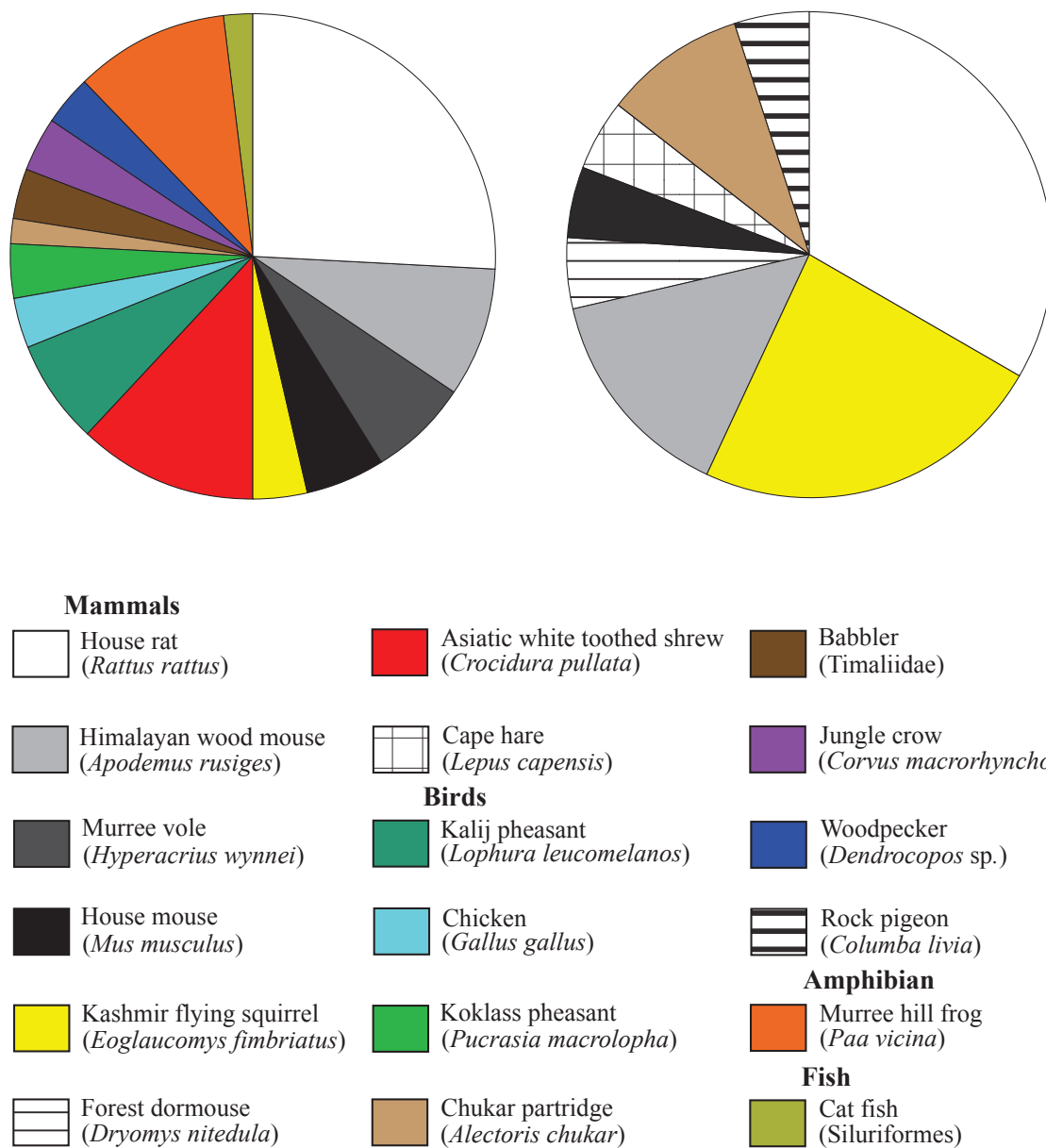
Fig. 1.2 Comparaison du régime alimentaire du chat léopard entre les Parcs Nationaux d'Ayubia et du Chitral Gol
