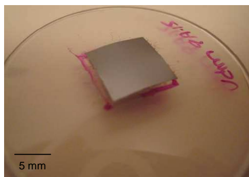
Figure B-24 : Courbure convexe d'un carré de silicium : 10 \times 10 \text{ mm}^2 épaisseur 25 \text{ }\mu\text{m}
