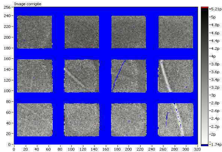
Figure C-36 : Caractérisation électrique de la matrice modifiée T – 480 \mu\text{m}
