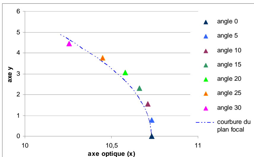
Figure A-16 : Graphe des coordonnées en mm des points de focalisation pour \phi / 2 = 1,5 mm
