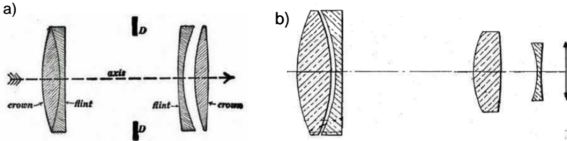
Figure A-20 : Objectif de Petzval : a) originel ; b) corrigé de l'aberration de courbure de champ
