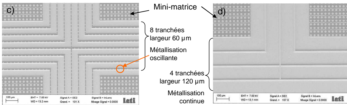
Figure C-23 : Variantes de métallisation des tranchées Photos : a) métallisation dentelle ; b) métallisation continue (1 tranchée) ; Clichés de microscopie électronique à balayage :
