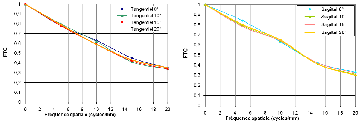
B : Système avec le détecteur courbé
