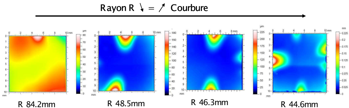
Figure B-37 : Surfaces des écarts à la sphère parfaite – Courbure convexe 10x10 mm 2 épaisseur 25 µ m Influence du rayon de courbure sur le nombre de pliures
