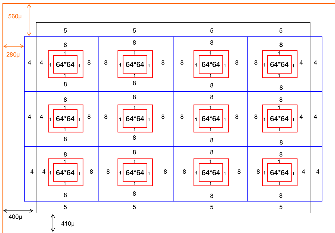
Figure C-20 : La matrice sensible modifiée et structurée en mini-matrice
