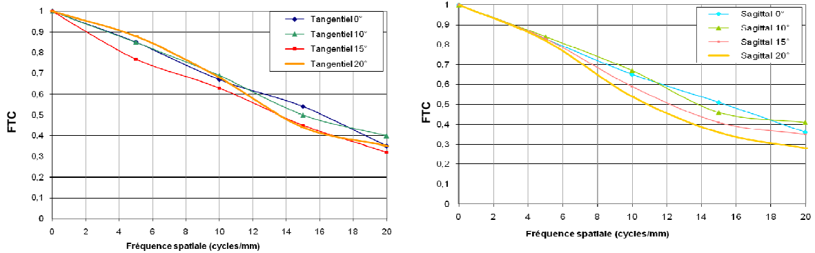
A : Système avec le détecteur plan
