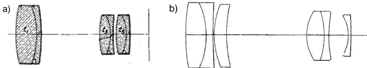
Figure A-21 : Lentilles de projection de Petzval avec a) deux doublets ; b) ménisque divergent
