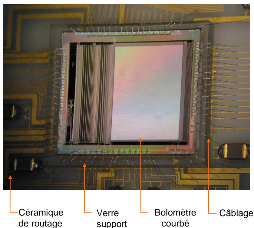
Figure C-51 : Bolomètre courbé
