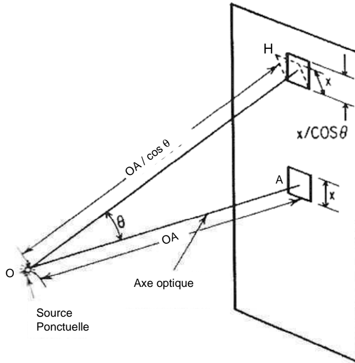
Figure A-27 : Eclairage sur un détecteur plan
