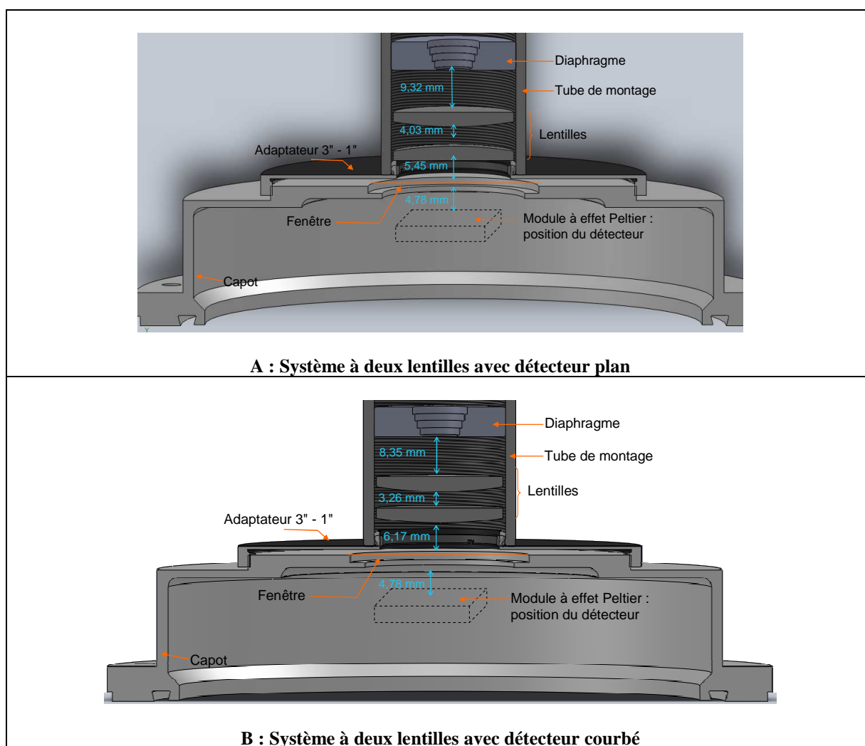
Figure D-28 : Plan des deux montages réalisés (issus de Solidworks)
