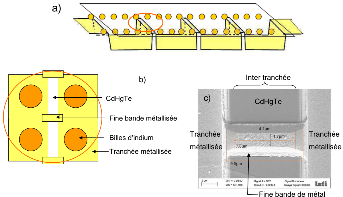
Figure C-24 : Métallisation des tranchées oscillantes a) schéma 3D des tranchées ; b) agrandissement au niveau des inter-tranchées ; c) photo au microscope électronique à balayage d'une fine bande sur une inter-tranchée
