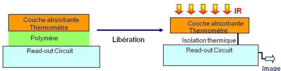
Figure C-39 : Fin du procédé de fabrication d'un bolomètre standard
