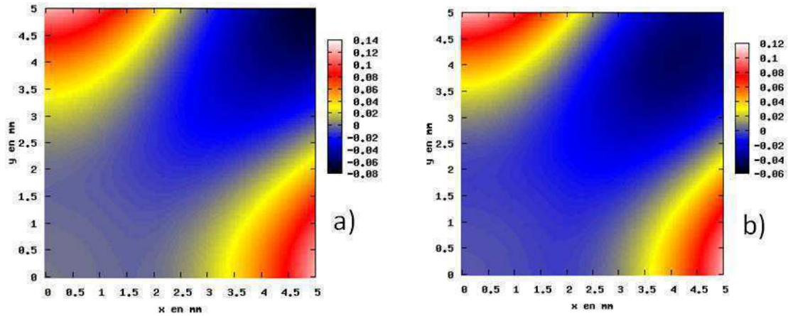
Figure B-58 : Comparaison des échantillons de 15 µm et 50 µm d'épaisseur courbés à un rayon de 45 mm a) Pression 8 kPa – 15 µm d'épaisseur ; b) Pression 50 kPa – 50 µm d'épaisseur
