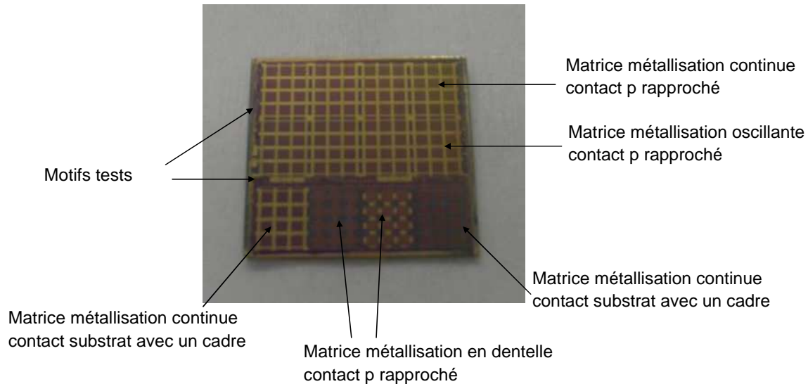
Figure C-33 : Plaqué fabriquée avec 12 variantes
