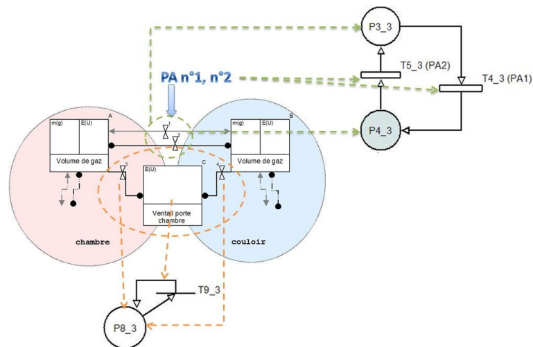
FIGURE 67 : PARALLÈLE ENTRE LE MODÈLE SYSTÉMIQUE ET LA PARTIE DE RÉSEAU REPRÉSENTANT LES INTERACTIONS CONTINUES DE L'OBJET AVEC LE MODÈLE AÉRAULIQUE
