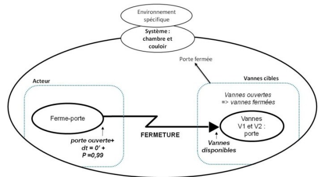
PA 2 : FERMETURE DE LA PORTE PAR LE FERME-PORTE
