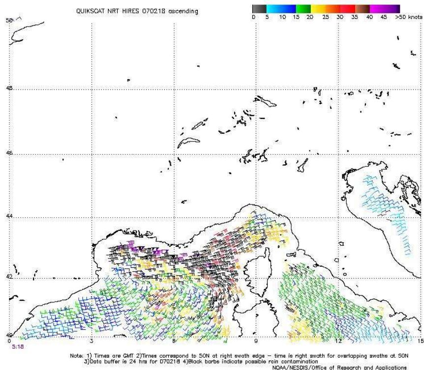
Fig. IV.39 – Mesure du vent par le satellite Quikscat le 18/02 à 5h18. Les mesures en noires sont des mesures incertaines.
