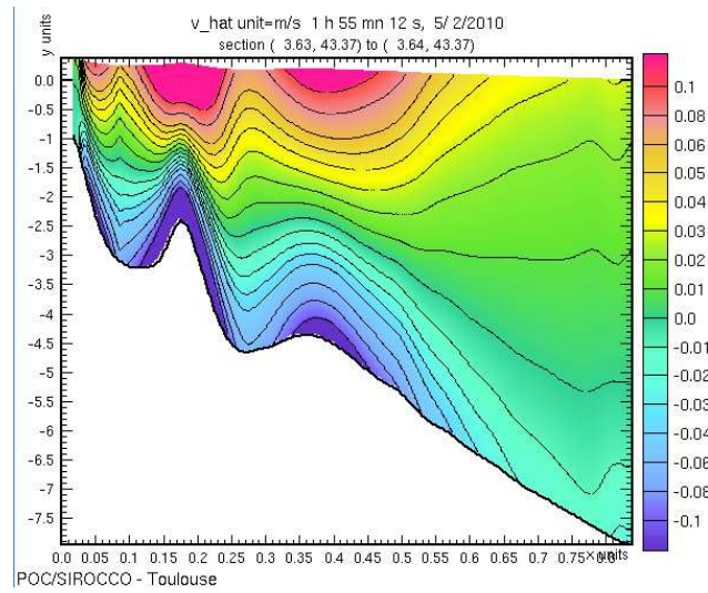
Fig. VI.26 – Coupe transversale de la vitesse cross-shore quasi-eulérienne (en \text{m}\cdot\text{s}^{-1} ) le long de la plage, le 5 février à 2h00 (moment où la dérive est maximale).
