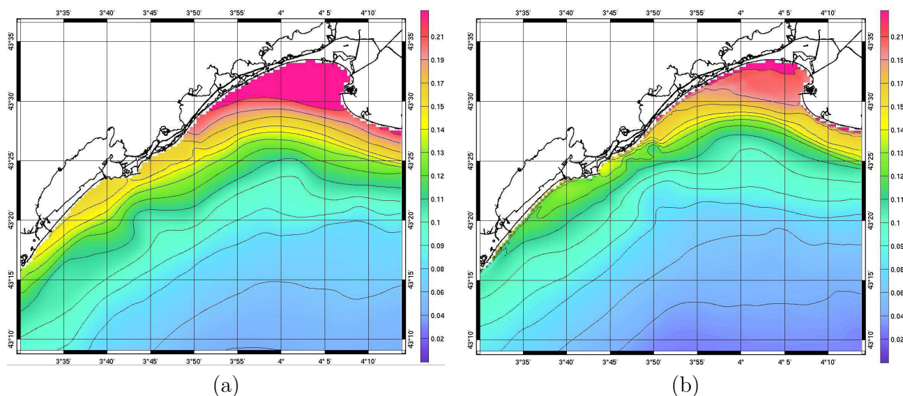
Fig. IV.24 – Élévation de la surface libre (en m) dans le GAM avec une simulation sans vague (a) et avec (b) pendant le second pic de la tempête, le 2 novembre 2008 à 15h
