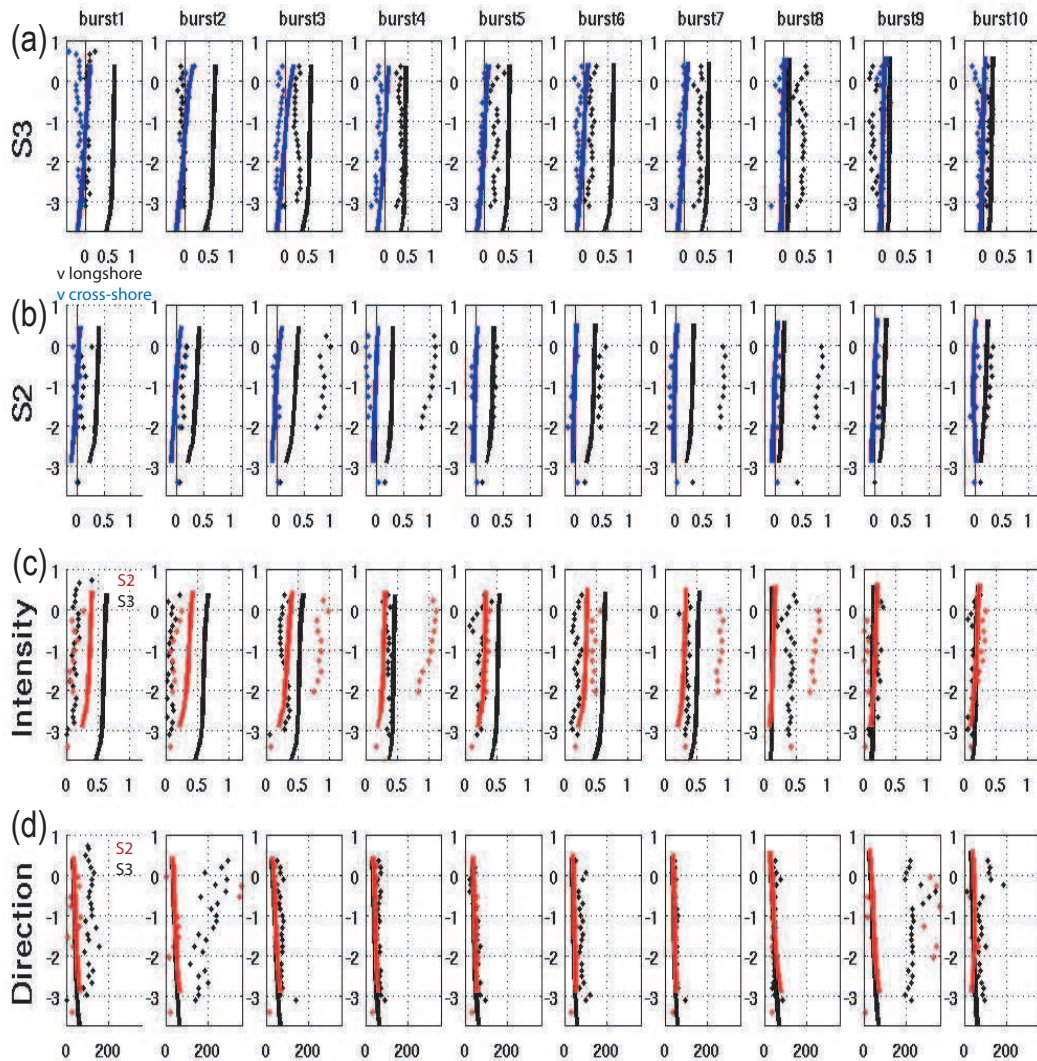
Fig. VI.23 – Courant simulé (traits continus) et observé (points) pendant le 2nd pic la tempête de février : profil des vitesses longshore (noir) et cross-shore (bleu) du courant en S3 (a), profil des vitesses longshore (noir) et cross-shore (bleu) du courant en S2 (b), intensité du courant en S3 et S2 (c) et direction du courant en S3 et S2 (d), par burst. La position des busts est précisée à la figure VI.6. Adapté de Robin [2011]
