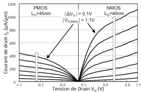
Figure II.31 : caractéristiques I_{\text{D}}(V_{\text{D}}) obtenues expérimentalement sur des transistors LSOI type-A. Les valeurs de courant sont normalisées par la largeur dessinée W_{\text{D}} = 110\text{nm} .
