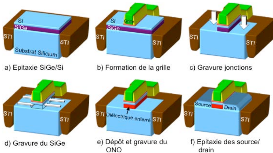
Figure II.14 : Schéma d'intégration d'un transistor LSOI type-A présentant principalement les étapes spécifiques à cette architecture.
