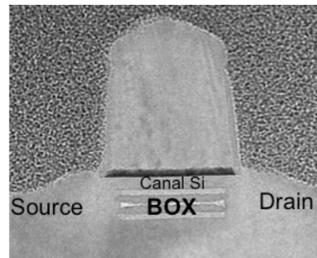
Figure II.17 : image en coupe TEM d'un transistor LSOI type-A après l'épithaxie des jonctions source/drain.
