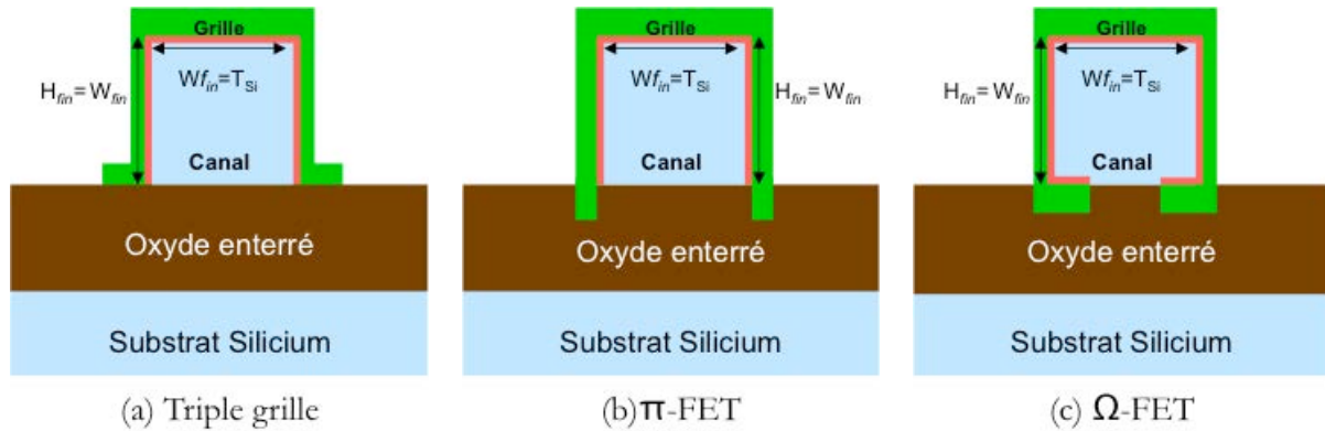
Figure I.21 : schéma d'une vue en coupe dans le sens de la largeur de transistors : a) triple grille, b) \pi -FET et c) \Omega -FET.
