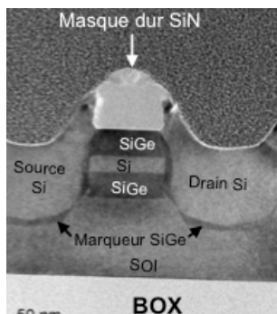
Figure IV.19 : Vue en coupe TEM d'un transistor GAA sur SOI après épitaxie des jonctions source/drain. Le marqueur SiGe avait été utilisé pour repérer la profondeur de la gravure jonction.
