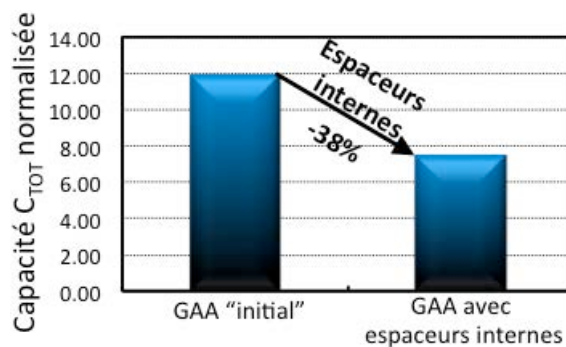
Figure IV.64 : Evaluation de la capacité totale C_{TOT} (normalisée par la capacité "utile" C_{GC} ) du GAA réalisé et du GAA intégrant des espaceurs internes.
