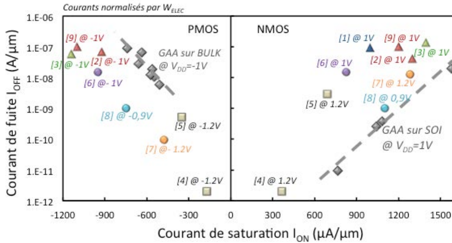
Figure IV.49 : compromis I_{ON}(I_{OFF}) comparant les différentes architectures à grilles multiples de la littérature récente. Toutes les valeurs de courant sont normalisées par la largeur effective W_{ELEC} et par le nombre de canaux le cas échéant ([4] et [5]).
