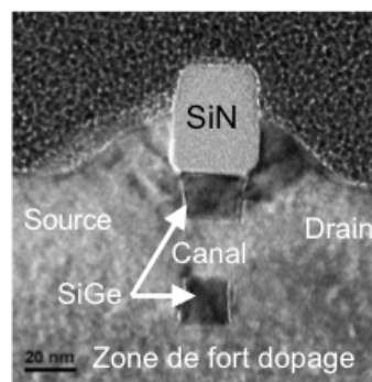
Figure IV.20 : Vue en coupe TEM d'un transistor GAA sur BULK après épitaxie des jonctions source/drain.
