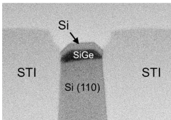
Figure III.6 : image en coupe TEM dans le sens de la largeur d'une épétaxie SiGe/Si enterrée sur substrat (110). On note la présence de facettes liée à la "non-optimisation" de l'abaissement du silicium par gravure HCl.
