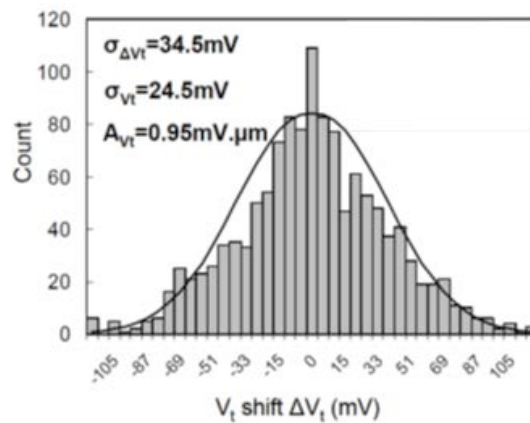
Figure II.6 : Distribution du décalage de la tension de seuil \Delta V_{TH} pour des transistors FDSOI courts et étroits ( L_G=25\text{nm} et W=60\text{nm} ). A_{V_{TH}}=0.95\text{mV}\cdot\mu\text{m} est une des plus petite variabilité présentées dans la littérature [Weber08].
