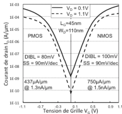
Figure II.30 : caractéristiques I_{\text{D}}(V_{\text{G}}) obtenues expérimentalement sur des transistors LSOI type-A. Les valeurs de courant sont normalisées par la largeur dessinée W_{\text{D}} = 110\text{nm} .
