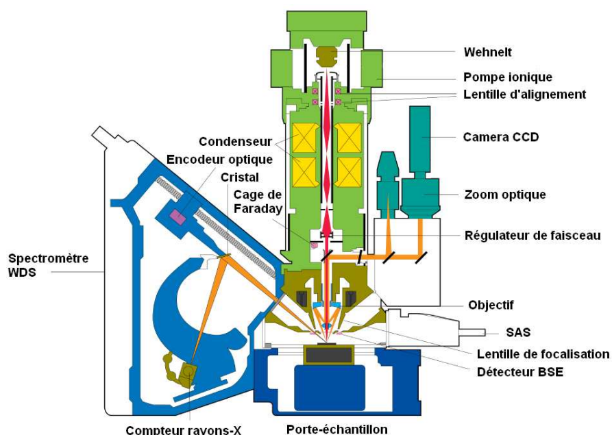
Figure II-14 : Schéma d'une microsonde électronique
