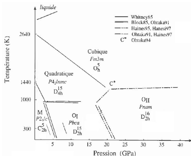
Figure I-16 : Diagramme pression température de la zircone pure (Bouvier 2000)
