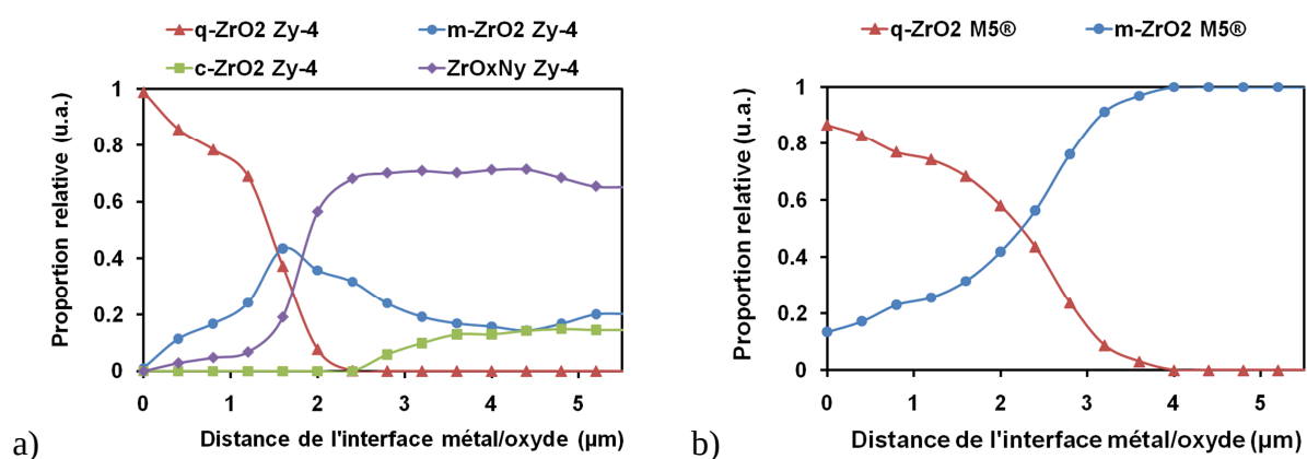
Figure VI-3 : Proportion relative de phases présentes dans les couches d'oxyde pré-transitoire d'épaisseur égale à 5.5 \mu\text{m} , formées à 800°C sur a) Zy-4 et b) M5®
