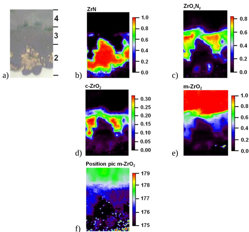
Figure IV-29 : a) Métallographie de l'interface métal/oxyde d'un oxyde post-transitoire formé à 800°C (surface évaluée 16 \times 24 \mu\text{m}^2 ). Images Raman à partir du signal de b) ZrN, c) \text{ZrO}_x\text{N}_y , d) c- \text{ZrO}_2 , e) m- \text{ZrO}_2 , et f) de la position du pic m_1 de la zircone monoclinique
