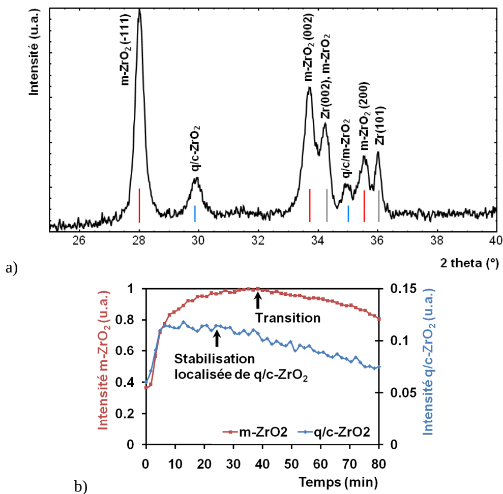
Figure VI-4 : a) Diagramme DRX acquis sur un échantillon de Zy-4 au moment de son oxydation sous air à 800°C, b) Variation de l'intensité des pics DRX de la zircon monoclinique ( m\text{-ZrO}_2 (-111)) et de la zircon quadratique et/ou cubique (q/c-ZrO 2 ) lors d'une oxydation de Zy-4 sous air à 800°C
