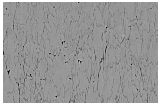
Figure IV-5 : Images MEB d'un oxyde post-transitoire formé sous air à 1000°C sur un échantillon en alliage de Zy-4 RXA. Révélation de a) la morphologie des grains en couche dense après fissuration, avec détails b) de petits grains en surface externe de la couche et c) de grains allongés dans l'épaisseur de l'oxyde
