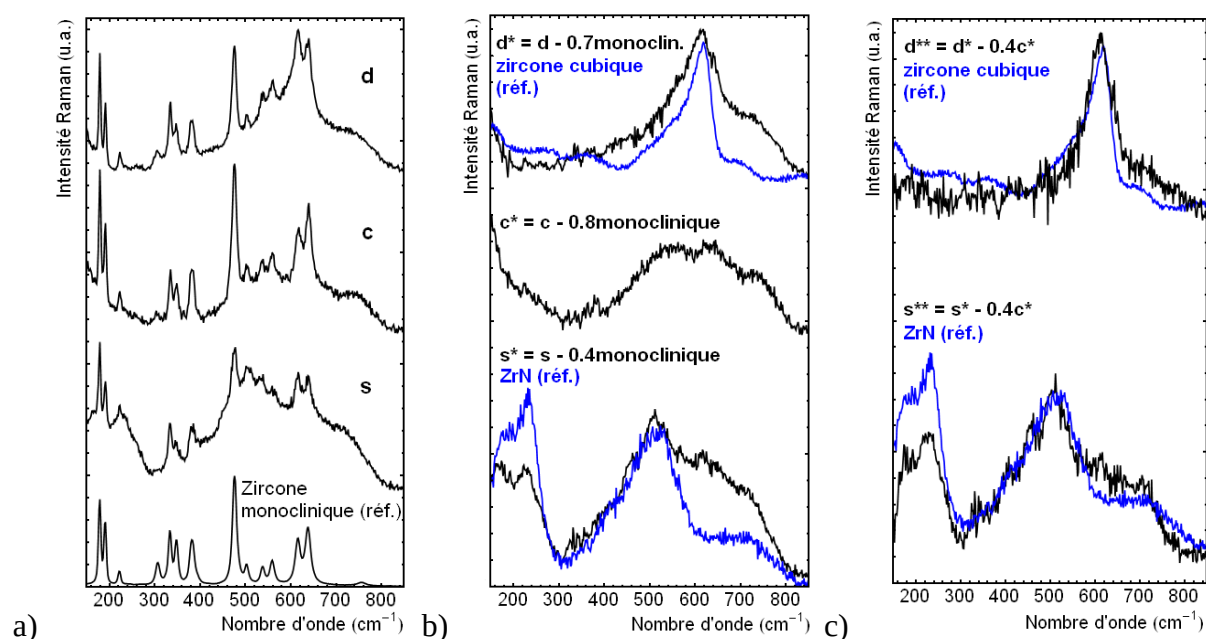
Figure IV-18 : a) spectres caractéristiques des phases s, c et d, b) résultantes s^* , c^* et d^* après soustraction de la composante de zircone monoclinique à chaque spectre, et c) résultantes s^{**} et d^{**} après soustraction de la résultante c^* à s^* et d^* , et comparaison avec les spectres de référence de la zircone cubique et du ZrN
