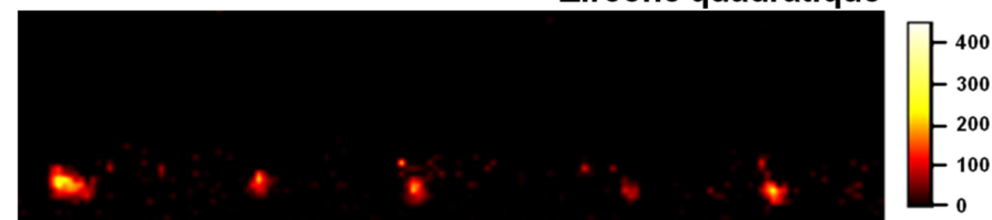
Zircone quadratique
