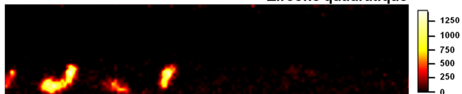
Zircone quadratique
