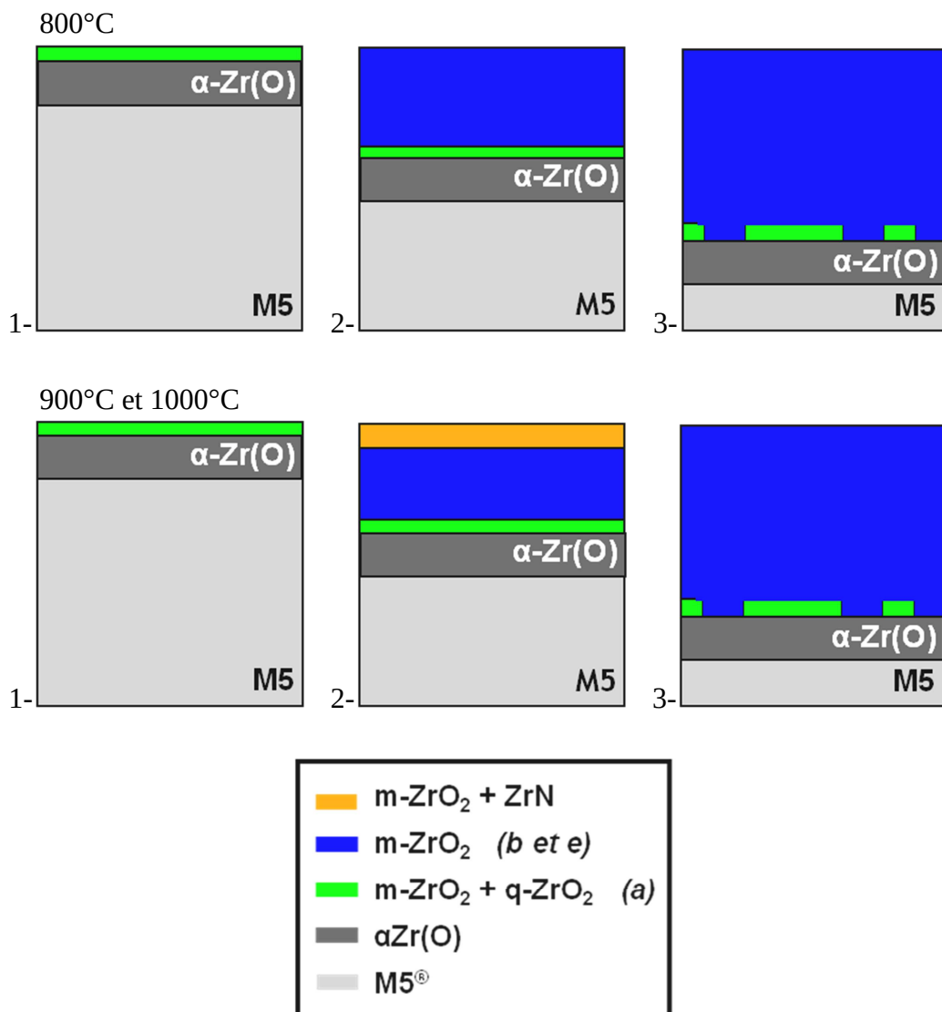
Figure VI-15 : Différentes étapes d'oxydation sous air du M5® en régime pré-transitoire
