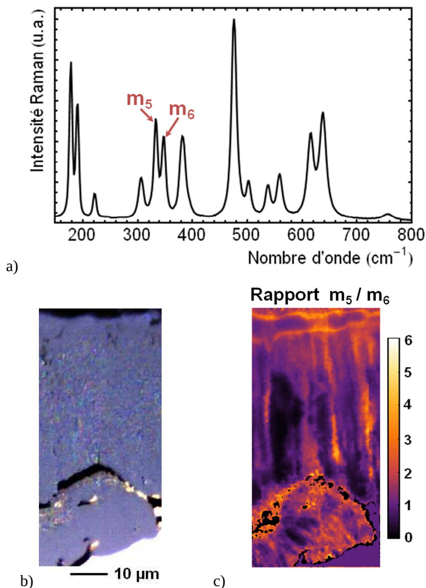
Figure IV-7 : a) Identification des pics m_5 et m_6 sur un spectre de zircone monoclinique, b) image optique d'une couche d'oxyde de Zy-4 SRA post-transitoire, formée à 1000°C, c) images Raman à partir du rapport d'intensité des deux pics monocliniques m_5/m_6
