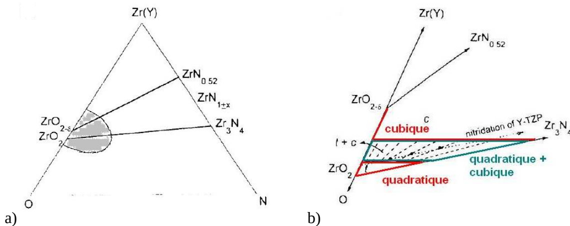
Figure I-20 : Représentation de a) la section isotherme à 1700°C du diagramme ternaire du système Zr(Y)-N-O, b) détails de la zone grisée en a) (Chung et al. 2001)
