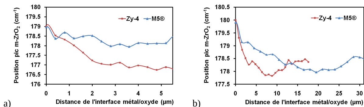
Figure VI-2 : Evolution de la position du pic de monoclinique m_1 sur des couches d'oxyde pré-transitoire formées à 800°C sur du Zy-4 et du M5®, d'épaisseurs a) 5.5 \mu\text{m} , et b) critique avant fissuration
