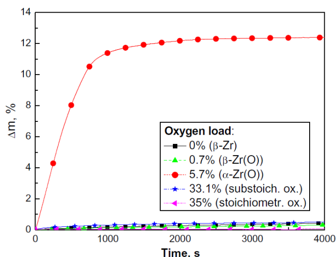
Figure I-12 : Prise de masse des échantillons de Zy-4 pré-oxydés et homogénéisés, puis recuits sous azote à 1200°C (Steinbrück 2009; Duriez et al. 2009)
