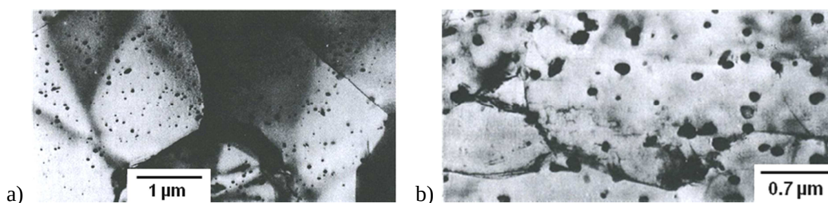
Figure I-5 : Microstructure et distribution des a) précipités \beta -Nb dans l'alliage Zr-1%Nb recristallisé, et b) des précipitées Zr(Nb,Fe)_2 dans l'alliage Zr-1Nb-1.3Sn-0.4Fe (Cox et al. 1998)
