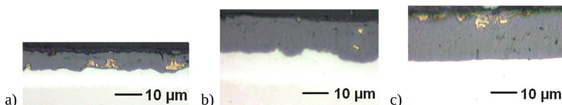
Figure IV-14 : Métallographies des couches d'oxyde pré-transitoires avec particules de ZrN, formées à des températures d'oxydation de a) 800°C, b) 900°C et c) 1000°C
