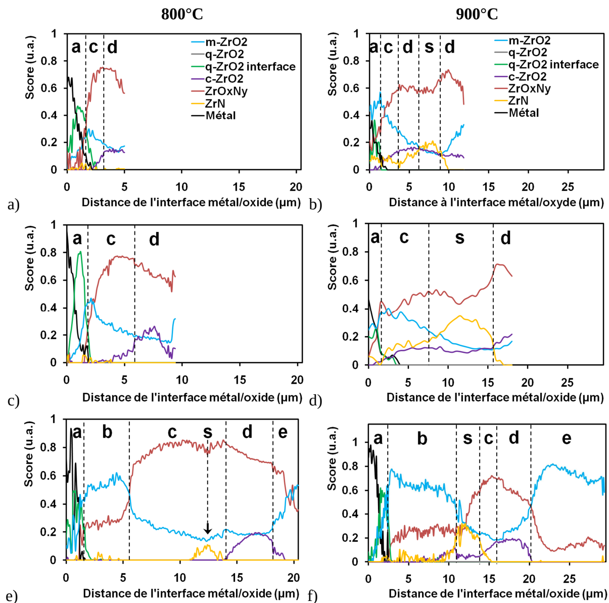
Figure IV-23 : Profils de présence des phases élémentaires pour les couches d'oxyde de Zy-4 RXA formées à 800°C d'épaisseur de a) 5 \mu\text{m} , c) 9 \mu\text{m} et e) 20 \mu\text{m} , et à 900°C dont l'épaisseur est de b) 12 \mu\text{m} , d) 18 \mu\text{m} et f) 29 \mu\text{m}
