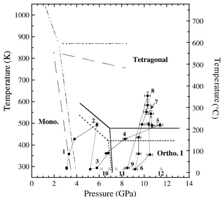
Figure I-17 : Diagramme de phase P-T de la zircon à P isostatique. Les domaines d'existence déterminés sur des zircons issues de l'oxydation d'alliages M5 ® et Zy-4 sont respectivement représentés par des traits pleins et des traits en pointillés. Les traits segmentés correspondent aux résultats de Block (Block et al. 1985). Chaque point noir correspond à une mesure réalisée sur un spectre Raman acquis sur des zircons produites par oxydation d'alliages de Zr pour un couple P-T déterminé. Les triangles correspondent à une référence de zircon monoclinique (Bouvier 2000)
