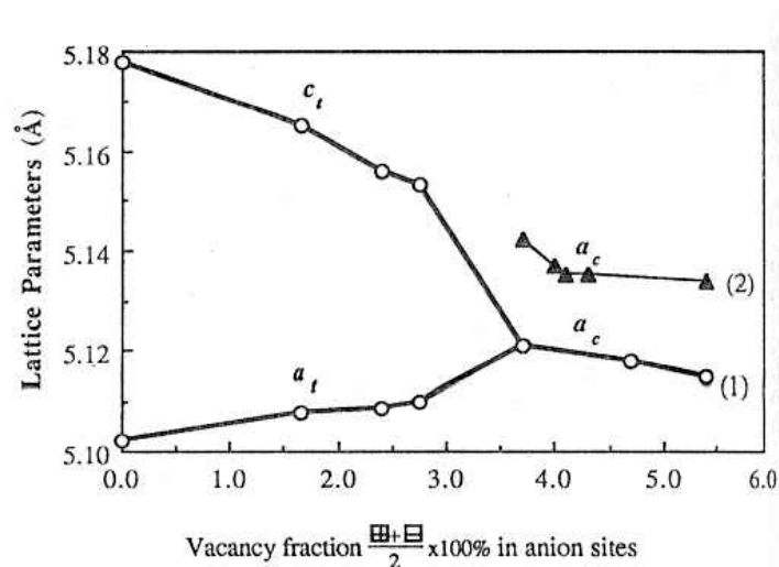
Figure I-22 : Variation de paramètres de maille de la zircone en fonction du pourcentage de lacunes anioniques pour (1) (3Y)ZrO_2 + N_2 , et (2) (8Y)ZrO_2 + N_2 (Cheng & Thompson 1993)
