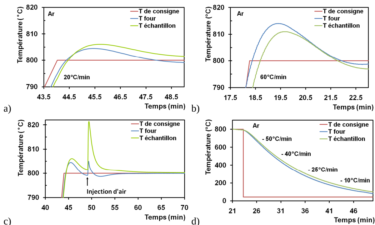
Figure II-4 : Températures de consigne, du four et de l'échantillon relevées par les thermocouples au cours a) d'une transition chauffage à 20°C.min -1 - palier isotherme à 800°C, b) d'une transition chauffage à 60°C.min -1 /palier isotherme à 800°C, c) d'un changement d'atmosphère Ar/air lors d'un palier isotherme à 800°C, et d) d'un refroidissement continu
