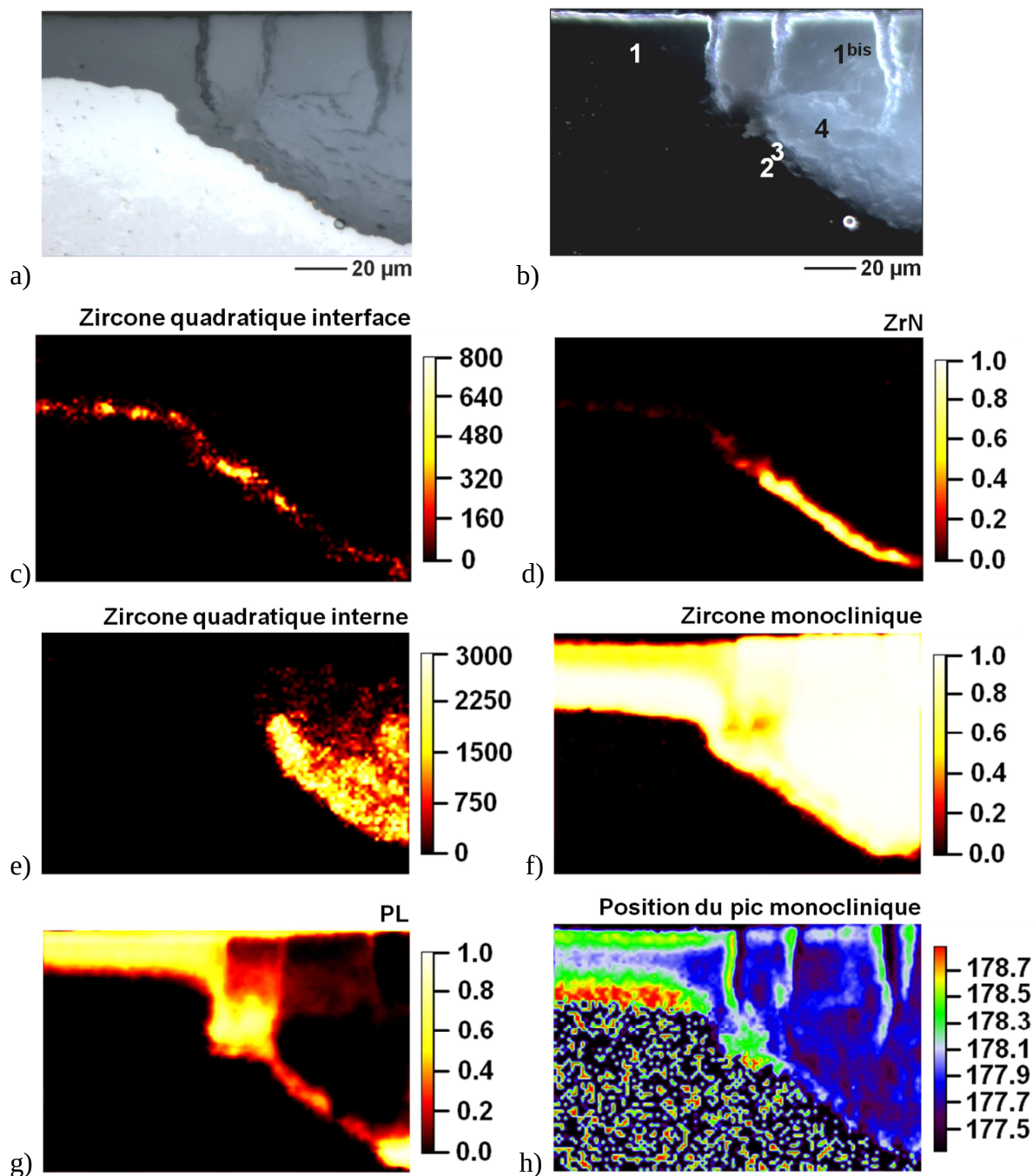
Figure V-10 : Images optiques en a) champ clair, et b) champ sombre d'une couche d'oxyde de M5 ® post-transitoire formée à 800°C. Images Raman à partir c) de la phase de zircon quadratique à l'interface métal/oxyde, d) du ZrN, e) de la phase de zircon quadratique en couche interne, f) de la phase de zircon monoclinique, g) du fond PL, et h) de la position du pic de monoclinique m_1
