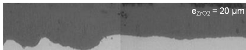
Zircone quadratique
