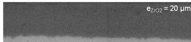
Zircone quadratique
