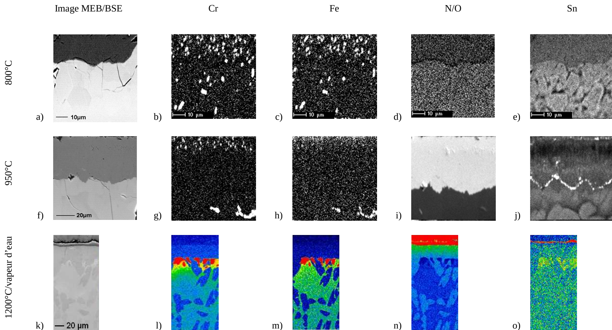
Figure IV-9 : Images BSE d'oxydes formés sur a) Zy-4 SRA sous air à 800°C, f) Zy-4 RXA sous air à 950°C et k) Zy-4 SRA sous vapeur d'eau à 1200°C. Cartographies EPMA respectives de b-g-l) Cr, c-h-m) Fe, d) N, i-n) O, et e-j-o) Sn
